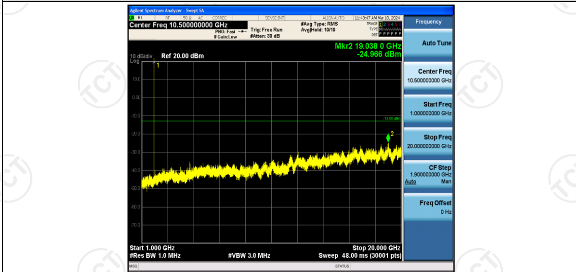
Band2-5MHz-16QAM-19175-1RB#0-Range2:1000~20000MHz
