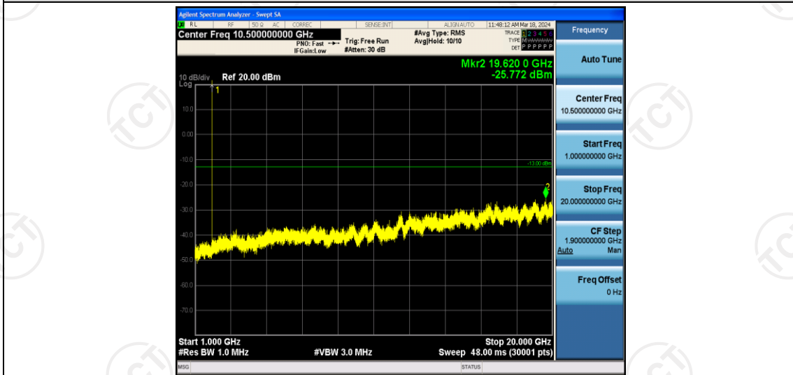
Band2-5MHz-QPSK-19175-1RB#0-Range2:1000~20000MHz
