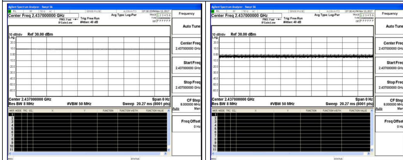
IEEE 802.11b
