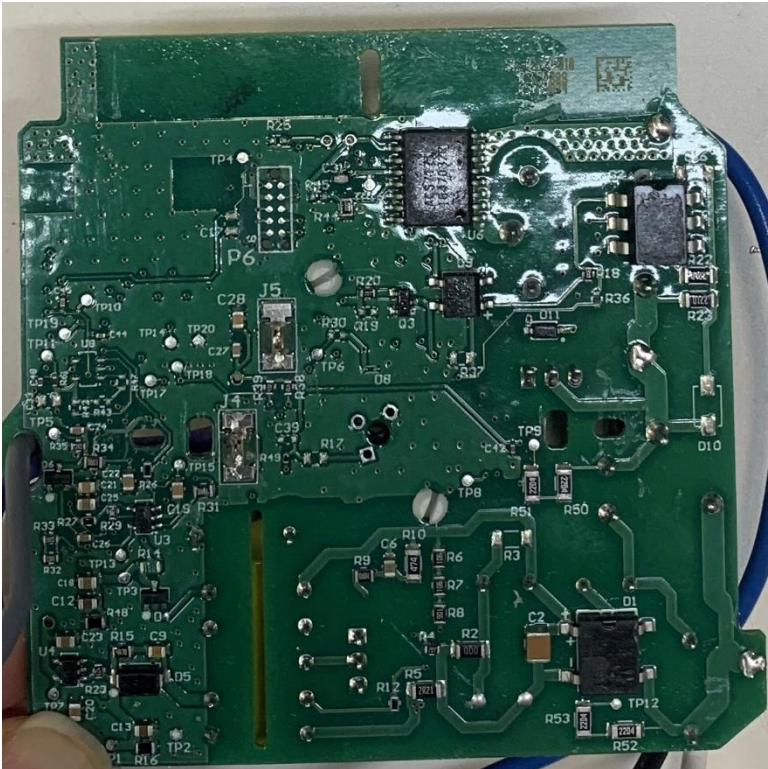
PCBA ( Bottom)
