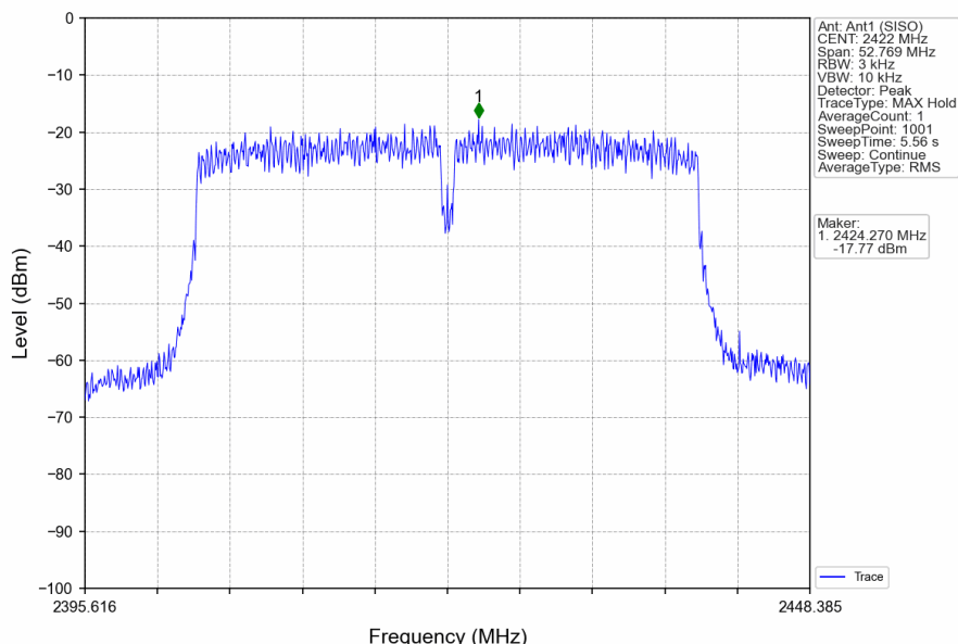
802.11n(HT40)_LCH_2422MHz_Ant1 (SISO)_NTNV
