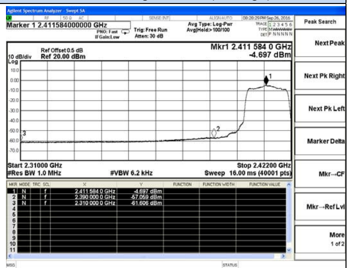
802.11g-Low channel(Average)
