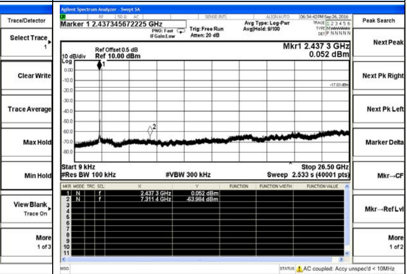
IEEE 802.11b-Middle channel
