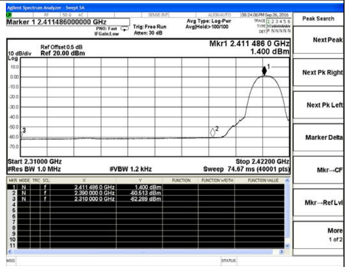
802.11b-Low channel(Average)
