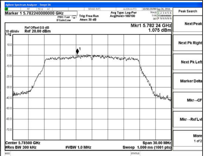
802.11ac20-5785MHz
