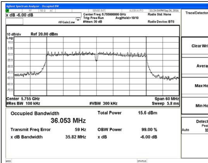
802.11n-HT40-5755MHz
