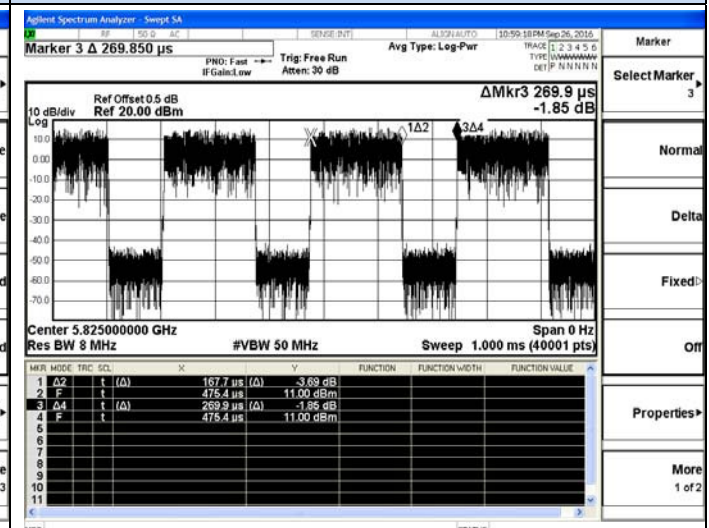
802.11ac20
