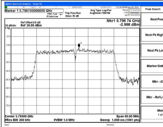
802.11n-HT40-5795MHz
