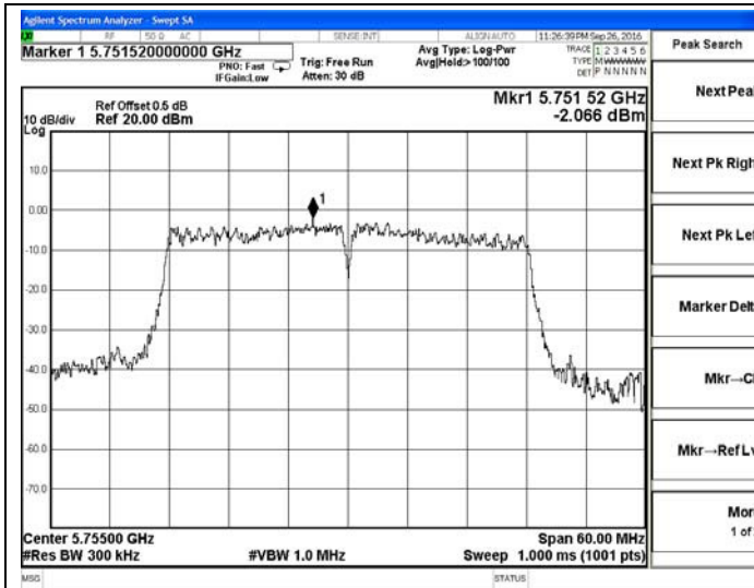
802.11n-HT40-5755MHz
