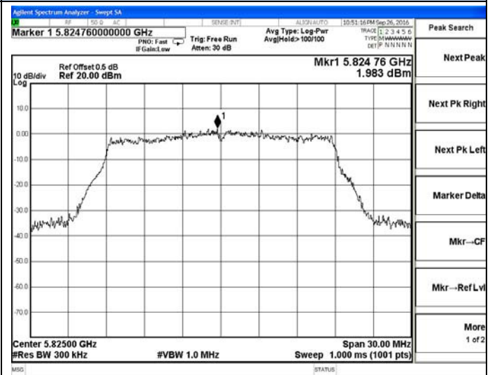
802.11ac20-5825MHz
