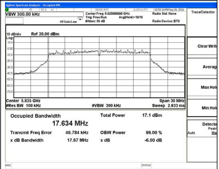
802.11ac20-5825MHz
