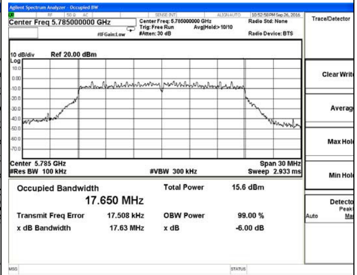
802.11ac20-5785MHz
