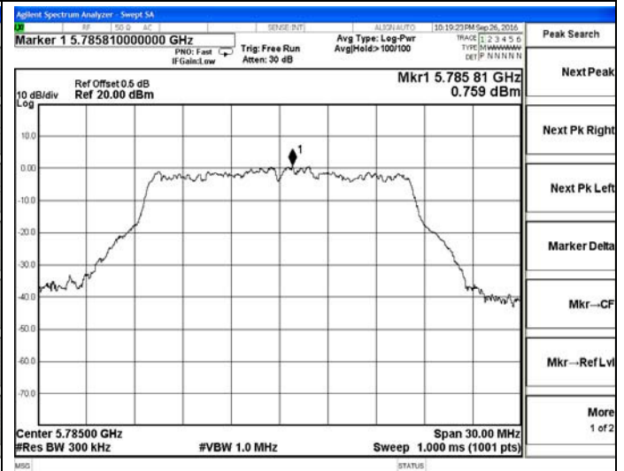
802.11n-HT20-5785MHz
