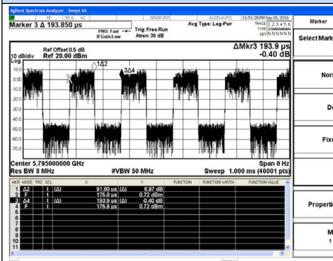
802.11ac40
