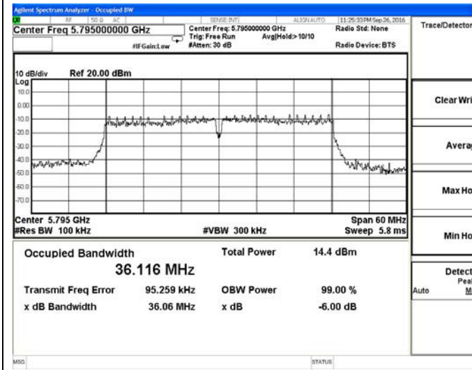
802.11n-HT40-5795MHz
