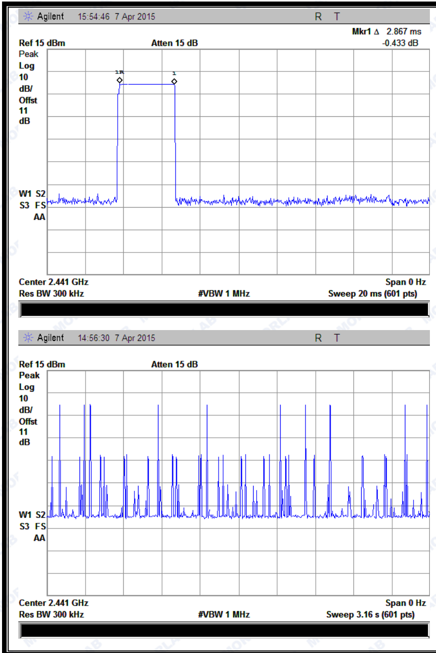
(Plot F: DH5 @ \pi/4 -DQPSK)
