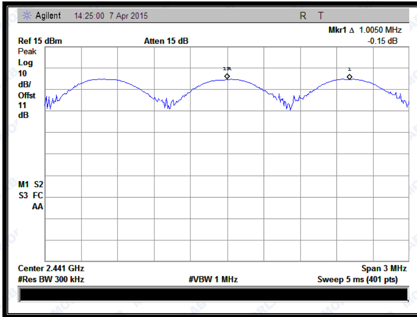
(Plot B: 1/4-DQPSK)
