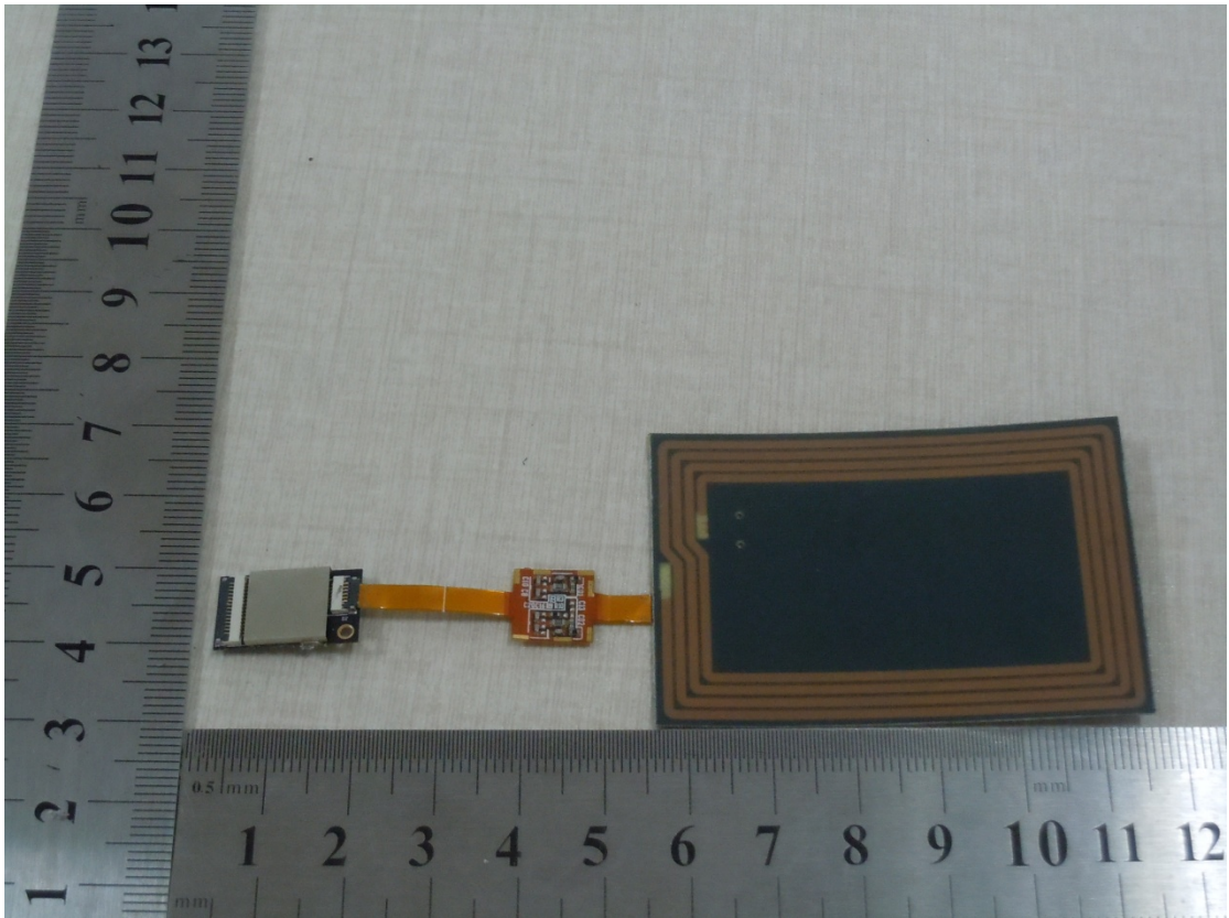
NFC Module:
