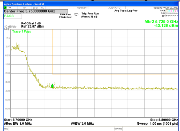
W56_11ac20_Higher_Band edge
