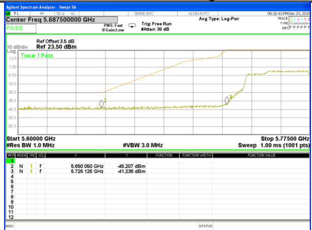
W58_11ac80_Band edge_Left
