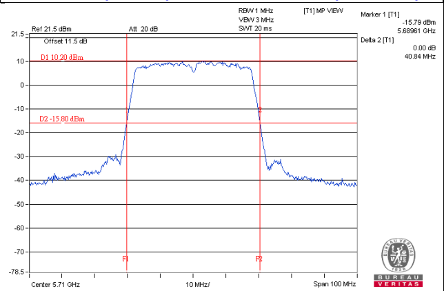
802.11ac (VHT80+80) / Chain 3 - CH130(U_NII-2C)
