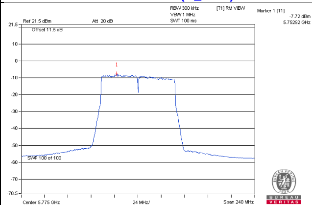
802.11ac (VHT80+80) / Chain 3– CH155(U_NII-3)
