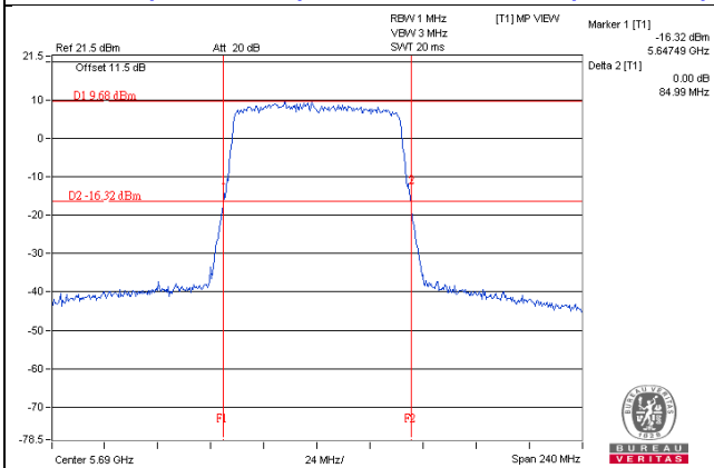
802.11ac (VHT80+80) / Chain 3 - CH138 (U_NII-2C)
