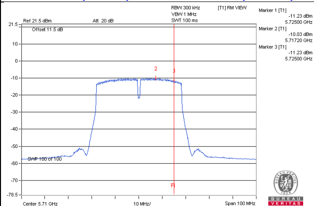
802.11ac (VHT80+80) / Chain 3– CH155(U_NII-3)
