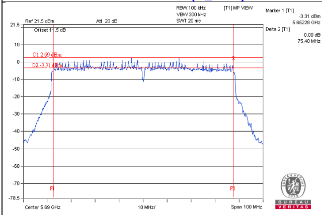
802.11ac (VHT80+80) / Chain 3 - CH138 (U_NII-3)
