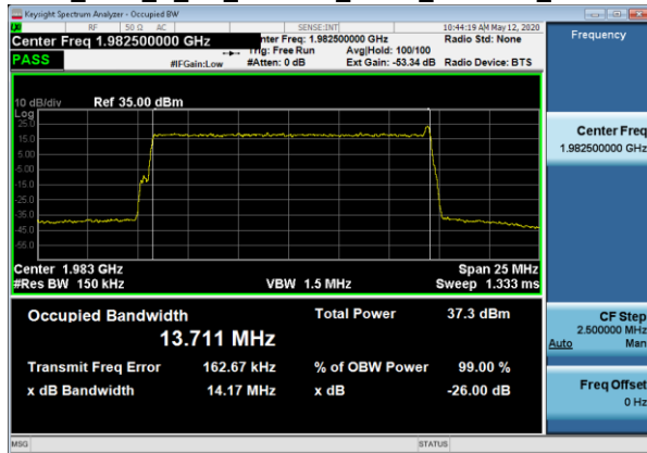
OBW_TM1_1_1C_15MBW_1982_TX1 GB_1982
