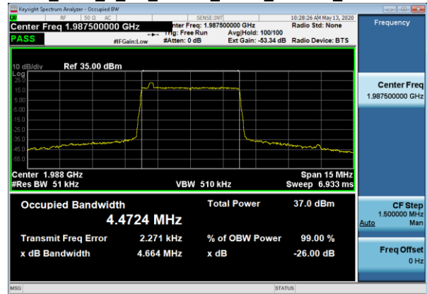
OBW_TM1_1_1C_5MBW_1987_TX1 IB_1987
