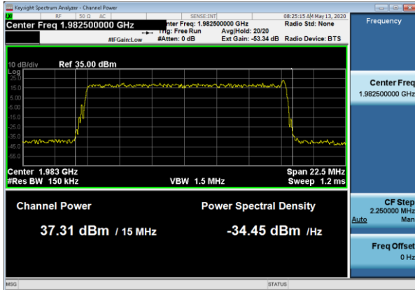
Ch_Power_TM1_1_1C_15MBW_1982_TX1 GB
