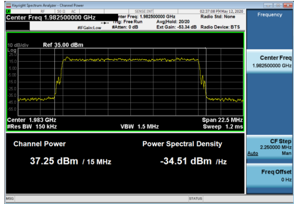
Ch_Power_TM1_1_1C_15MBW_1982_TX1 IB
