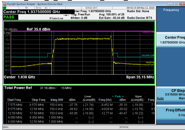
OOBE_TM1_1_1C_15MBW_1937_TX1 GB
