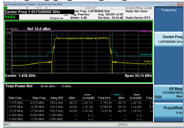
OOBE_TM1_1_1C_15MBW_1937_TX1 IB
