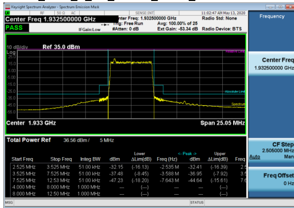
OOBE_TM1_1_1C_5MBW_1932_TX1 IB
