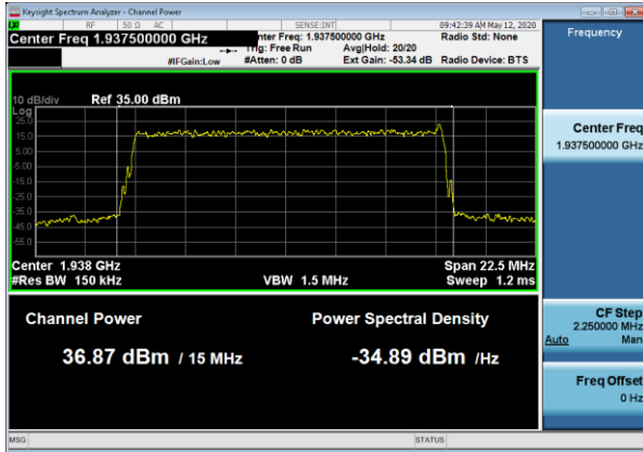
Ch_Power_TM1_1_1C_15MBW_1937_TX1 GB
