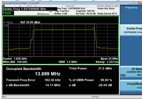
OBW_TM1_1_1C_15MBW_1937_TX1 GB_1937
