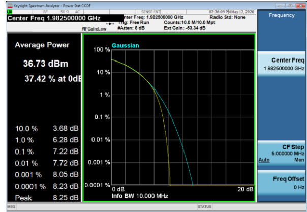
PAR_TM1_1_1C_15MBW_1982_TX1 IB_1982
