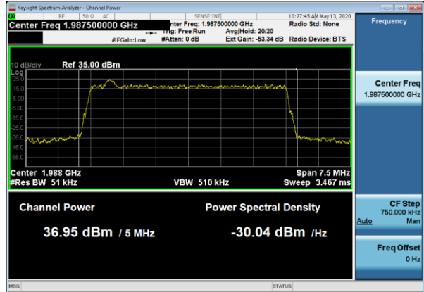
Ch_Power_TM1_1_1C_5MBW_1987_TX1 IB
