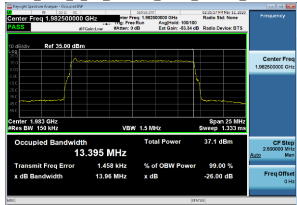
OBW_TM1_1_1C_15MBW_1982_TX1 IB_1982
