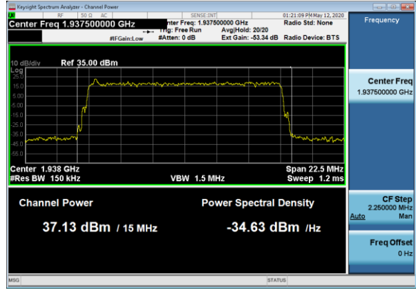
Ch_Power_TM1_1_1C_15MBW_1937_TX1 IB
