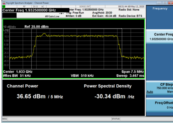
Ch_Power_TM1_1_1C_5MBW_1932_TX1 IB
