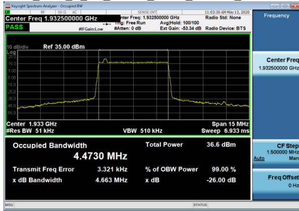
OBW_TM1_1_1C_5MBW_1932_TX1 IB_1932
