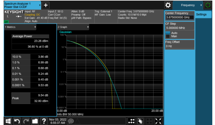
50MHz BW, TM3.1a Channel Frequency 3675MHz
