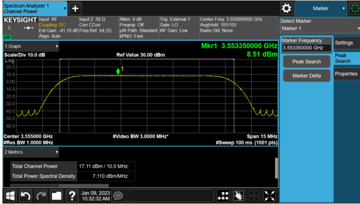
10MHz BW, TM1.1 Channel Frequency 3555MHz
