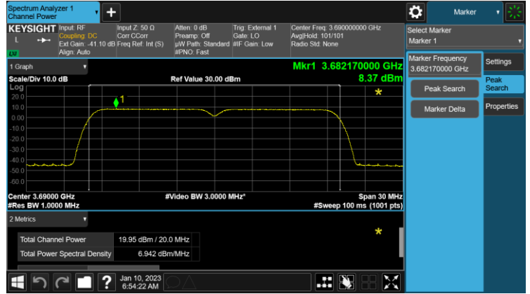
10+10MHz BW, TM1.1 Channel Frequency 3685+3695MHz
