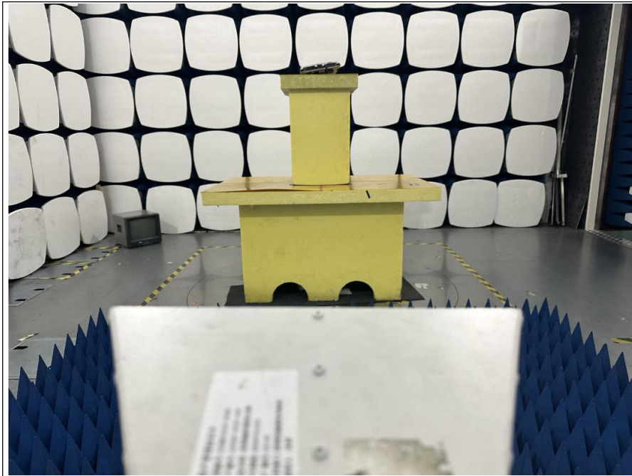
1GHz-18GHz(WiFi)
