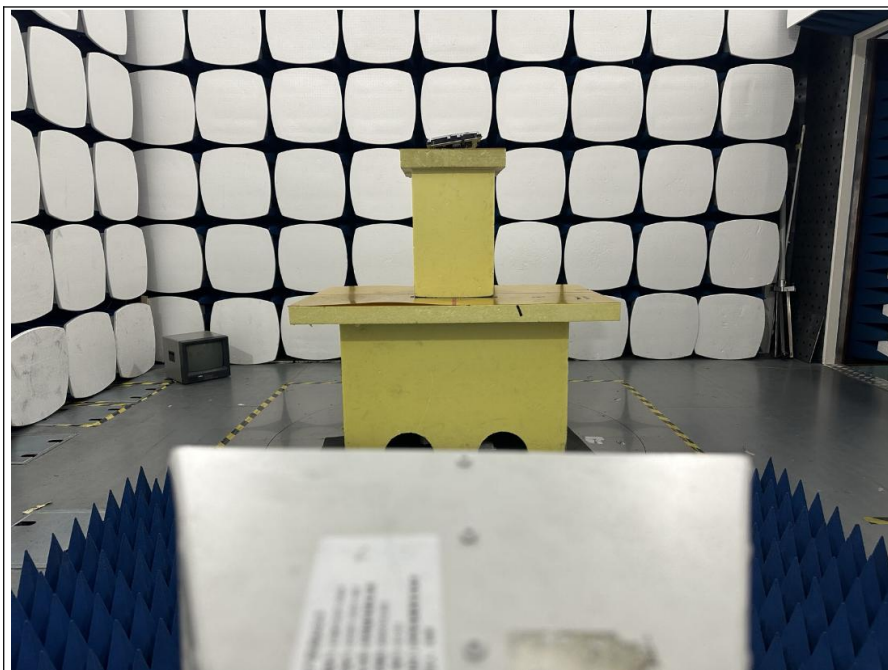
1GHz-18GHz(BT&BLE)
