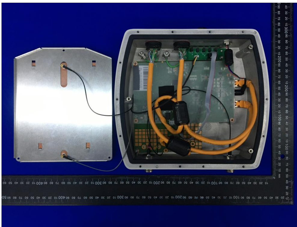
(2)EUT Photo (AX52)
