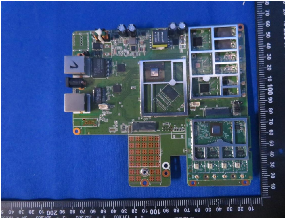
(5)EUT Photo (AX52)
