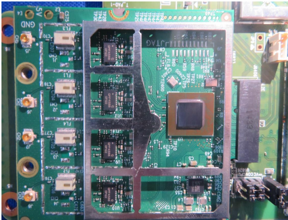
(9) EUT Photo (AX52)
