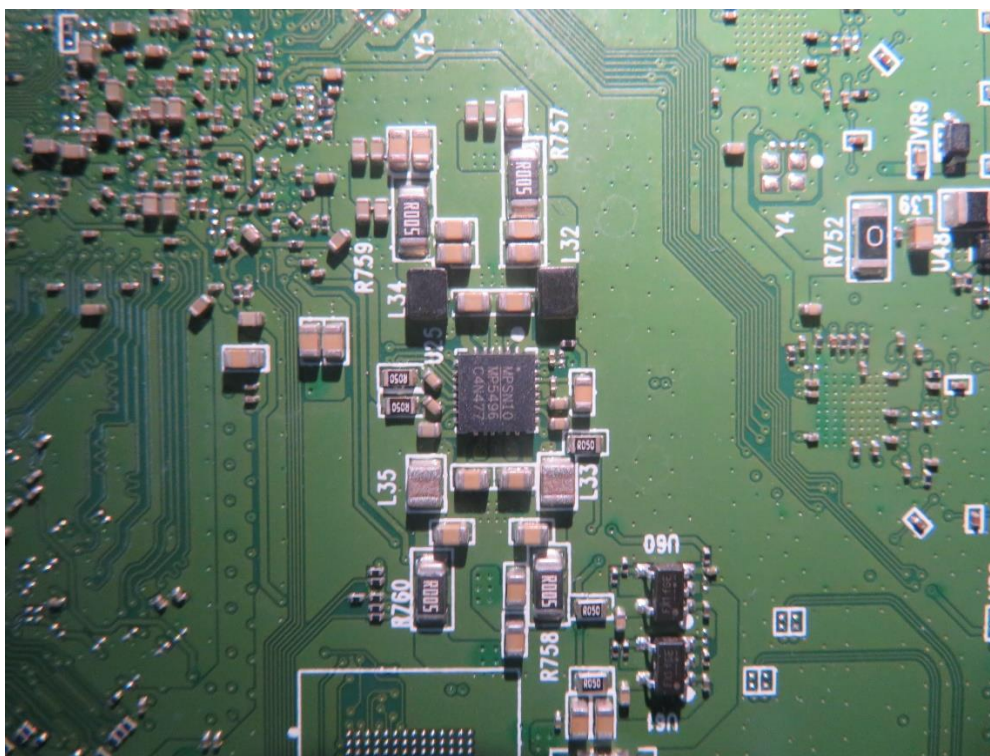
(12) EUT Photo (AX52e)
