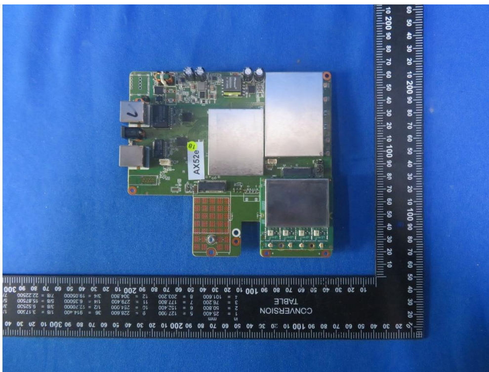
(2) EUT Photo (AX52e)
