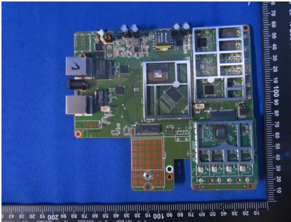
(17) EUT Photo (AX52)
