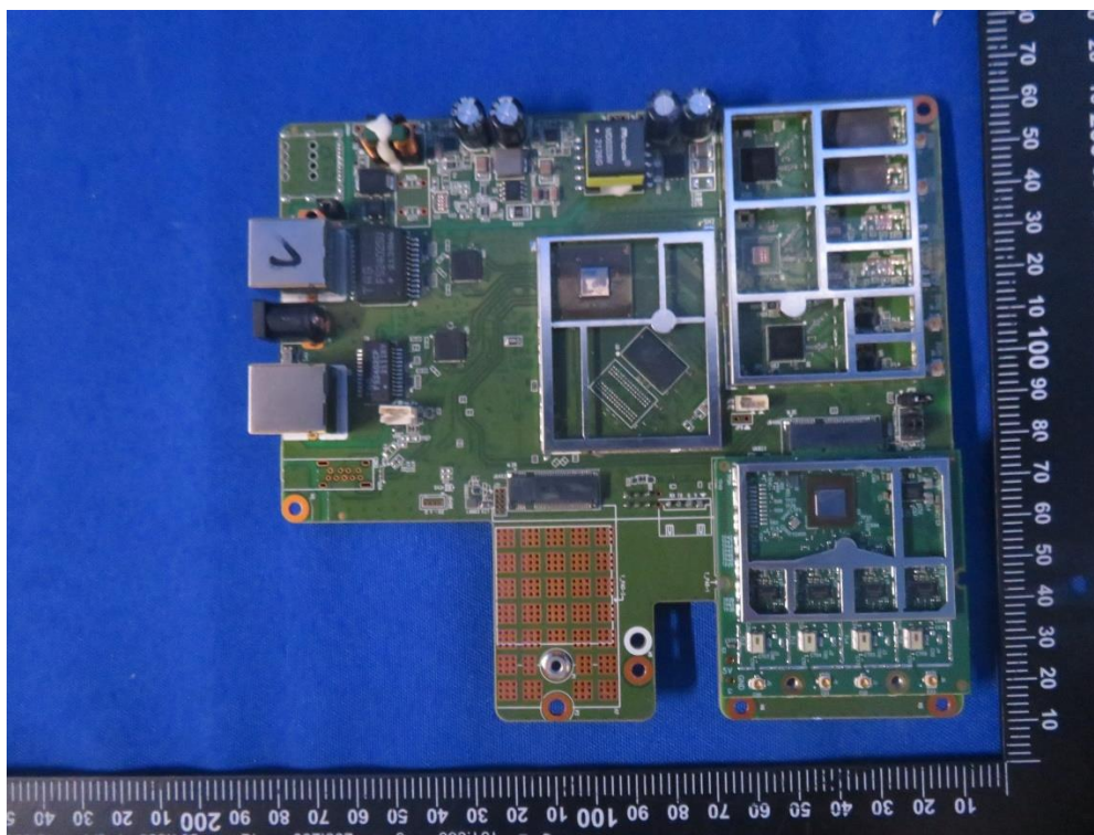
(4) EUT Photo (AX52e)
