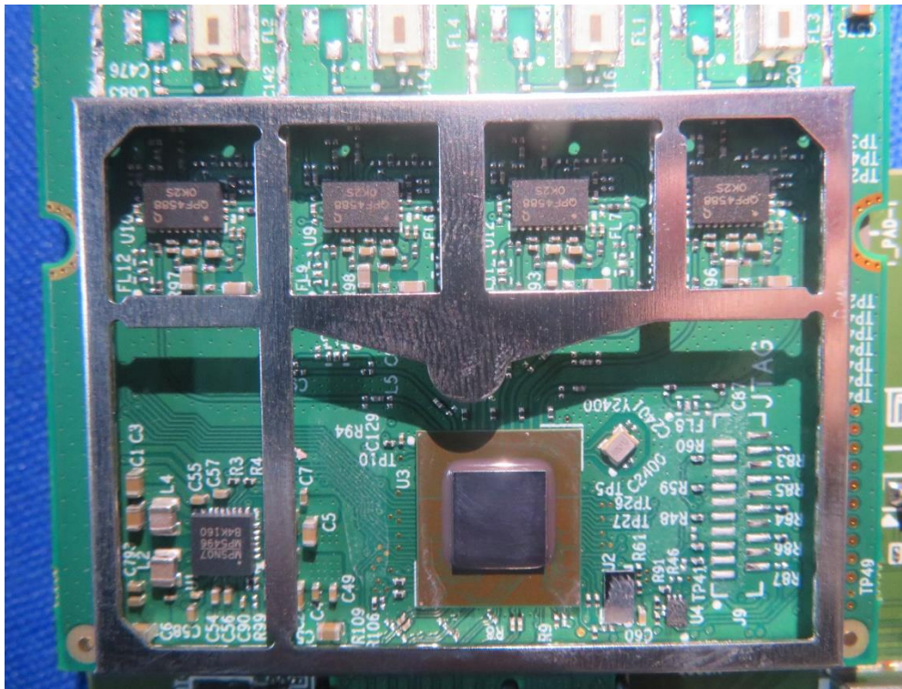
(7) EUT Photo (AX52e)
