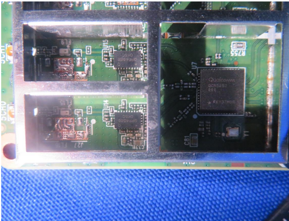
(11) EUT Photo (AX52)
