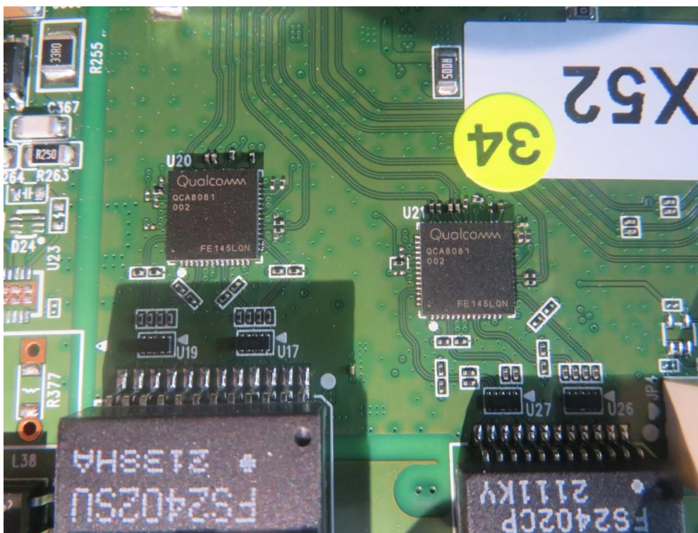
(8)EUT Photo (AX52)
