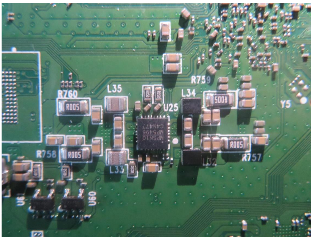
(16) EUT Photo (AX52)
