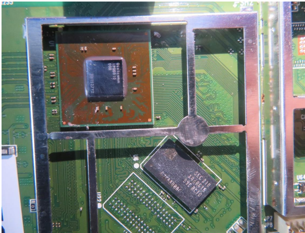
(5) EUT Photo (AX52e)
