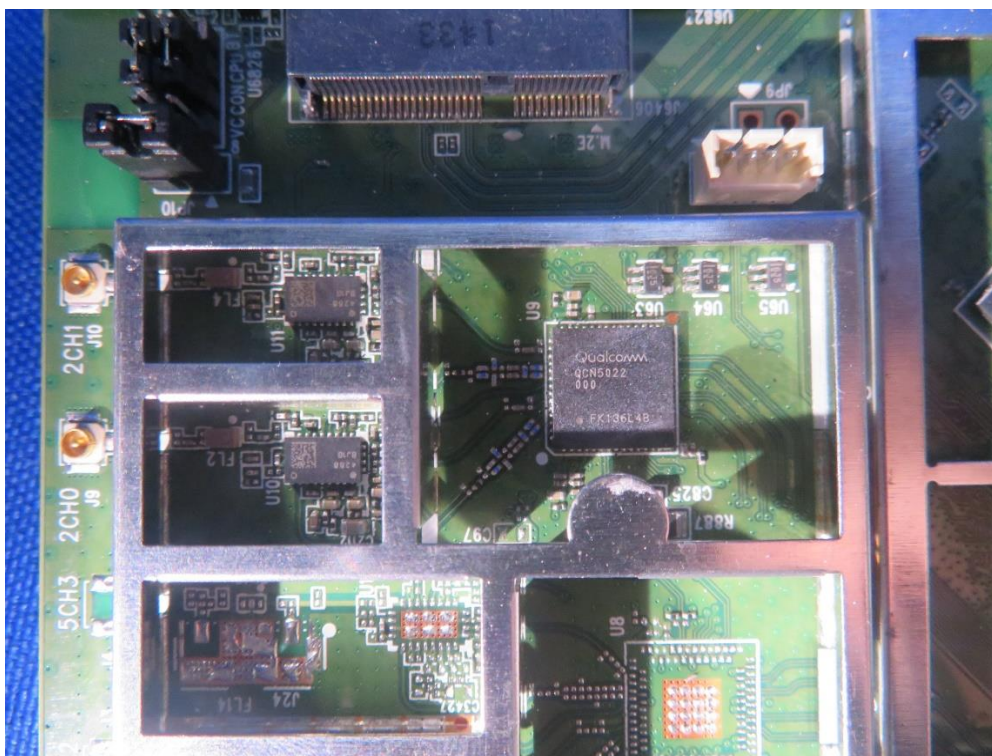
(10) EUT Photo (AX52e)
