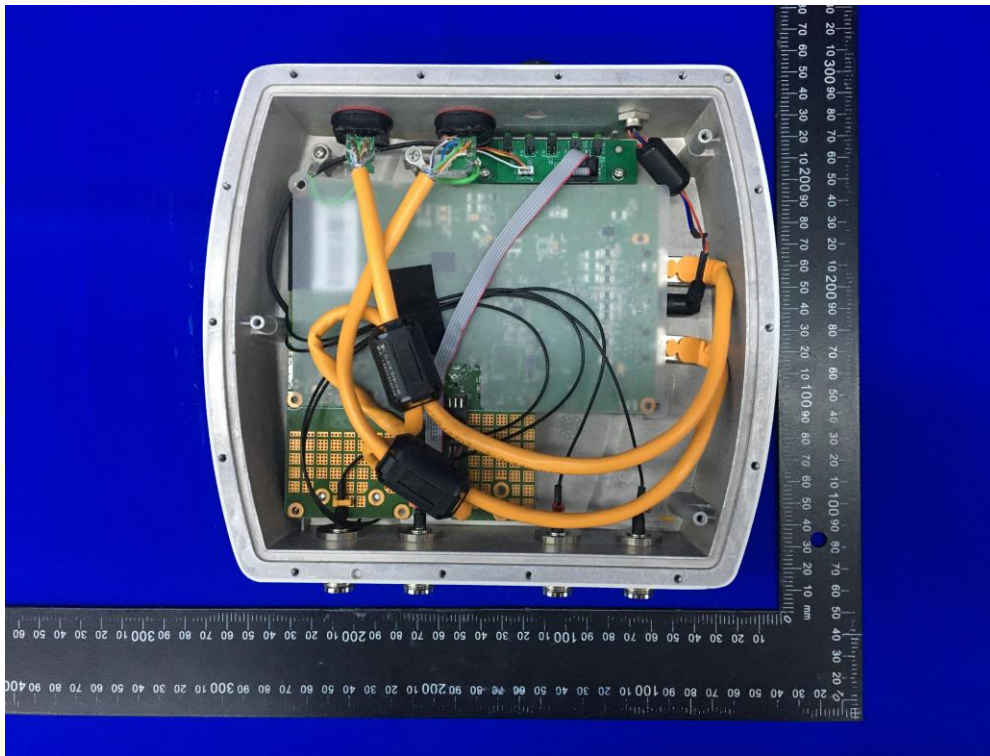
(1) EUT Photo (AX52e)
