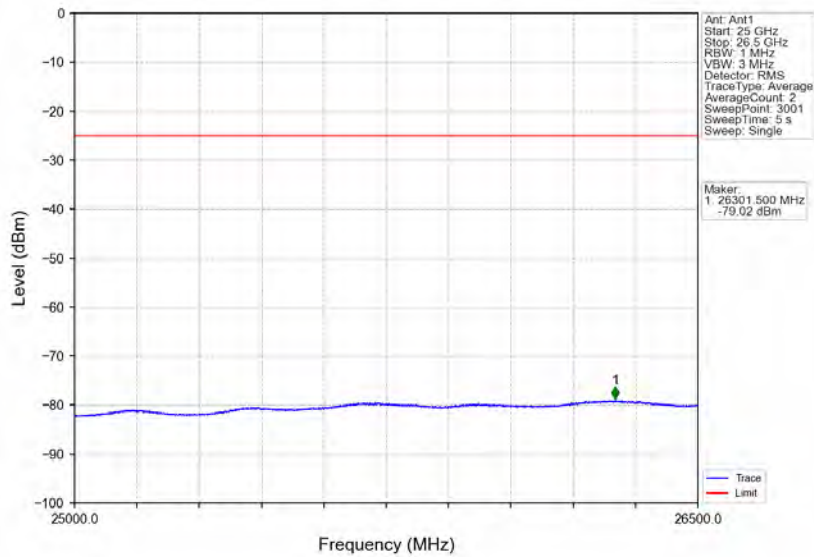
Band7_10MHz_QPSK_HCH_2565MHz_RB_1_49_NTNV
