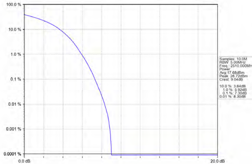
Band7_20MHz_16QAM_LCH_2510MHz_RB_100_0_NTNV
