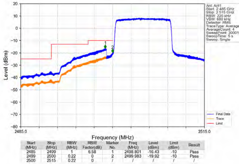
Band7_10MHz_QPSK_LCH_2505MHz_RB_50_0_NTNV
