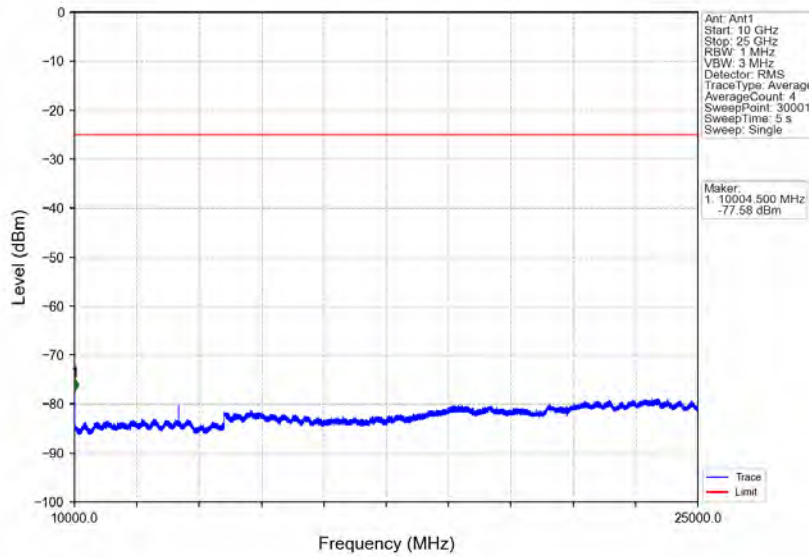
Band7_20MHz_16QAM_LCH_2510MHz_RB_1_0_NTNV
