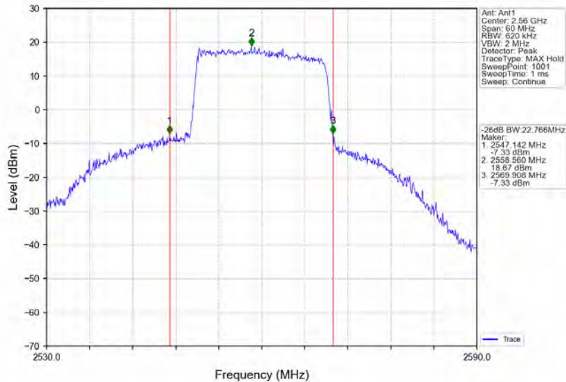
Band7_20MHz_16QAM_HCH_2560MHz_RB_100_0_NTNV
