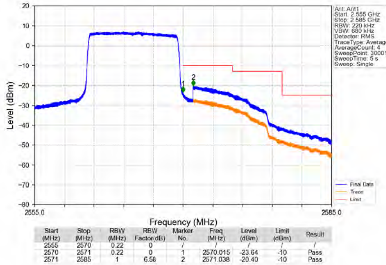
Band7_10MHz_QPSK_HCH_2565MHz_RB_50_0_NTNV
