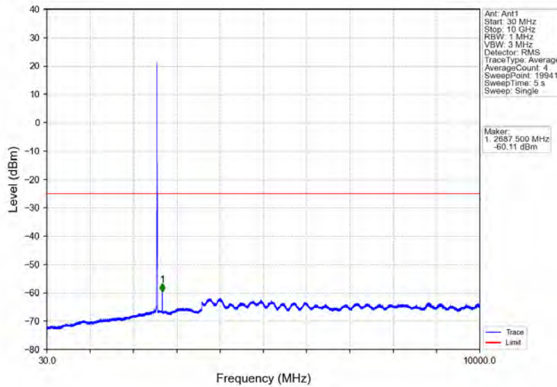
Band7_5MHz_QPSK_HCH_2567.5MHz_RB_1_0_NTNV
