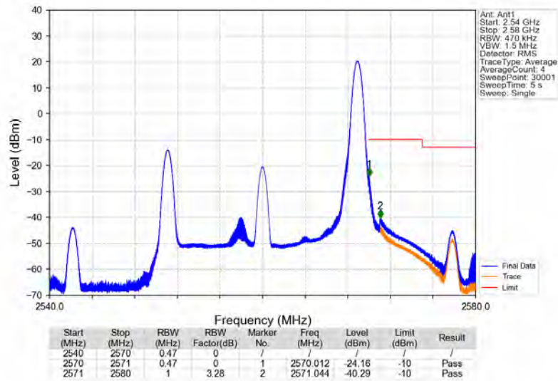
Band7_20MHz_QPSK_HCH_2560MHz_RB_1_99_NTNV
