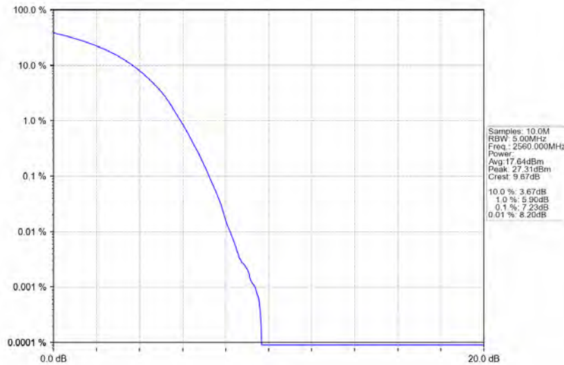
Band7_20MHz_16QAM_HCH_2560MHz_RB_100_0_NTNV
