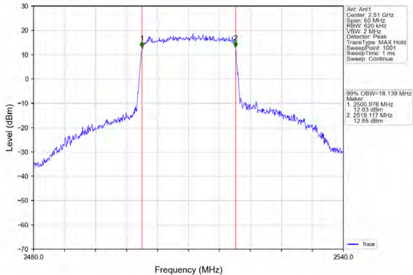
Band7_20MHz_16QAM_LCH_2510MHz_RB_100_0_NTNV
