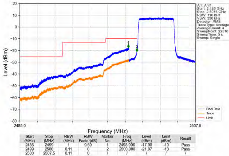
Band7_5MHz_QPSK_LCH_2502.5MHz_RB_25_0_NTNV
