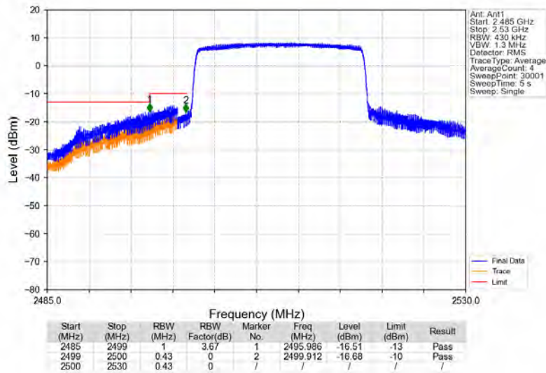
Band7_20MHz_QPSK_LCH_2510MHz_RB_100_0_NTNV
