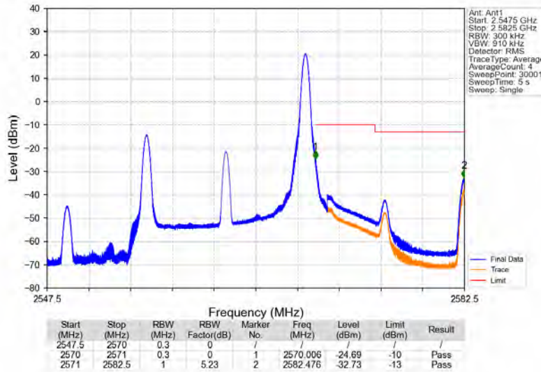
Band7_15MHz_QPSK_HCH_2562.5MHz_RB_1_74_NTNV
