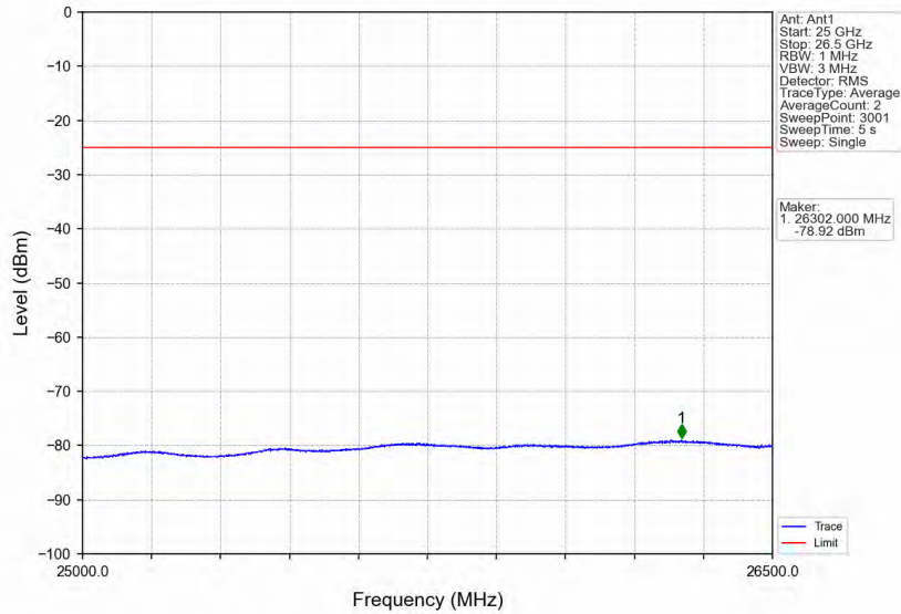
Band7_20MHz_QPSK_HCH_2560MHz_RB_1_99_NTNV
