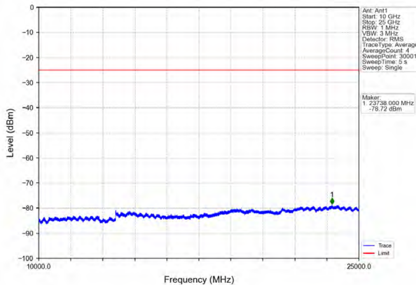
Band7_5MHz_QPSK_HCH_2567.5MHz_RB_1_0_NTNV
