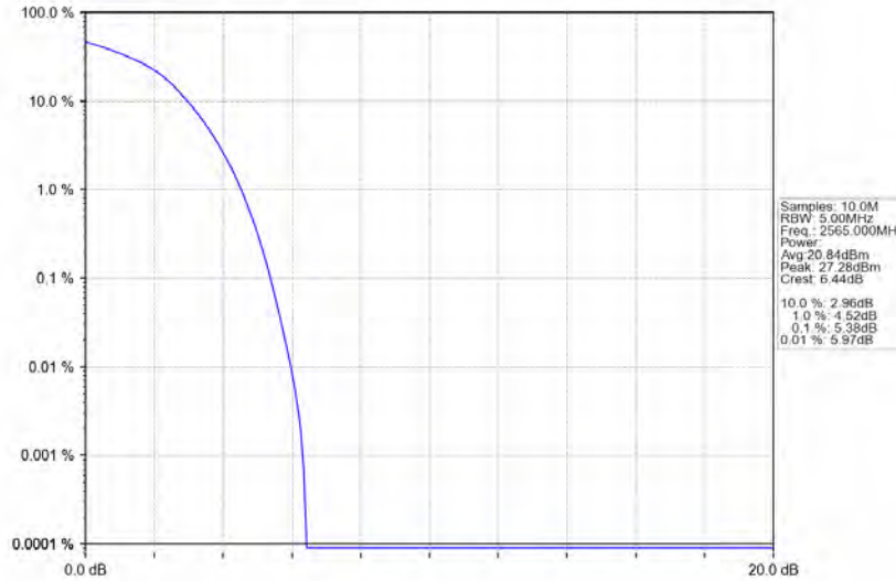
Band7_10MHz_QPSK_HCH_2565MHz_RB_50_0_NTNV
