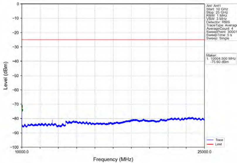
Band7_20MHz_QPSK_LCH_2510MHz_RB_1_0_NTNV
