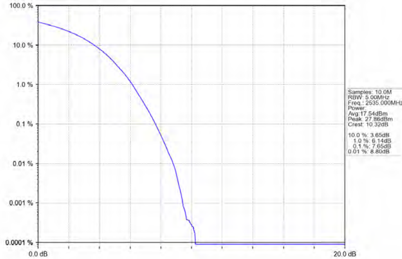
Band7_20MHz_16QAM_MCH_2535MHz_RB_100_0_NTNV
