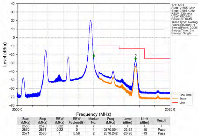
Band7_10MHz_QPSK_HCH_2565MHz_RB_1_49_NTNV
