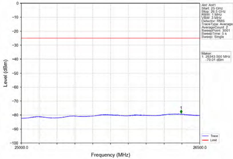
Band7_20MHz_16QAM_LCH_2510MHz_RB_100_0_NTNV
