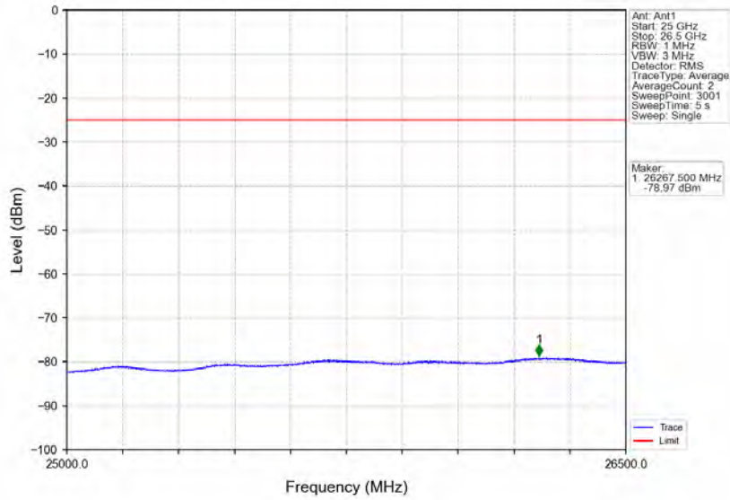
Band7_20MHz_16QAM_HCH_2560MHz_RB_1_0_NTNV
