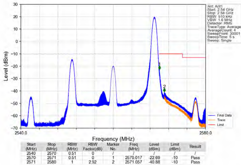
Band7_20MHz_16QAM_HCH_2560MHz_RB_1_99_NTNV
