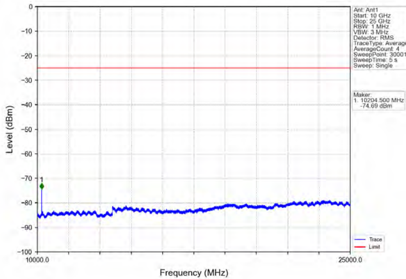
Band7_20MHz_16QAM_HCH_2560MHz_RB_1_0_NTNV
