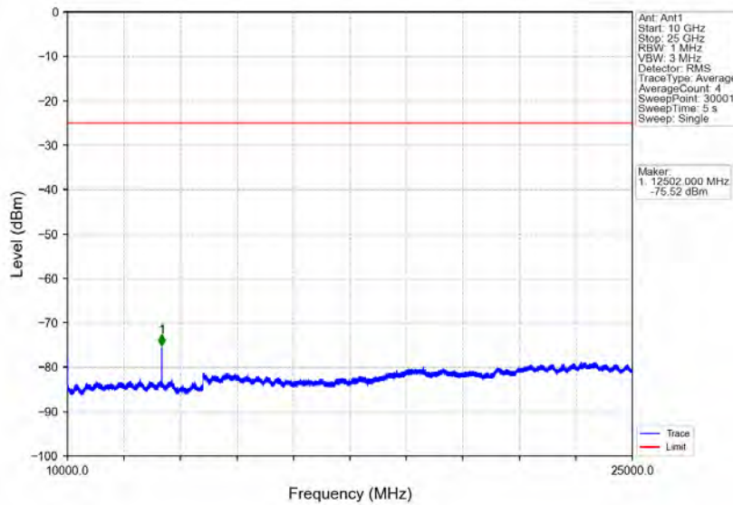
Band7_5MHz_QPSK_LCH_2502.5MHz_RB_1_0_NTNV
