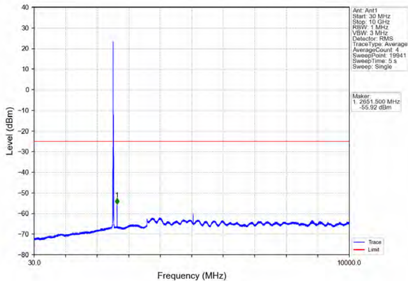
Band7_10MHz_QPSK_MCH_2535MHz_RB_1_0_NTNV
