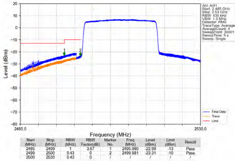
Band7_20MHz_16QAM_LCH_2510MHz_RB_100_0_NTNV
