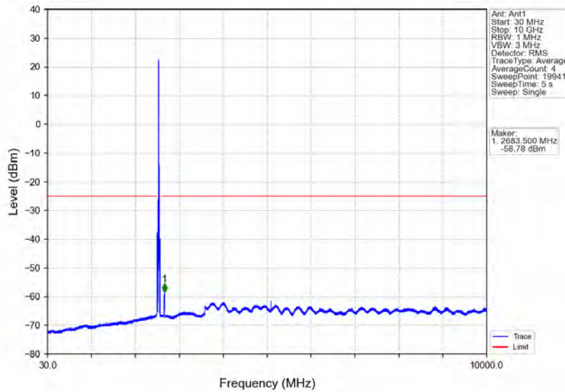
Band7_20MHz_QPSK_HCH_2560MHz_RB_1_0_NTNV
