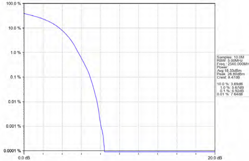
Band7_20MHz_QPSK_HCH_2560MHz_RB_100_0_NTNV
