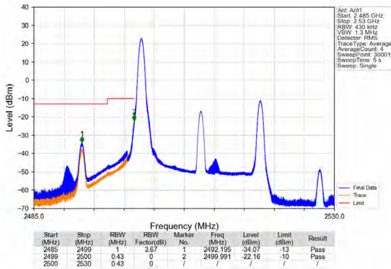
Band7_20MHz_16QAM_LCH_2510MHz_RB_1_0_NTNV
