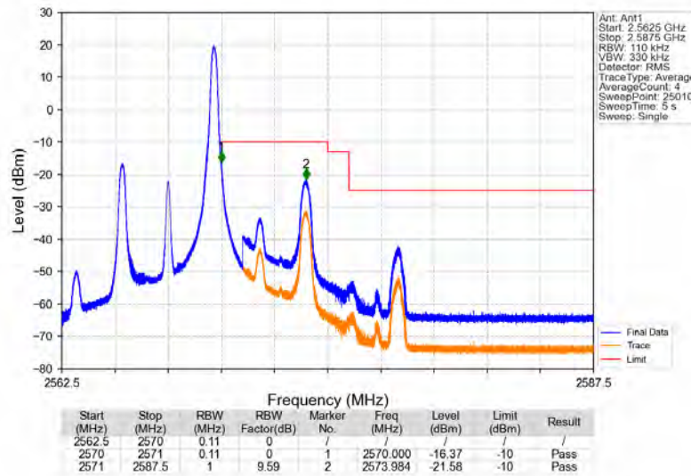
Band7_5MHz_QPSK_HCH_2567.5MHz_RB_1_24_NTNV
