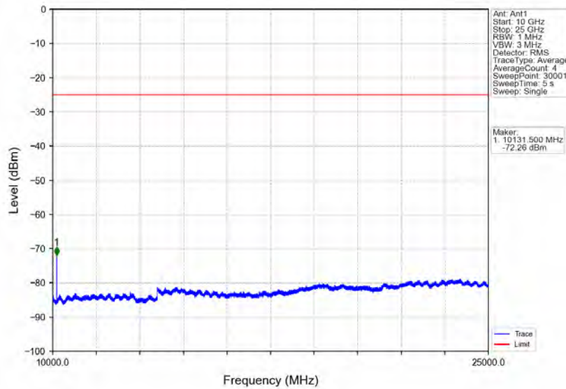
Band7_5MHz_QPSK_MCH_2535MHz_RB_1_0_NTNV
