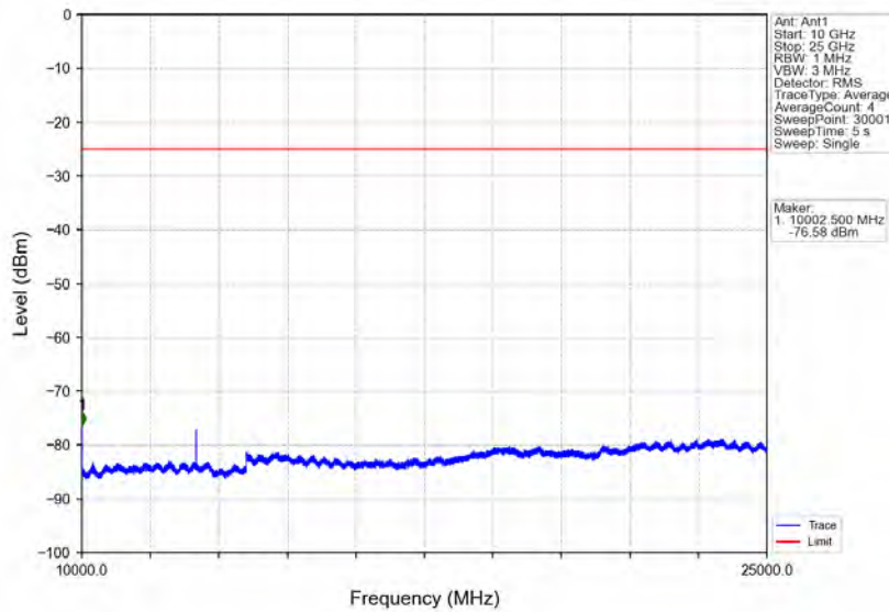
Band7_10MHz_QPSK_LCH_2505MHz_RB_1_0_NTNV
