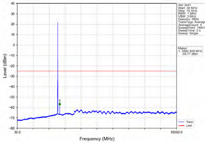
Band7_10MHz_QPSK_HCH_2565MHz_RB_1_0_NTNV
