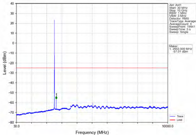
Band7_5MHz_QPSK_MCH_2535MHz_RB_1_0_NTNV
