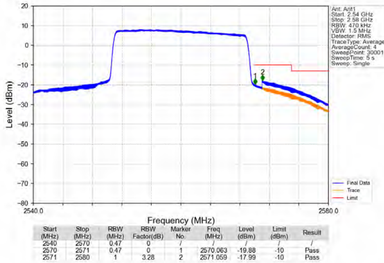
Band7_20MHz_QPSK_HCH_2560MHz_RB_100_0_NTNV
