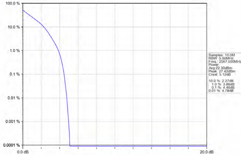
Band7_5MHz_QPSK_HCH_2567.5MHz_RB_25_0_NTNV
