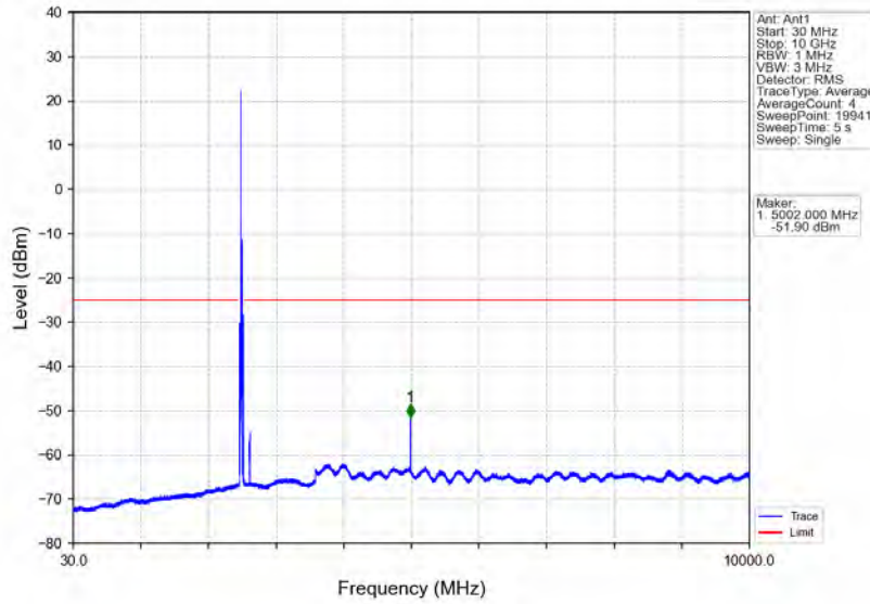
Band7_20MHz_16QAM_LCH_2510MHz_RB_1_0_NTNV
