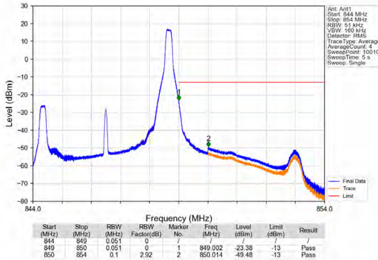
Band5_5MHz_QPSK_HCH_846.5MHz_RB_1_24_NTNV
