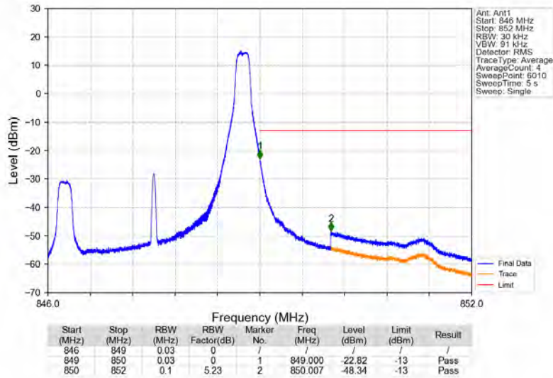
Band5_3MHz_QPSK_HCH_847.5MHz_RB_1_14_NTNV
