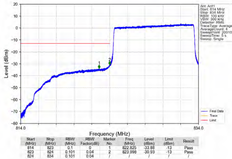
Band5_10MHz_QPSK_LCH_829MHz_RB_50_0_NTNV
