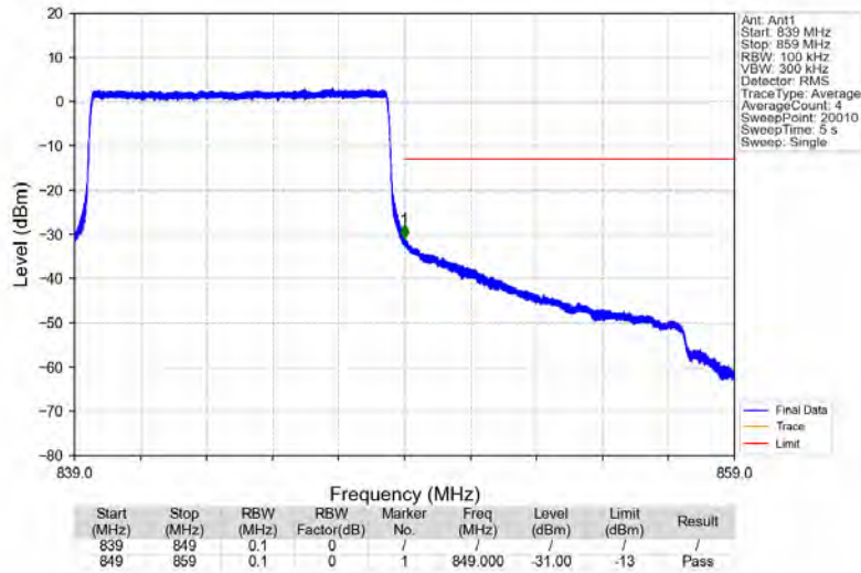
Band5_10MHz_QPSK_HCH_844MHz_RB_50_0_NTNV
