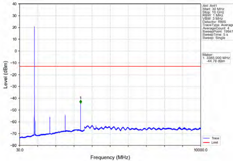
Band5_3MHz_QPSK_HCH_847.5MHz_RB_1_14_NTNV
