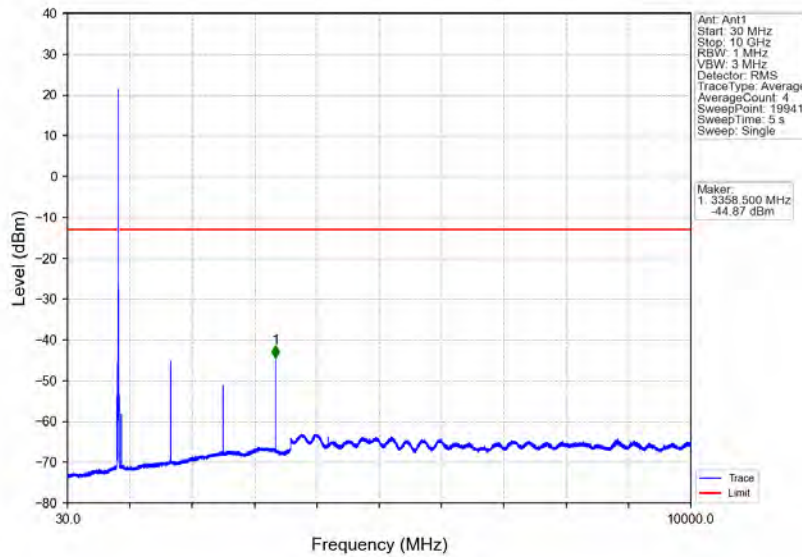
Band5_10MHz_QPSK_HCH_844MHz_RB_1_49_NTNV
