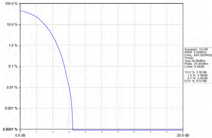
Band5_10MHz_QPSK_HCH_844MHz_RB_50_0_NTNV
