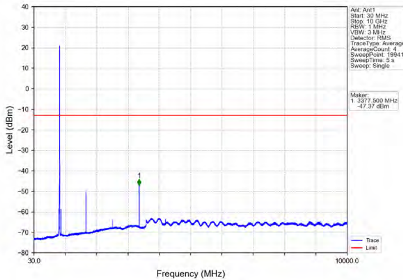
Band5_5MHz_QPSK_HCH_846.5MHz_RB_1_24_NTNV
