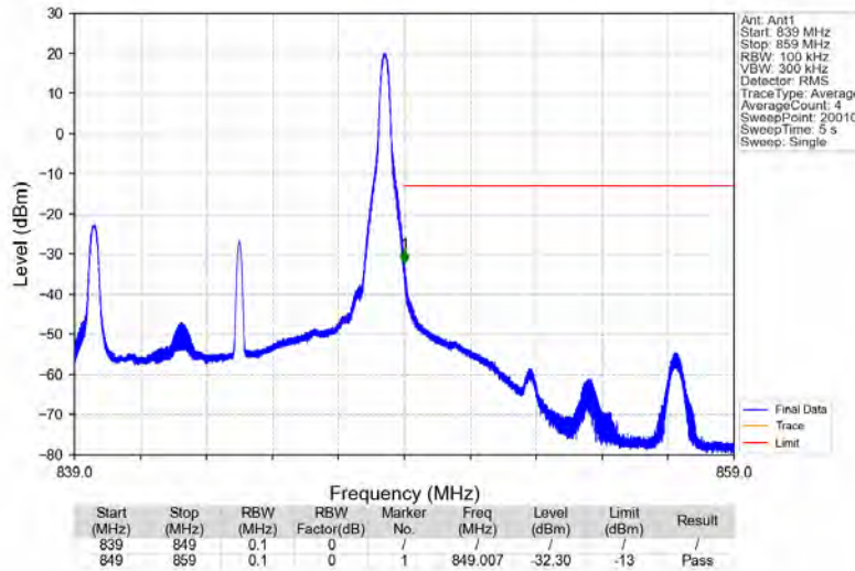
Band5_10MHz_QPSK_HCH_844MHz_RB_1_49_NTNV
