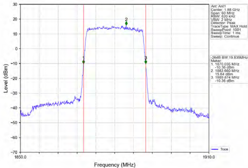
Band2_20MHz_QPSK_MCH_1880MHz_RB_100_0_NTNV
