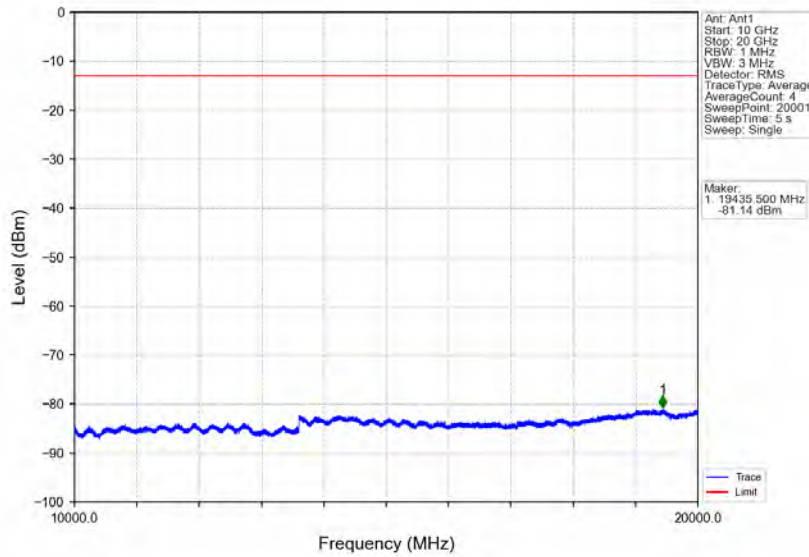
Band2_1.4MHz_QPSK_MCH_1880MHz_RB_1_0_NTNV
