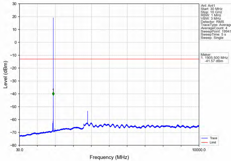
Band2_1.4MHz_QPSK_HCH_1909.3MHz_RB_1_0_NTV
