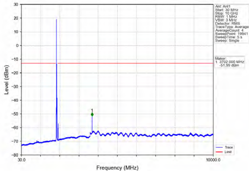
Band2_20MHz_16QAM_LCH_1860MHz_RB_1_0_NTNV
