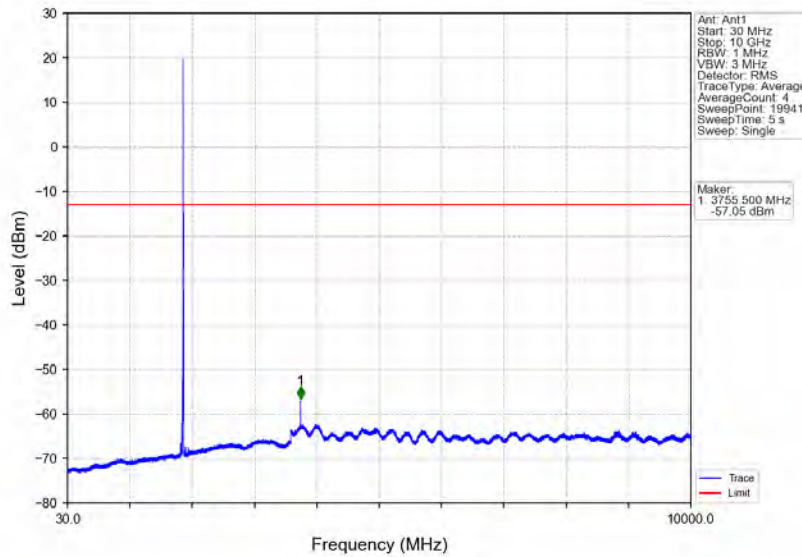
Band2_5MHz_QPSK_MCH_1880MHz_RB_1_0_NTNV
