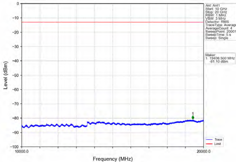
Band2_20MHz_QPSK_HCH_1900MHz_RB_1_0_NTNV
