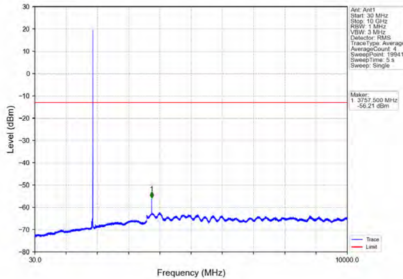
Band2_3MHz_QPSK_MCH_1880MHz_RB_1_0_NTNV
