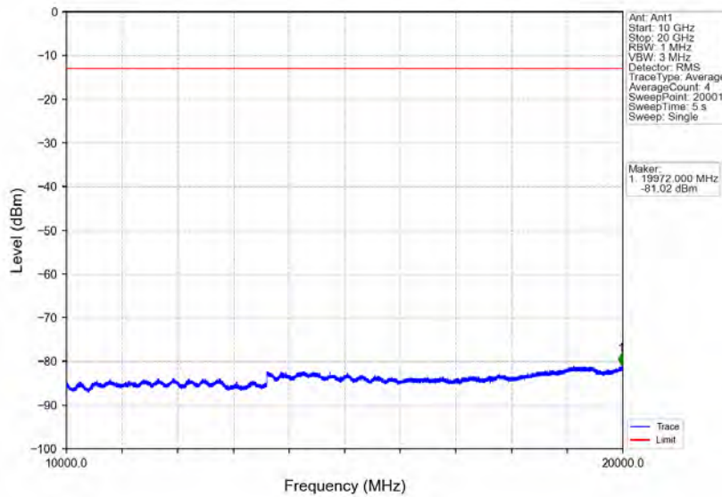
Band2_10MHz_16QAM_LCH_1855MHz_RB_50_0_NTNV
