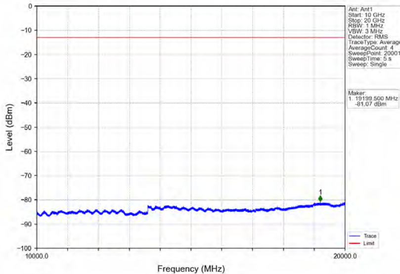
Band2_15MHz_QPSK_HCH_1902.5MHz_RB_1_0_NTNV
