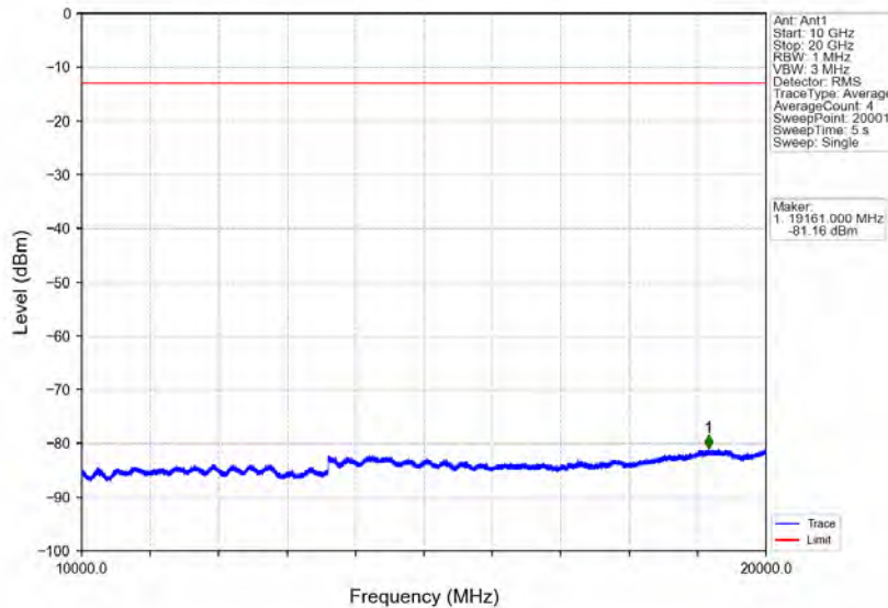
Band2_3MHz_16QAM_MCH_1880MHz_RB_1_0_NTNV
