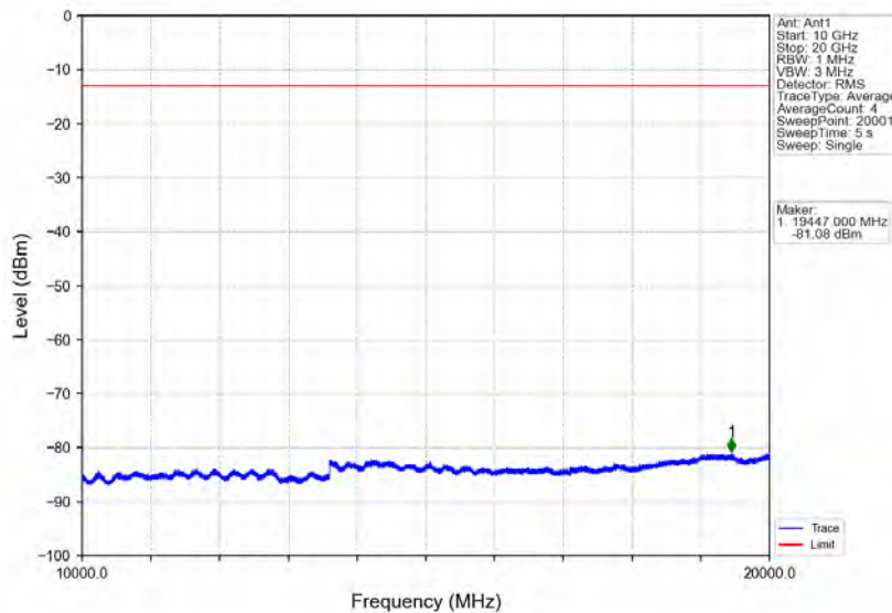
Band2_15MHz_QPSK_MCH_1880MHz_RB_1_0_NTNV
