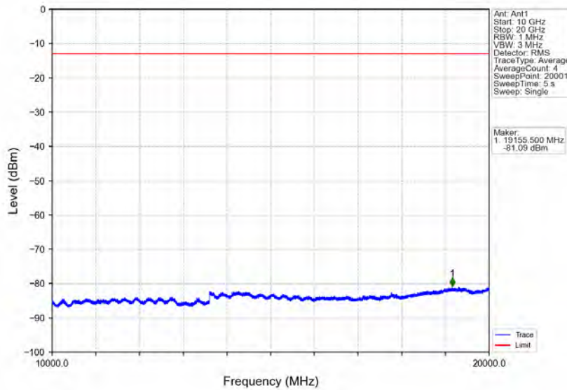
Band2_20MHz_16QAM_LCH_1860MHz_RB_100_0_NTNV
