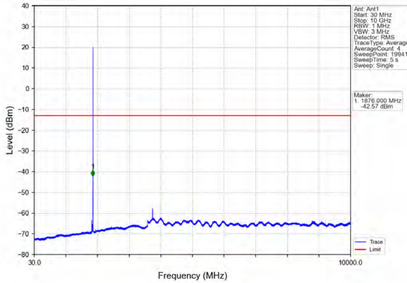
Band2_1.4MHz_QPSK_MCH_1880MHz_RB_1_0_NTNV
