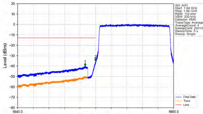
Band2_10MHz_16QAM_LCH_1855MHz_RB_50_0_NTNV
