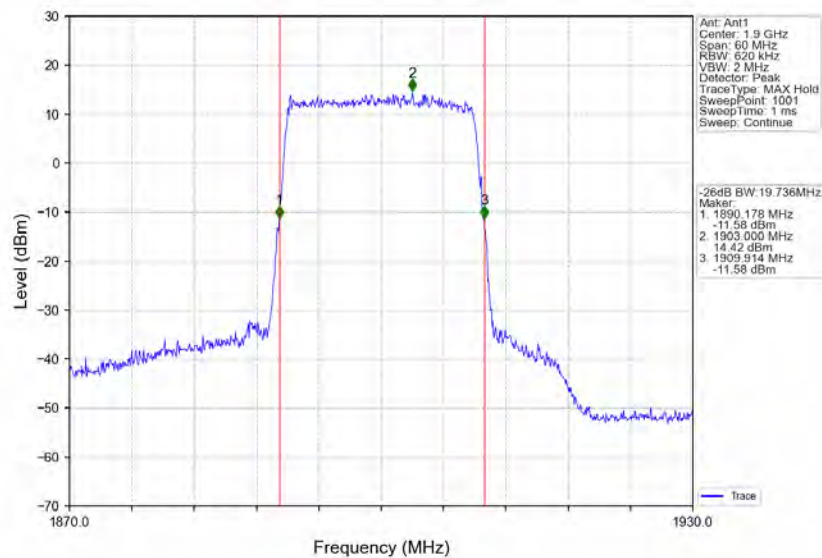
Band2_20MHz_16QAM_HCH_1900MHz_RB_100_0_NTNV
