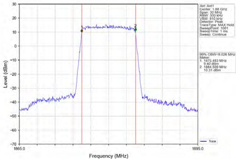
Band2_10MHz_QPSK_MCH_1880MHz_RB_50_0_NTNV
