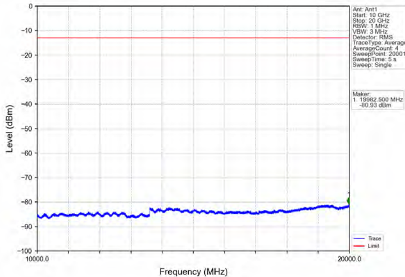
Band2_1.4MHz_QPSK_HCH_1909.3MHz_RB_1_0_NTV
