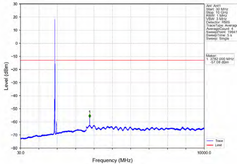
Band2_20MHz_16QAM_HCH_1900MHz_RB_1_0_NTNV
