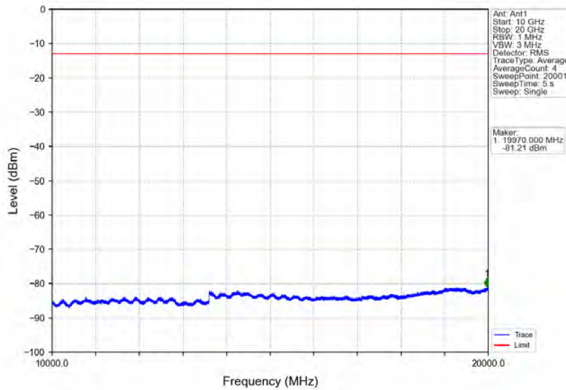
Band2_10MHz_QPSK_LCH_1855MHz_RB_50_0_NTNV
