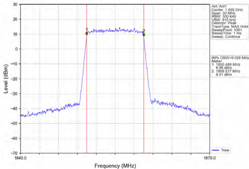
Band2_10MHz_16QAM_LCH_1855MHz_RB_50_0_NTNV
