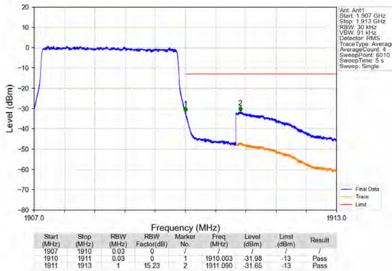
Band2_3MHz_QPSK_HCH_1908.5MHz_RB_15_0_NTNV
