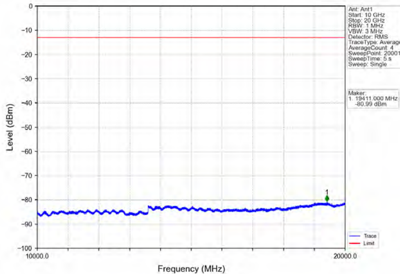
Band2_20MHz_16QAM_HCH_1900MHz_RB_1_0_NTNV
