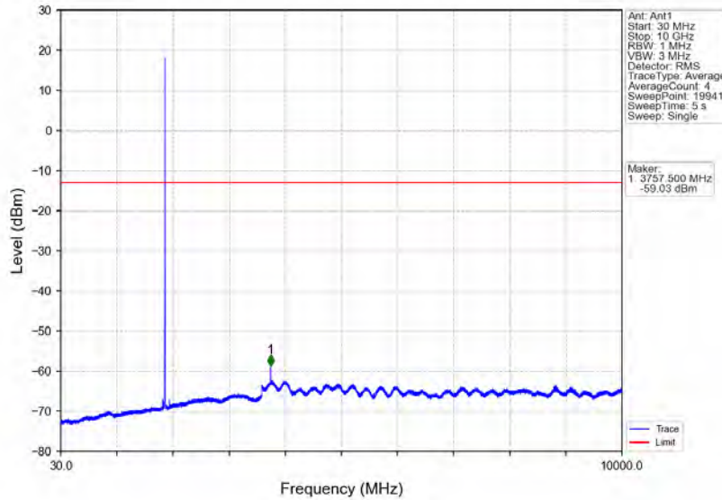
Band2_3MHz_16QAM_MCH_1880MHz_RB_1_0_NTNV
