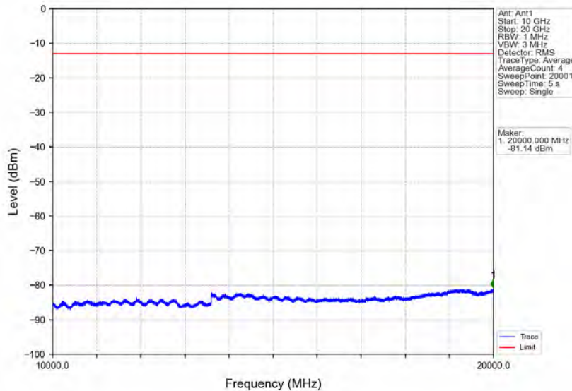
Band2_20MHz_QPSK_MCH_1880MHz_RB_1_0_NTNV
