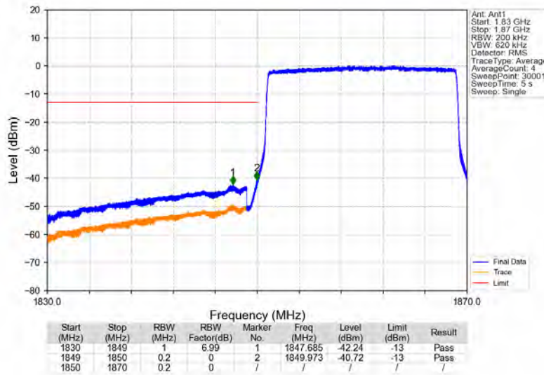
Band2_20MHz_16QAM_LCH_1860MHz_RB_100_0_NTNV
