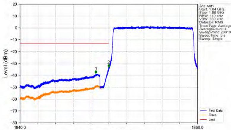
Band2_10MHz_QPSK_LCH_1855MHz_RB_50_0_NTNV
