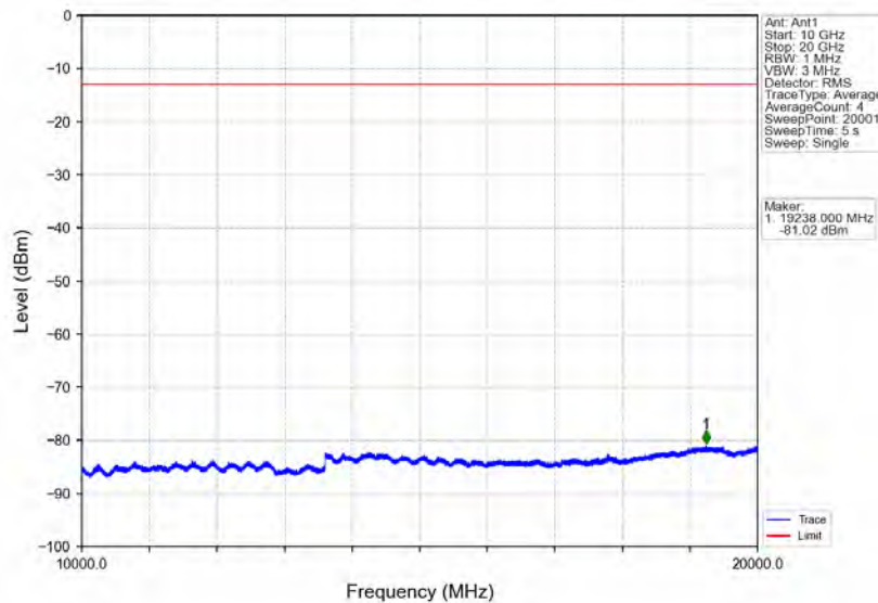
Band2_10MHz_16QAM_MCH_1880MHz_RB_1_0_NTNV
