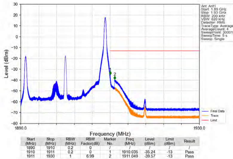
Band2_20MHz_16QAM_HCH_1900MHz_RB_1_99_NTNV
