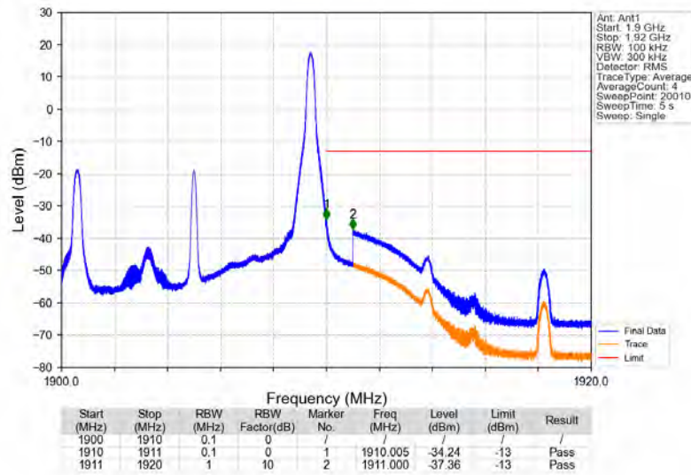
Band2_10MHz_QPSK_HCH_1905MHz_RB_1_49_NTNV
