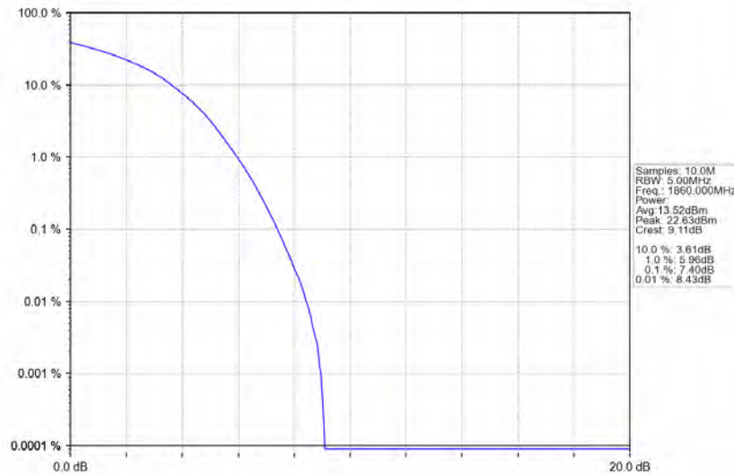
Band2_20MHz_16QAM_LCH_1860MHz_RB_100_0_NTNV
