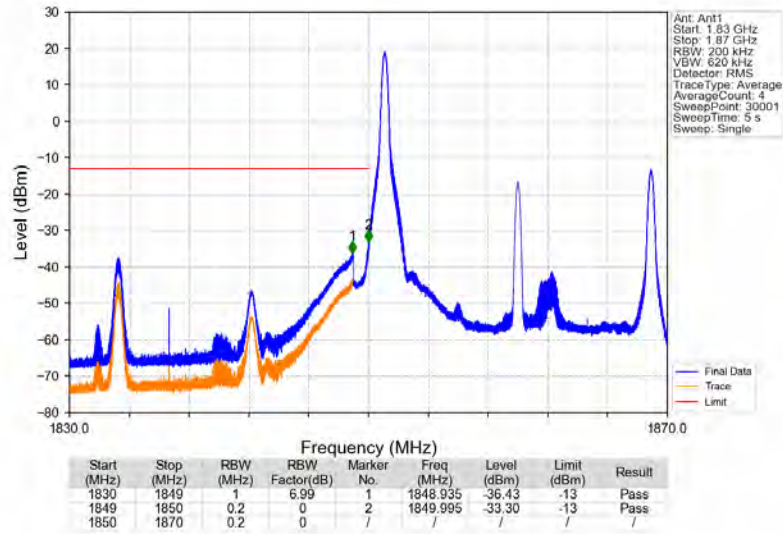
Band2_20MHz_16QAM_LCH_1860MHz_RB_1_0_NTNV
