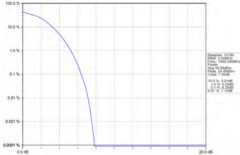
Band2_10MHz_16QAM_MCH_1880MHz_RB_50_0_NTNV
