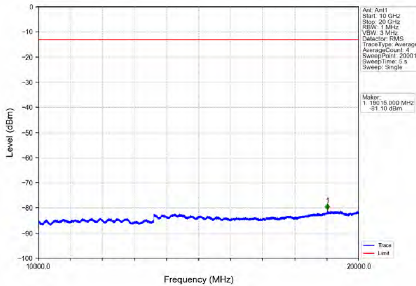
Band2_20MHz_QPSK_LCH_1860MHz_RB_100_0_NTNV
