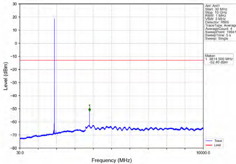
Band2_3MHz_QPSK_HCH_1908.5MHz_RB_1_0_NTNV
