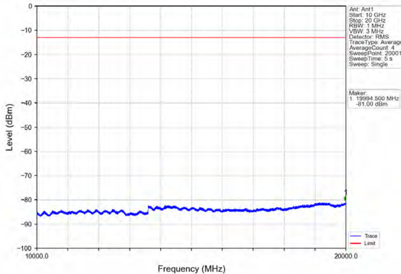
Band2_10MHz_QPSK_MCH_1880MHz_RB_1_0_NTNV
