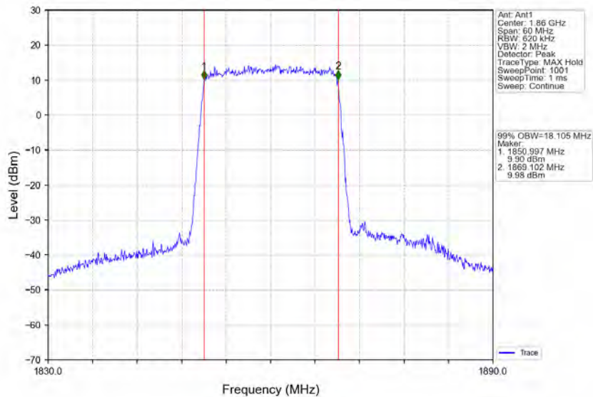
Band2_20MHz_16QAM_LCH_1860MHz_RB_100_0_NTNV
