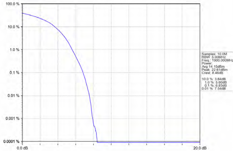
Band2_20MHz_QPSK_HCH_1900MHz_RB_100_0_NTNV
