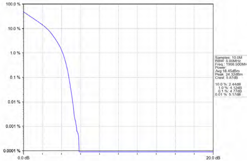
Band2_3MHz_QPSK_HCH_1908.5MHz_RB_15_0_NTNV
