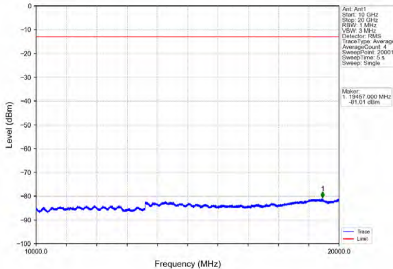
Band2_3MHz_QPSK_HCH_1908.5MHz_RB_1_0_NTNV
