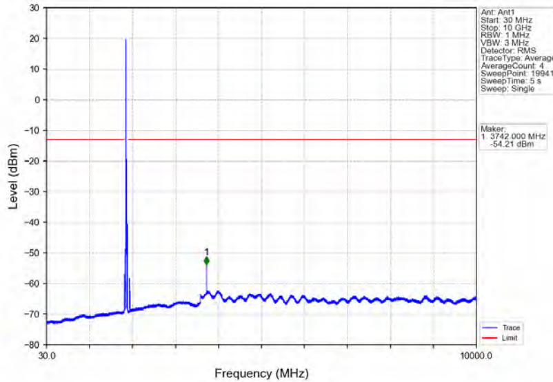
Band2_20MHz_QPSK_MCH_1880MHz_RB_1_0_NTNV
