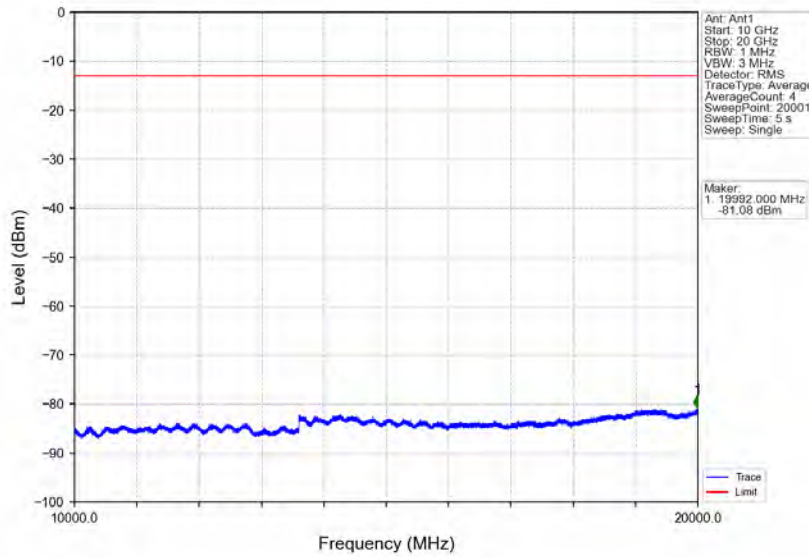
Band2_10MHz_QPSK_HCH_1905MHz_RB_1_0_NTNV
