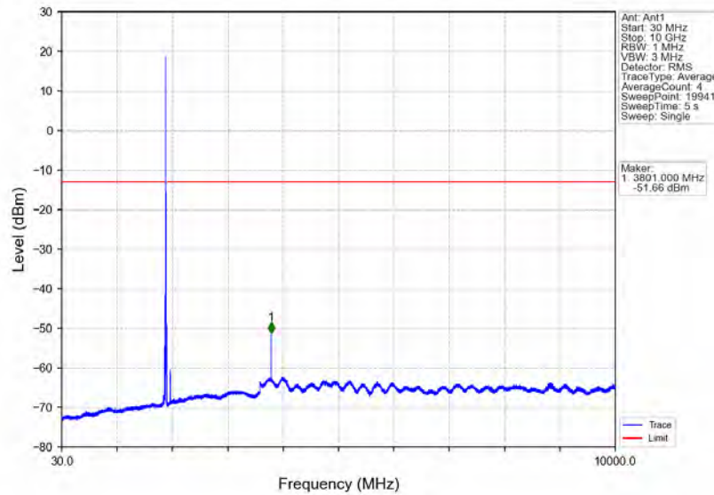
Band2_10MHz_16QAM_HCH_1905MHz_RB_1_0_NTNV
