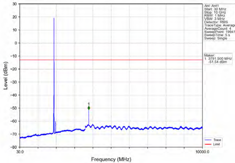
Band2_15MHz_QPSK_HCH_1902.5MHz_RB_1_0_NTNV
