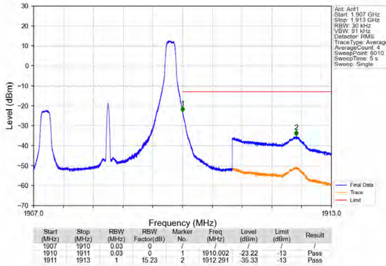
Band2_3MHz_QPSK_HCH_1908.5MHz_RB_1_14_NTNV
