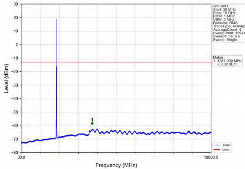
Band2_10MHz_16QAM_MCH_1880MHz_RB_1_0_NTNV
