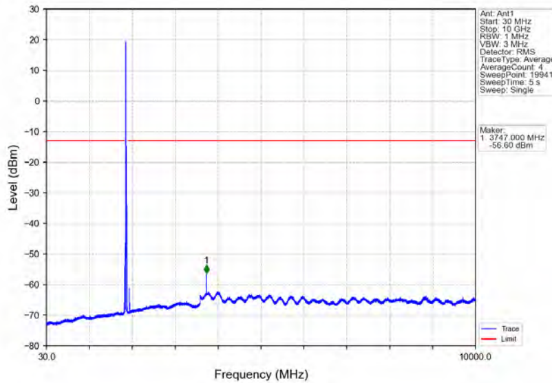
Band2_15MHz_QPSK_MCH_1880MHz_RB_1_0_NTNV
