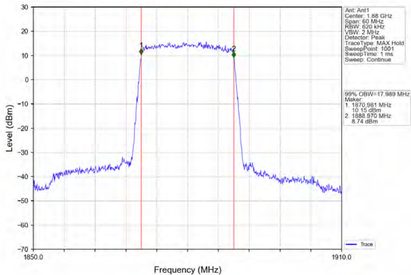
Band2_20MHz_QPSK_MCH_1880MHz_RB_100_0_NTNV
