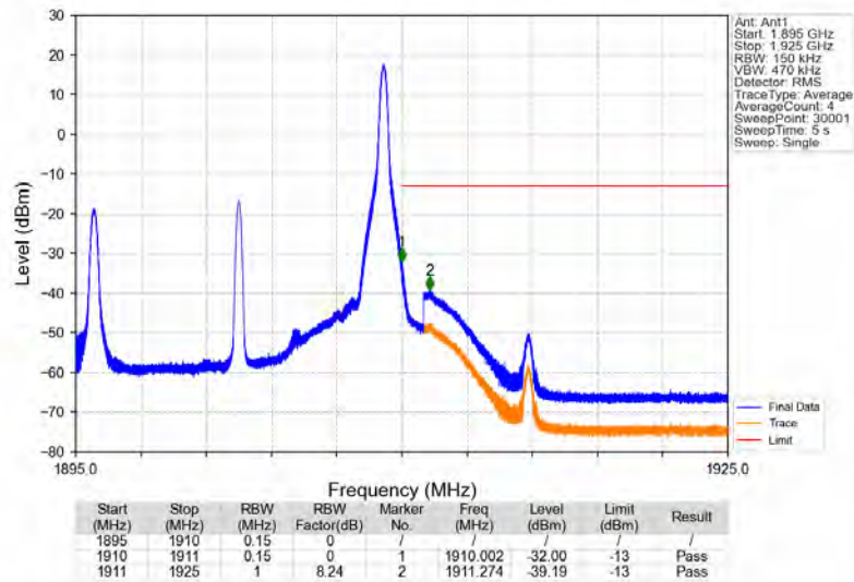
Band2_15MHz_16QAM_HCH_1902.5MHz_RB_1_74_NTNV
