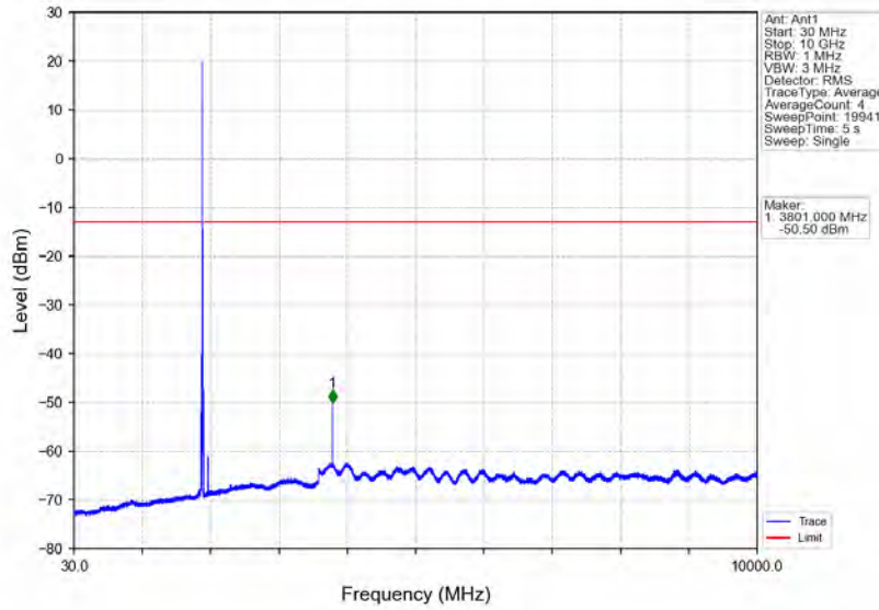
Band2_10MHz_QPSK_HCH_1905MHz_RB_1_0_NTNV
