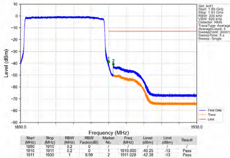
Band2_20MHz_16QAM_HCH_1900MHz_RB_100_0_NTNV
