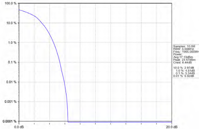
Band2_10MHz_QPSK_HCH_1905MHz_RB_50_0_NTNV
