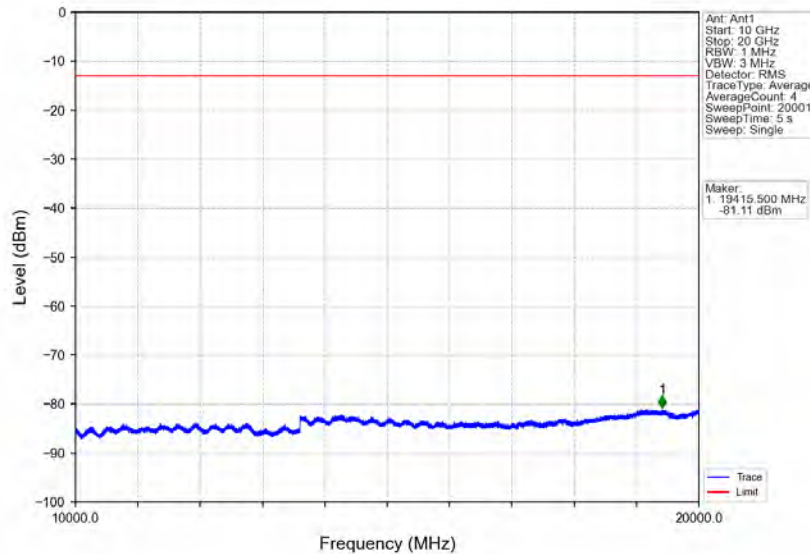
Band2_10MHz_16QAM_HCH_1905MHz_RB_1_0_NTNV
