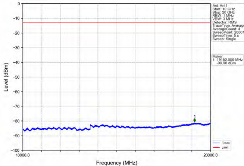
Band2_3MHz_QPSK_MCH_1880MHz_RB_1_0_NTNV
