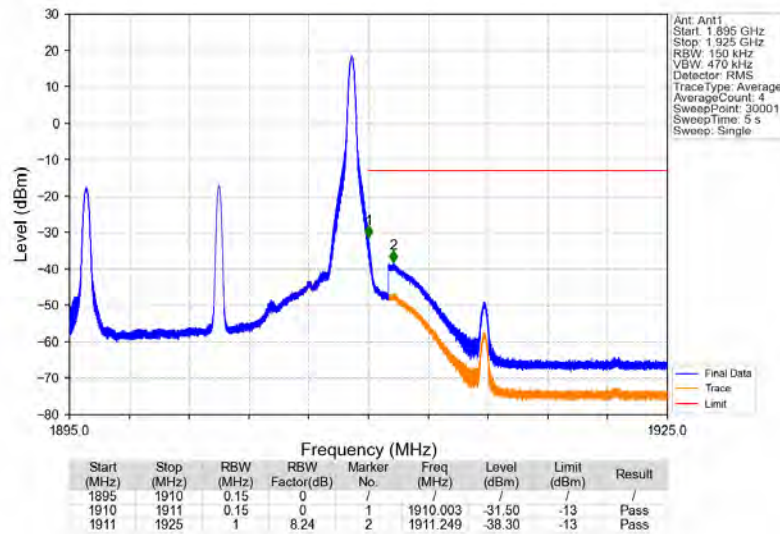
Band2_15MHz_QPSK_HCH_1902.5MHz_RB_1_74_NTNV
