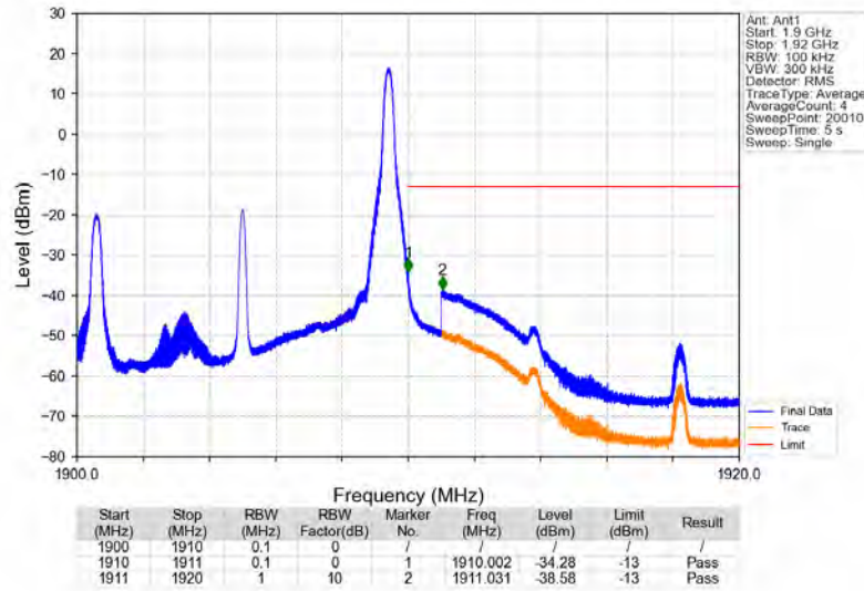
Band2_10MHz_16QAM_HCH_1905MHz_RB_1_49_NTV
