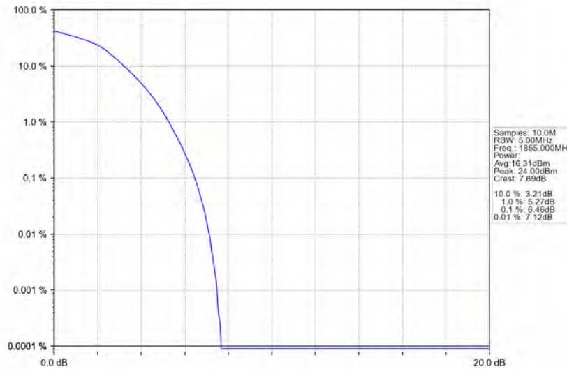
Band2_10MHz_16QAM_LCH_1855MHz_RB_50_0_NTNV
