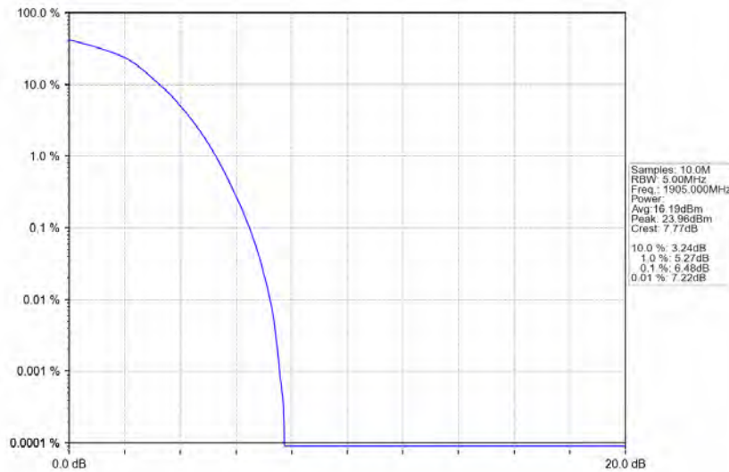
Band2_10MHz_16QAM_HCH_1905MHz_RB_50_0_NTNV
