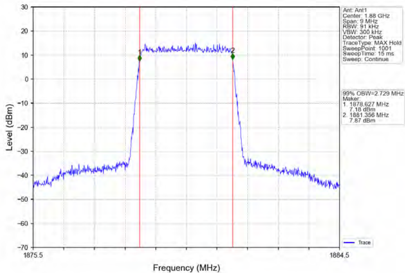
Band2_3MHz_QPSK_MCH_1880MHz_RB_15_0_NTNV
