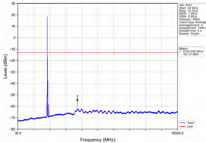
Band2_20MHz_16QAM_MCH_1880MHz_RB_1_0_NTNV
