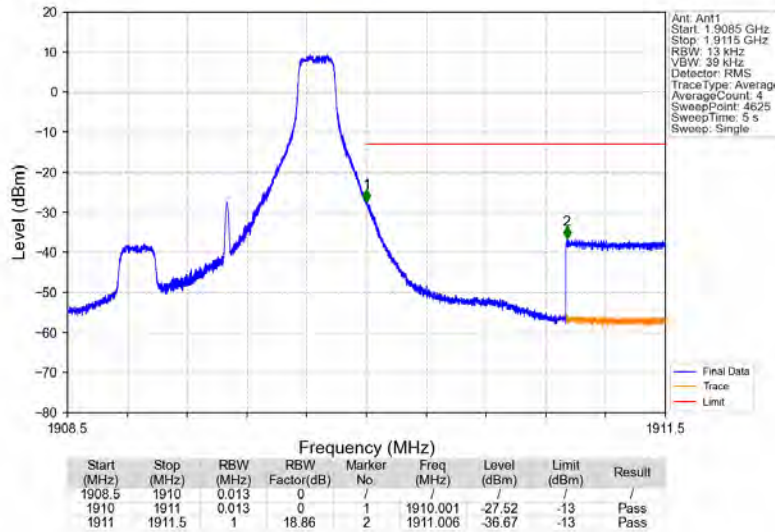
Band2_1.4MHz_QPSK_HCH_1909.3MHz_RB_1_5_NTV
