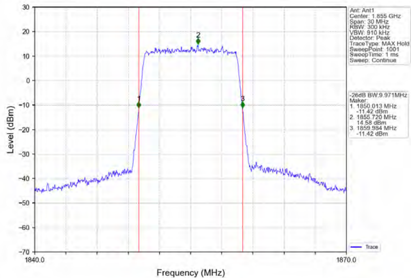
Band2_10MHz_16QAM_LCH_1855MHz_RB_50_0_NTNV
