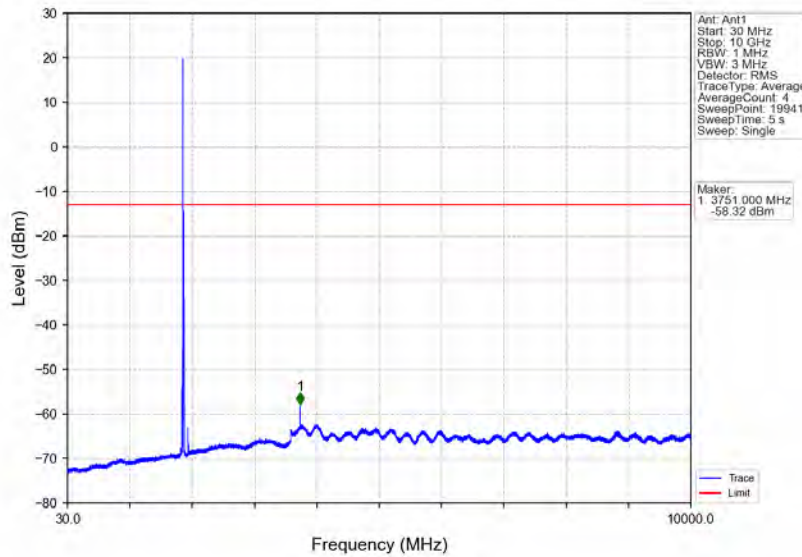
Band2_10MHz_QPSK_MCH_1880MHz_RB_1_0_NTNV
