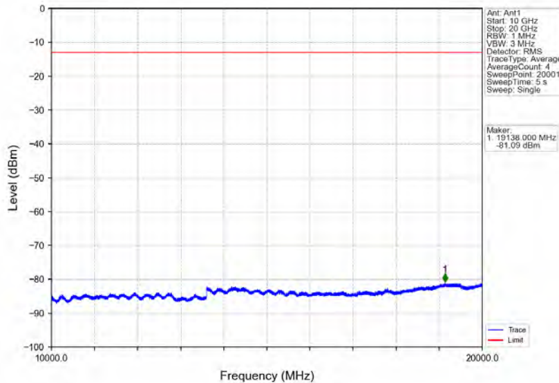
Band2_5MHz_QPSK_MCH_1880MHz_RB_1_0_NTNV
