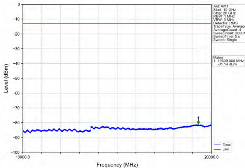
Band2_20MHz_16QAM_MCH_1880MHz_RB_1_0_NTNV
