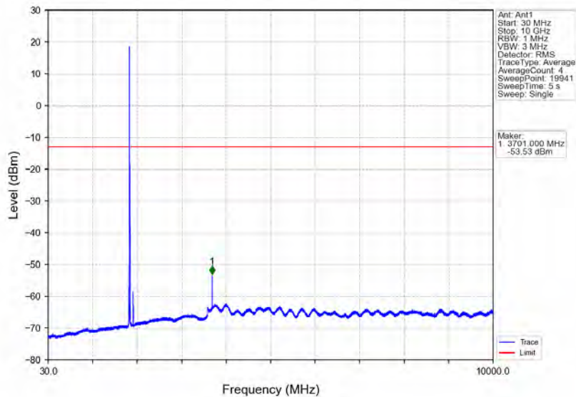
Band2_10MHz_16QAM_LCH_1855MHz_RB_1_0_NTV
