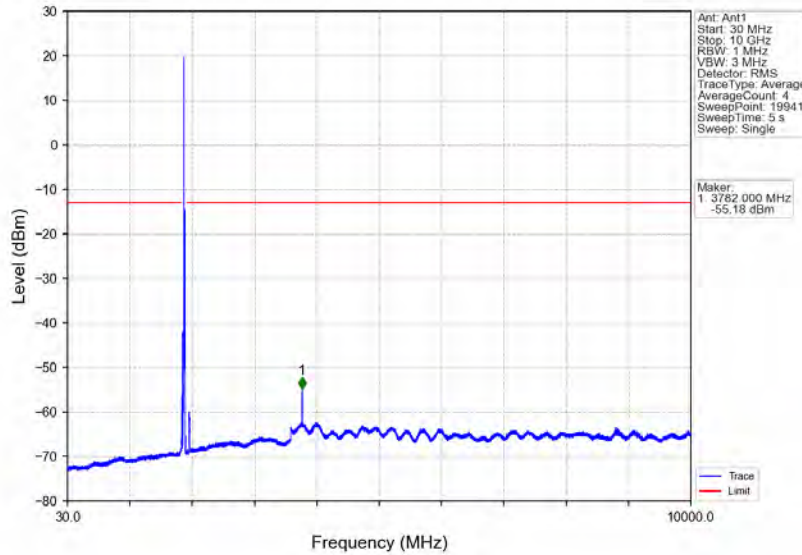
Band2_20MHz_QPSK_HCH_1900MHz_RB_1_0_NTNV
