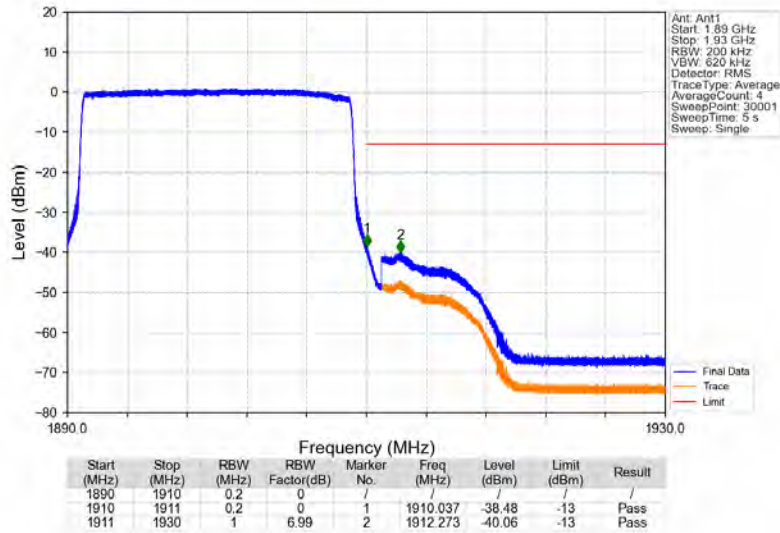
Band2_20MHz_QPSK_HCH_1900MHz_RB_100_0_NTNV
