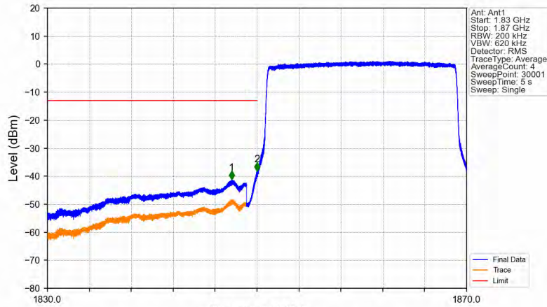
Band2_20MHz_QPSK_LCH_1860MHz_RB_100_0_NTNV
