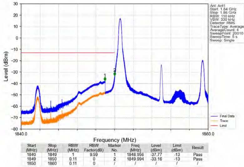
Band2_10MHz_16QAM_LCH_1855MHz_RB_1_0_NTV
