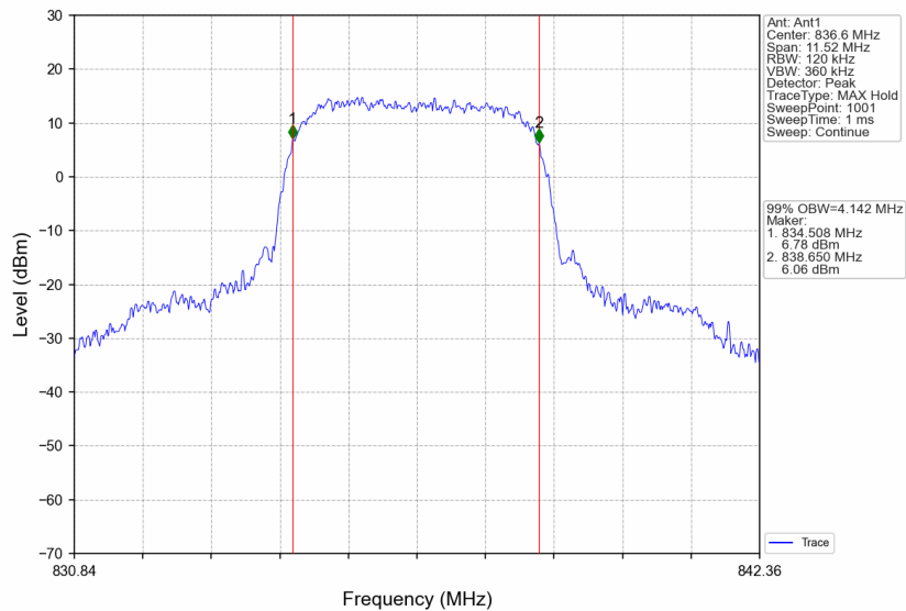
Band5_HSUPA_MCH_836.6MHz_Subtest 1_NTNV
