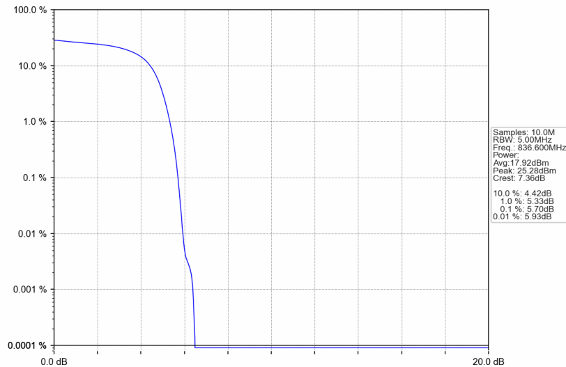
Band5_HSUPA_MCH_836.6MHz_Subtest 1_NTNV
