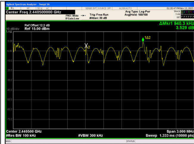
π/4DQPSK
