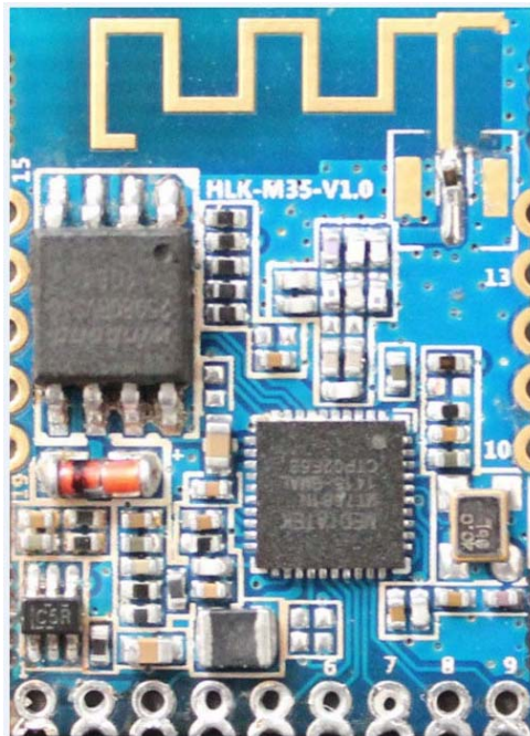
HLK-M35 top
