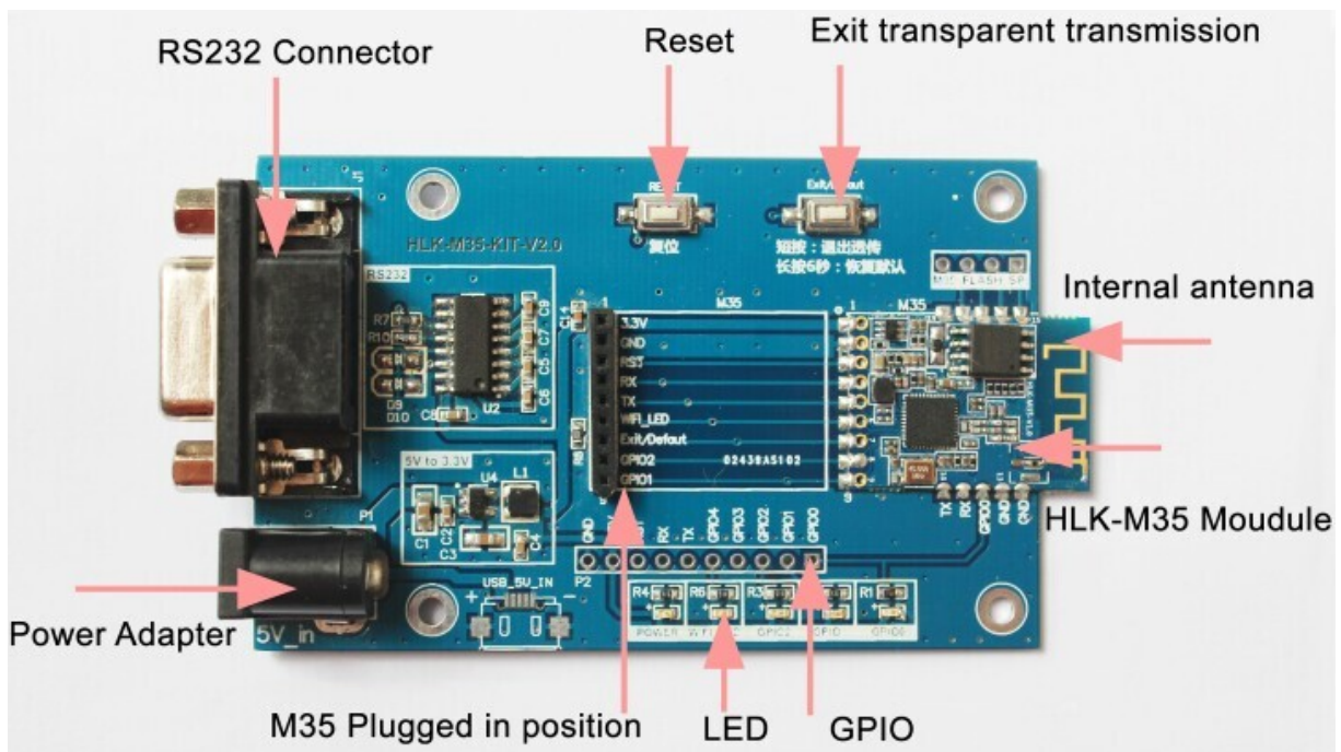
HLK-M35 StartKit
