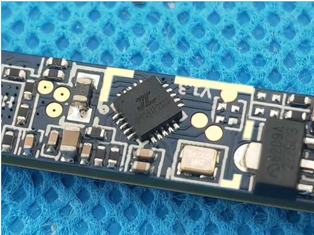
BLE Chip
