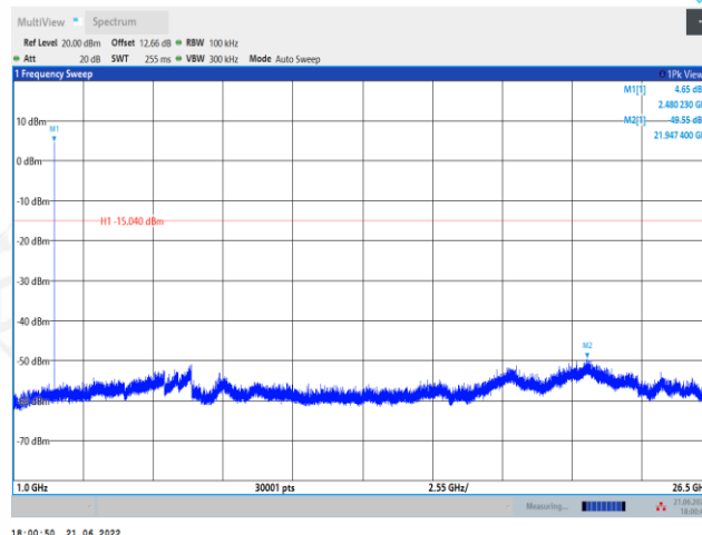
3DH5 Ant1 2480 1000~26500
