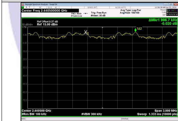
8DPSK
