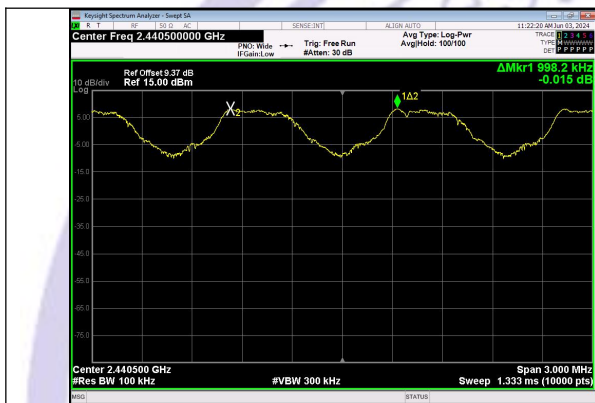
GFSK
