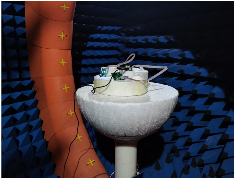
有源测试
