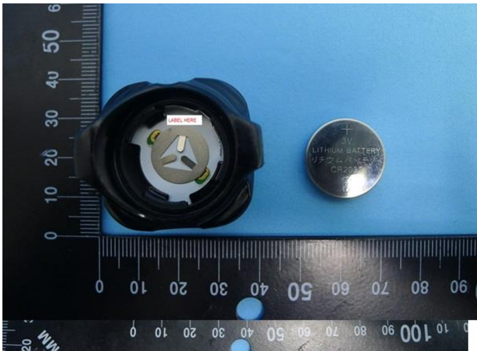
(4) EUT Photo
