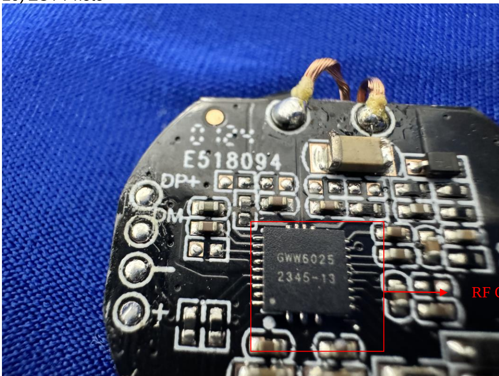
20) EUT Photo
