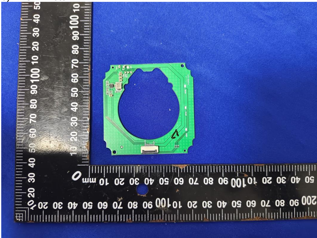
8) EUT Photo
