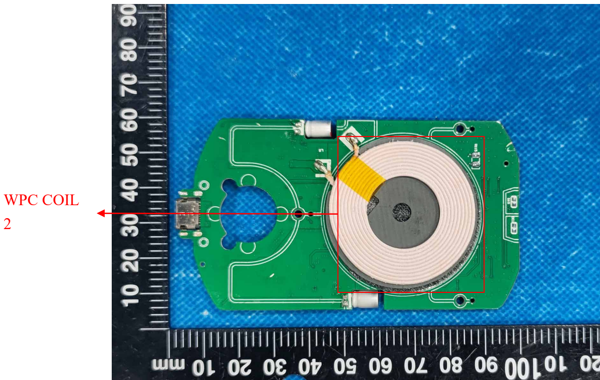
4) EUT Photo
