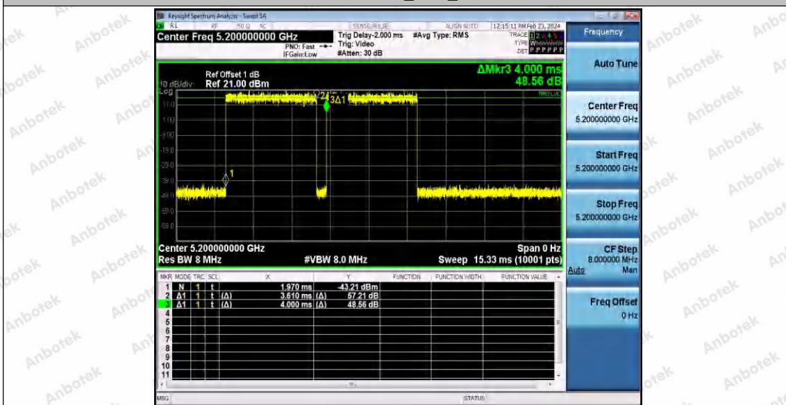
11AX20MIMO_Ant2_5200
