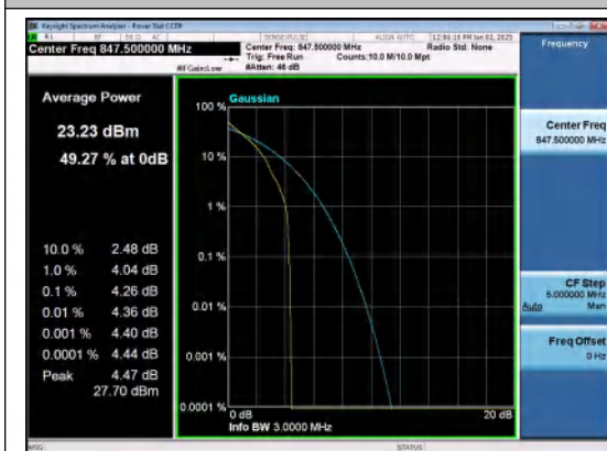
Band26(824-849)-3MHz-QPSK-27025-1RB#0-PA
