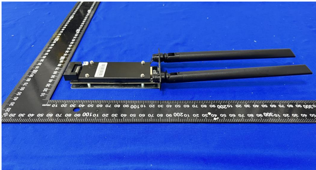
6) EUT Photo
