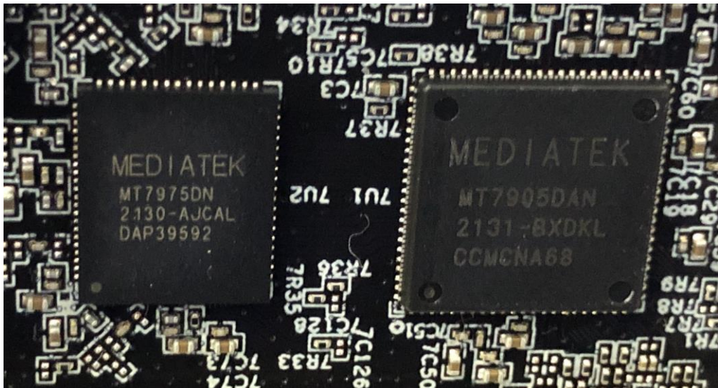
6) EUT Photo
