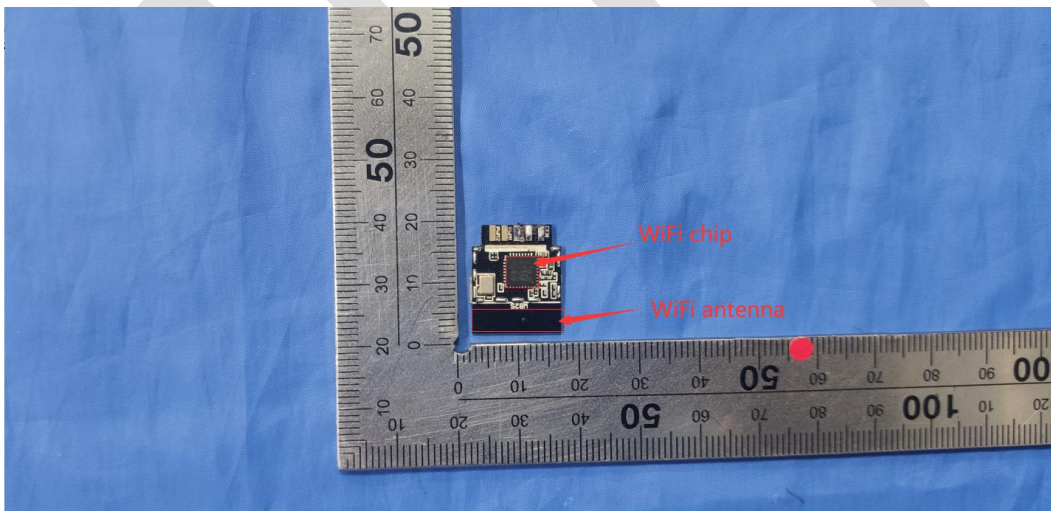
WI-FI module
