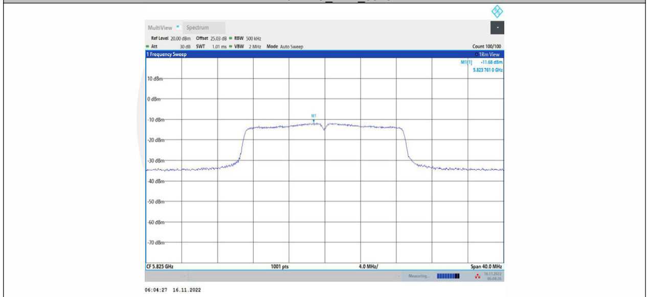
11N20MIMO_Ant2_5825
