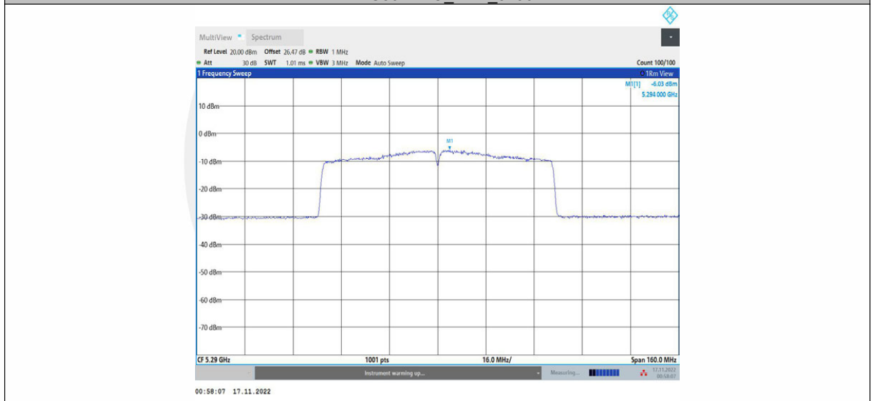
11AC80MIMO_Ant2_5290
