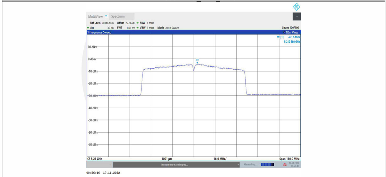
11AC80MIMO_Ant2_5210
