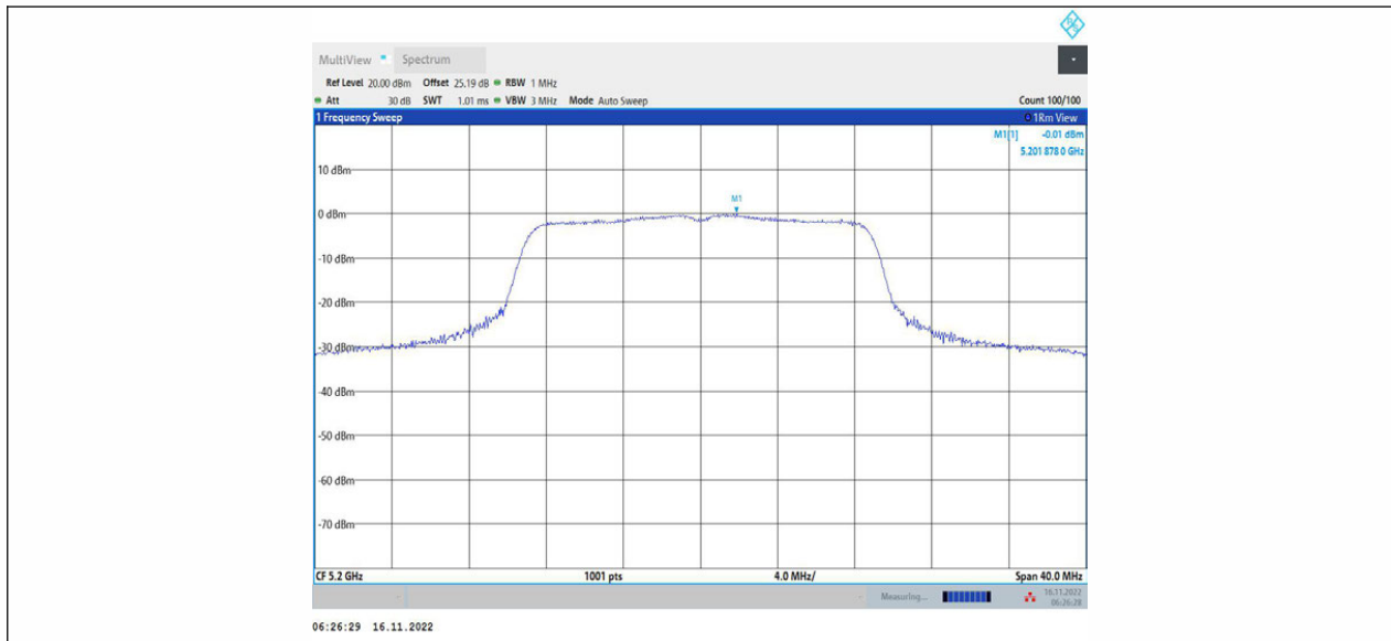
11AC20MIMO_Ant1_5200
