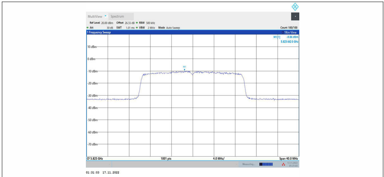
11AX20MIMO_Ant1_5825
