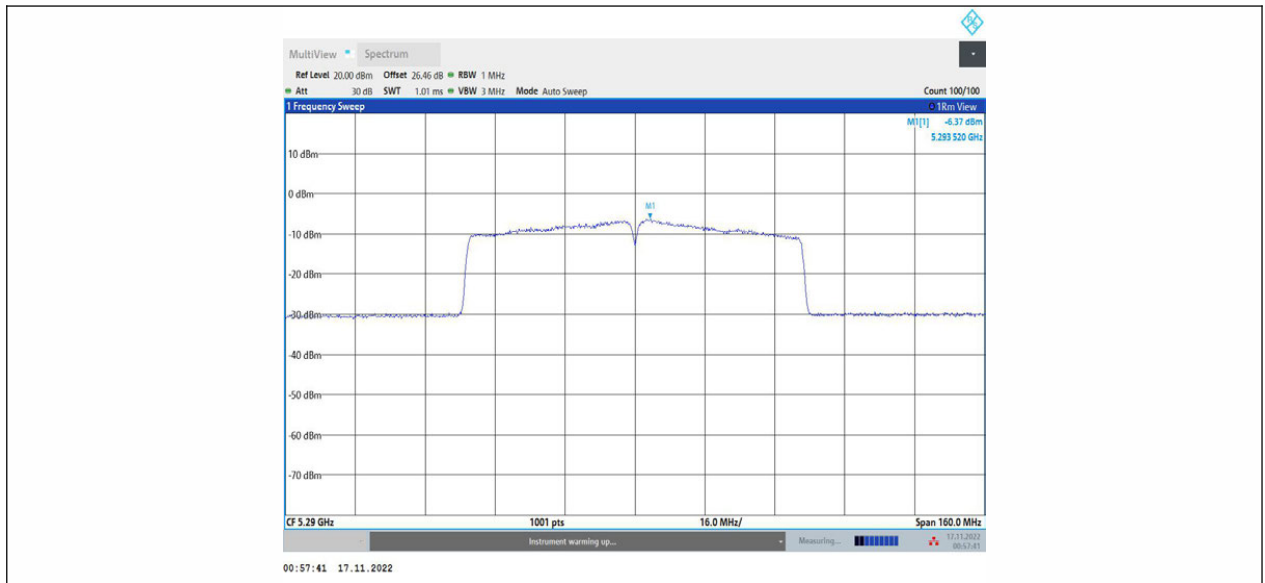
11AC80MIMO_Ant1_5290
