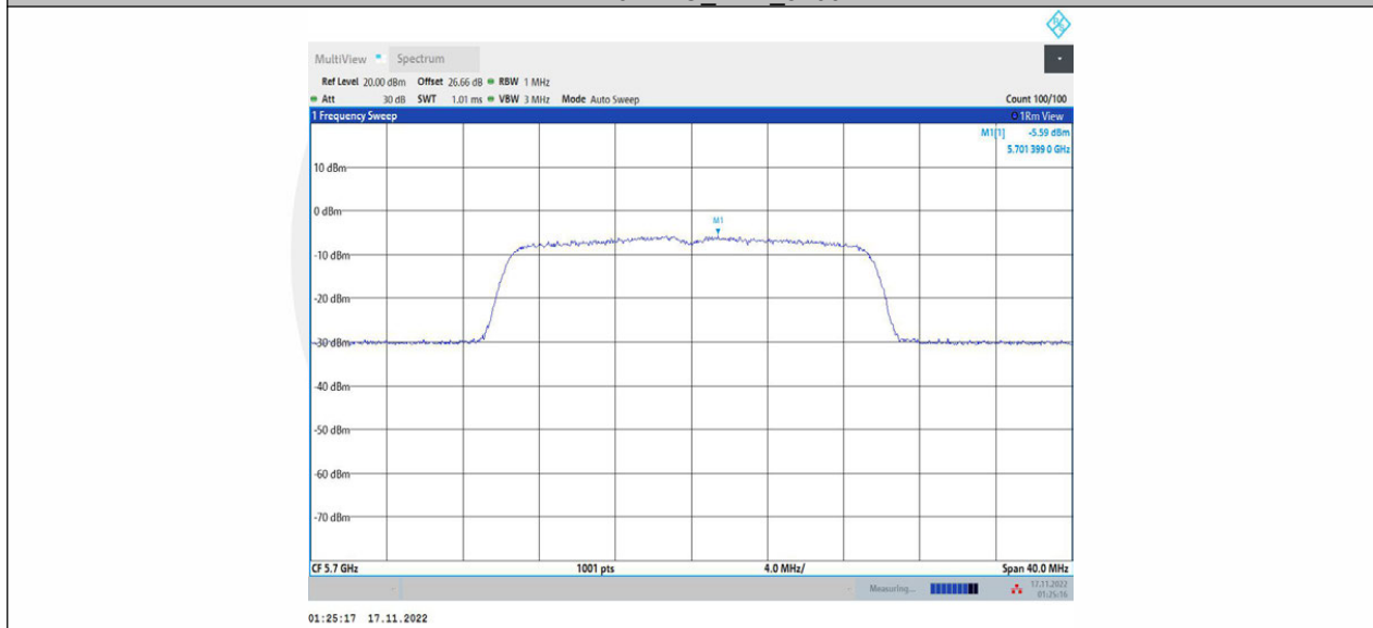
11AX20MIMO_Ant2_5700
