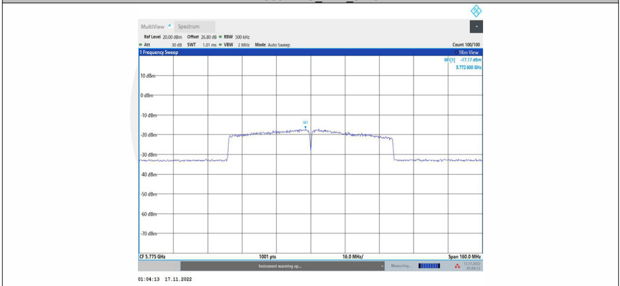
11AC80MIMO_Ant2_5775
