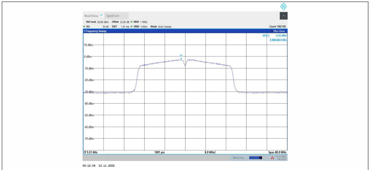
11N40MIMO_Ant1_5310
