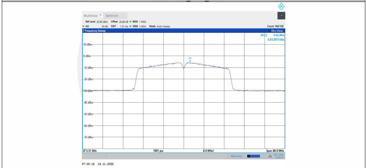
11AC40MIMO_Ant2_5510
