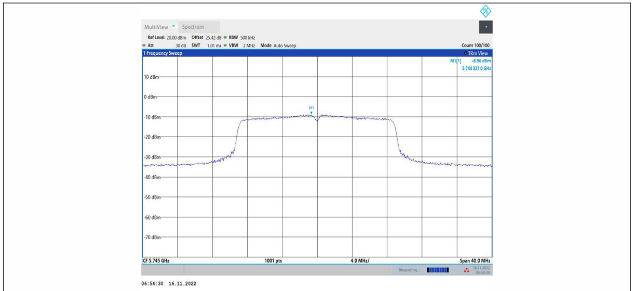
11AC20MIMO_Ant1_5745
