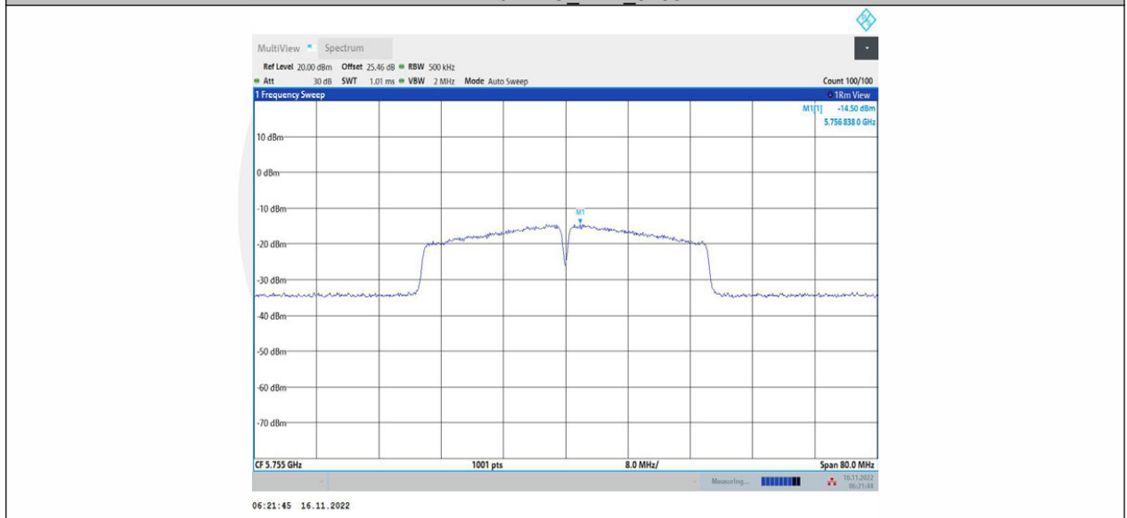
11N40MIMO_Ant2_5755
