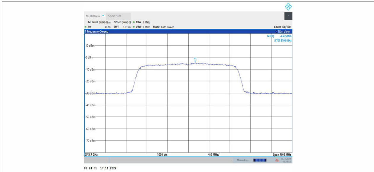
11AX20MIMO_Ant1_5700
