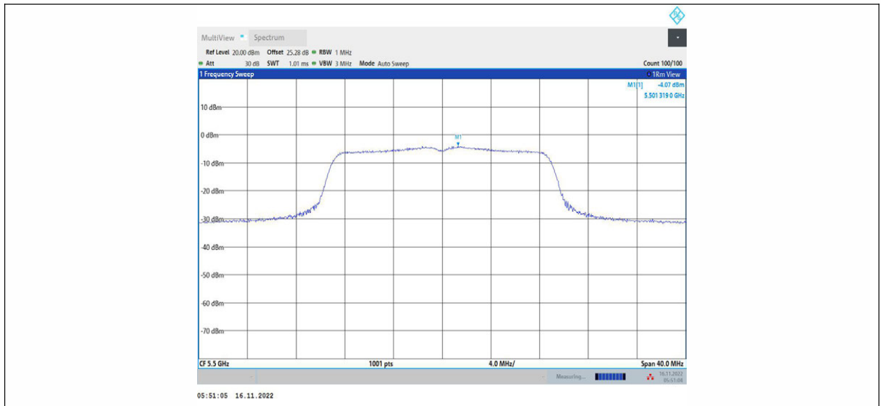
11N20MIMO_Ant1_5500
