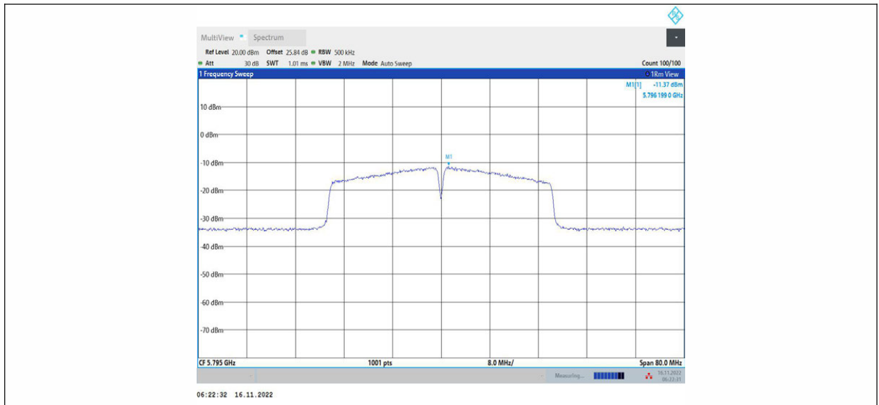
11N40MIMO_Ant1_5795
