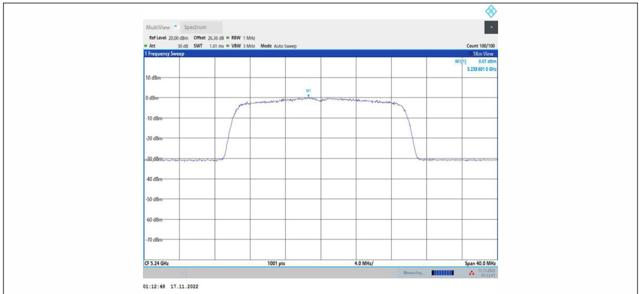
11AX20MIMO_Ant1_5240
