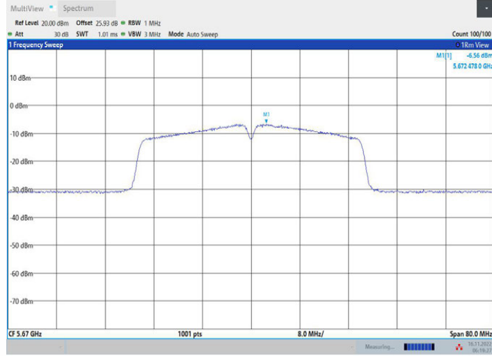
11N40MIMO_Ant1_5670
