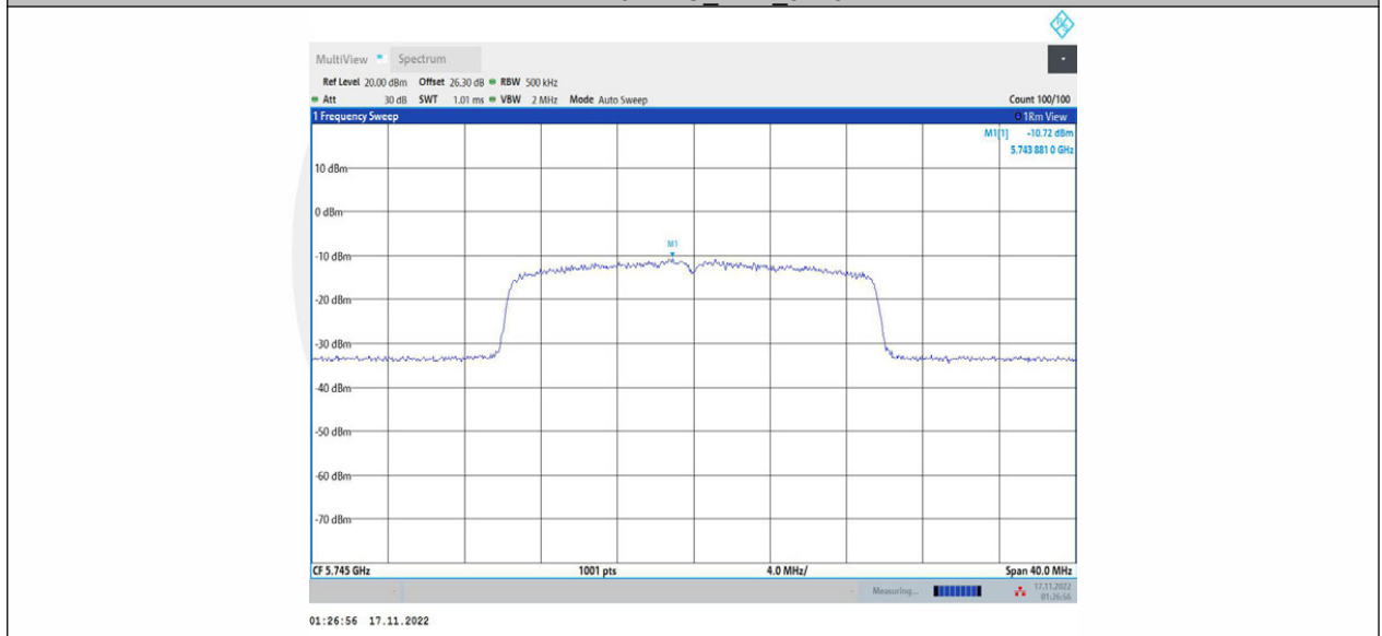
11AX20MIMO_Ant2_5745
