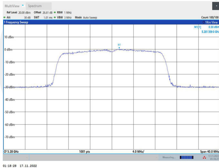
11AX20MIMO_Ant2_5280
