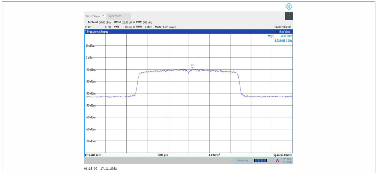
11AX20MIMO_Ant1_5785
