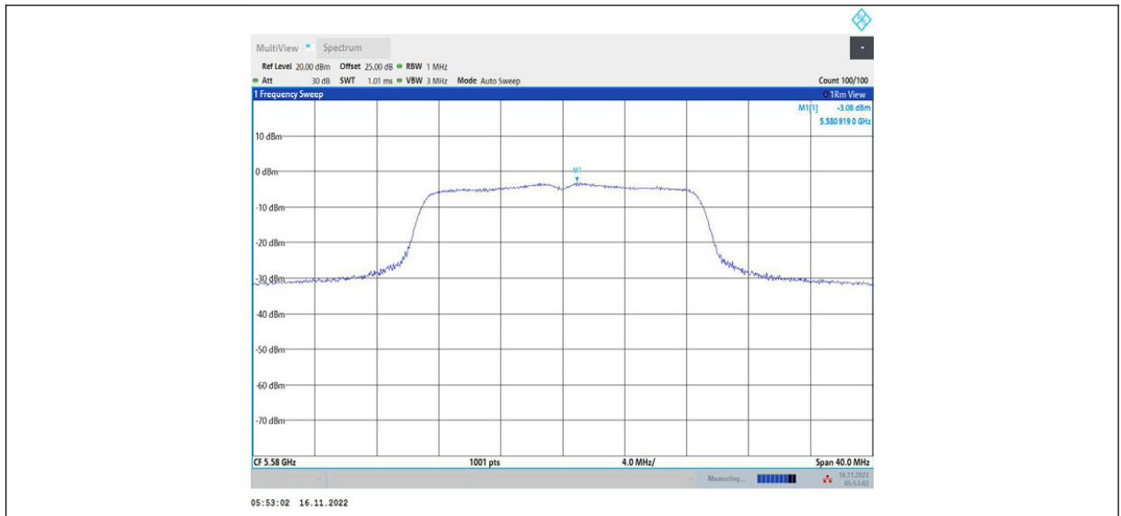
11N20MIMO_Ant1_5580
