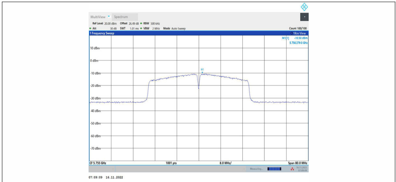
11AC40MIMO_Ant1_5755
