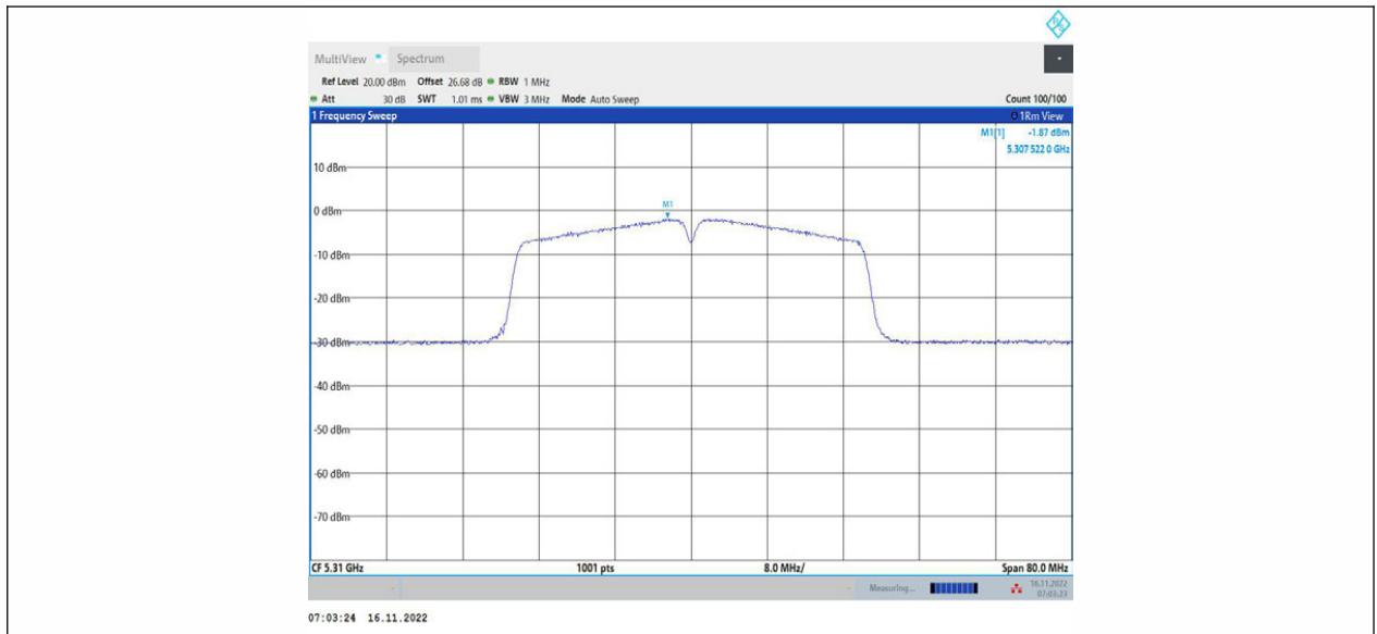
11AC40MIMO_Ant1_5310
