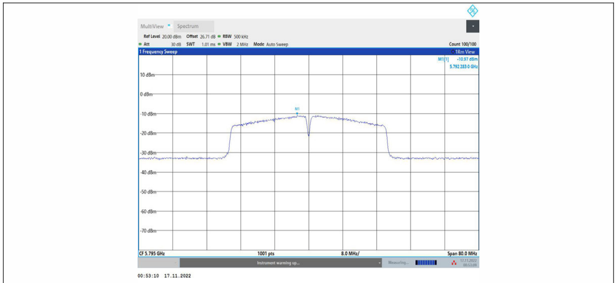
11AC40MIMO_Ant1_5795
