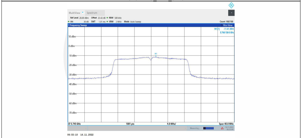
11AC20MIMO_Ant2_5745
