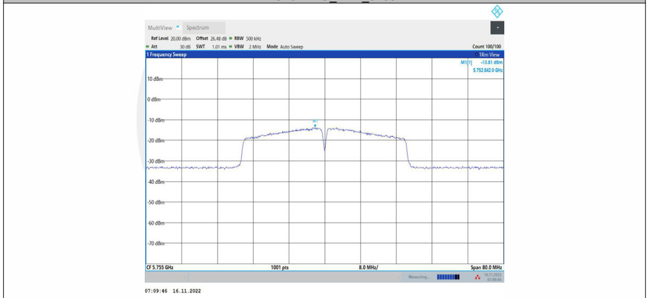
11AC40MIMO_Ant2_5755
