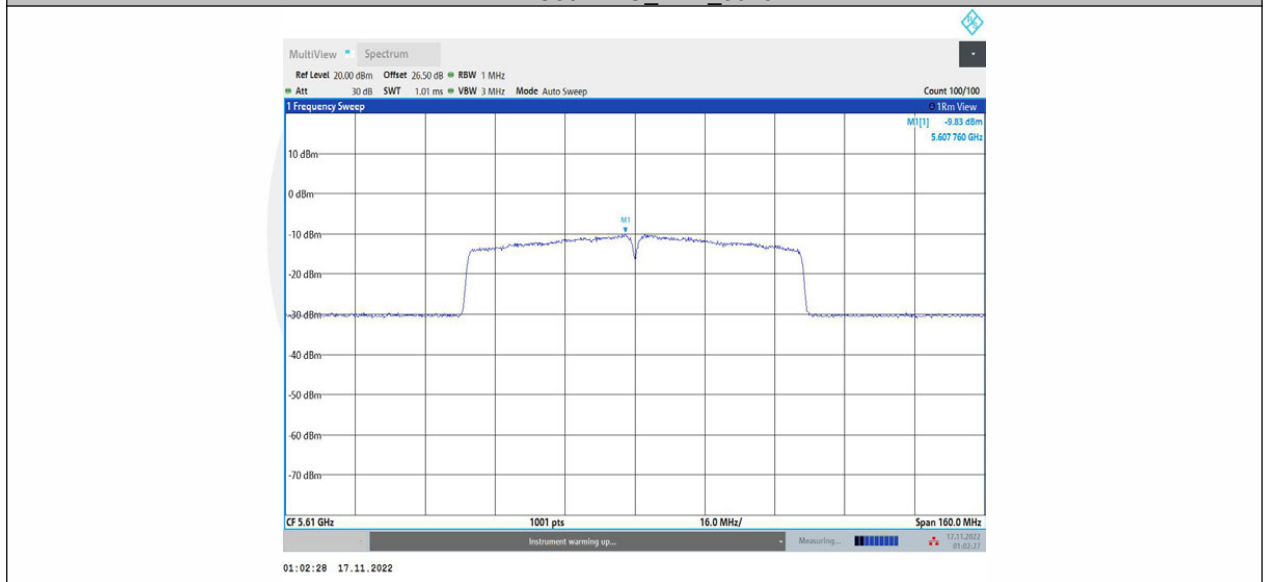
11AC80MIMO_Ant2_5610
