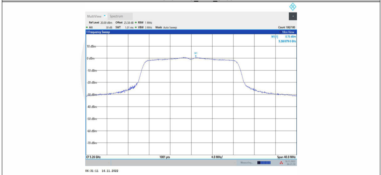
11AC20MIMO_Ant2_5260
