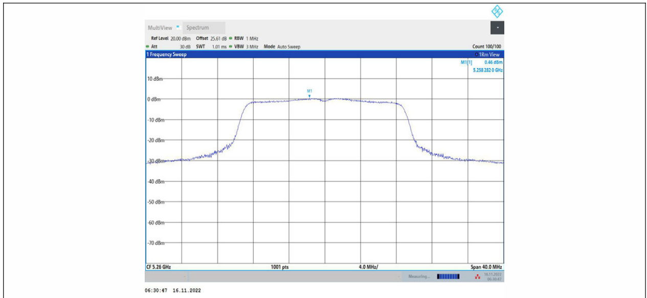
11AC20MIMO_Ant1_5260
