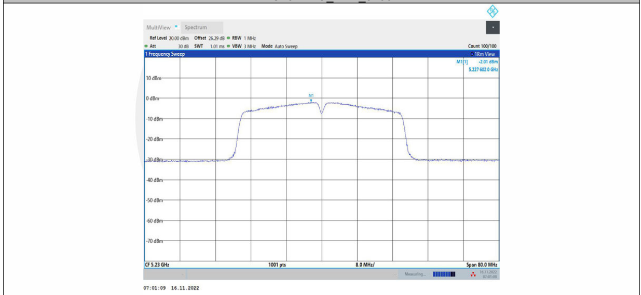
11AC40MIMO_Ant2_5230
