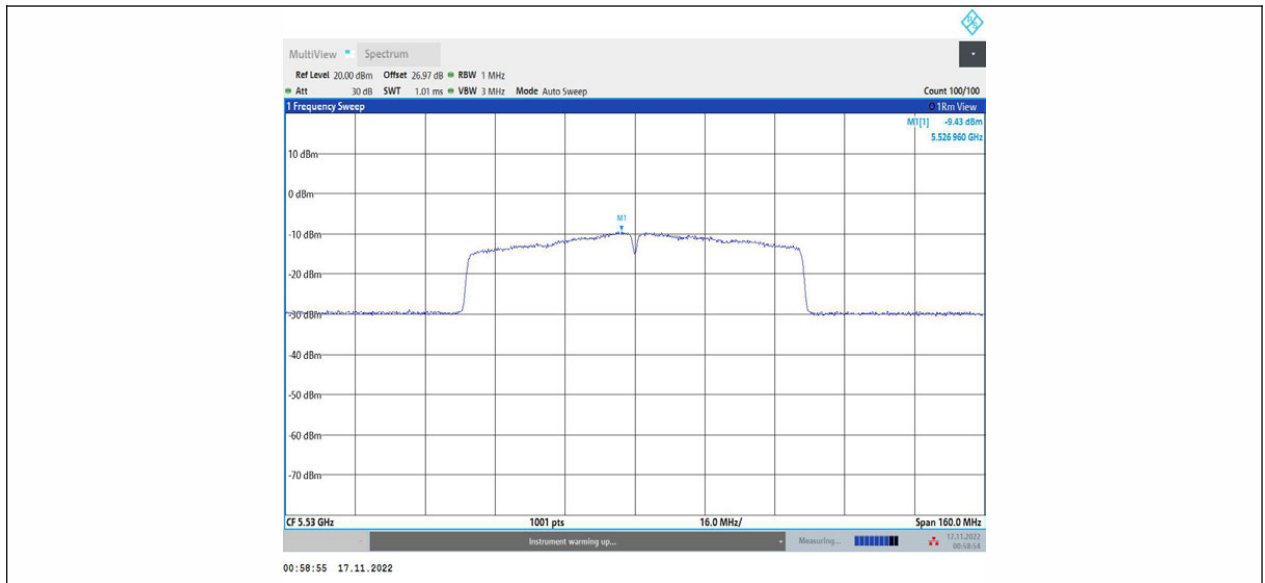
11AC80MIMO_Ant1_5530
