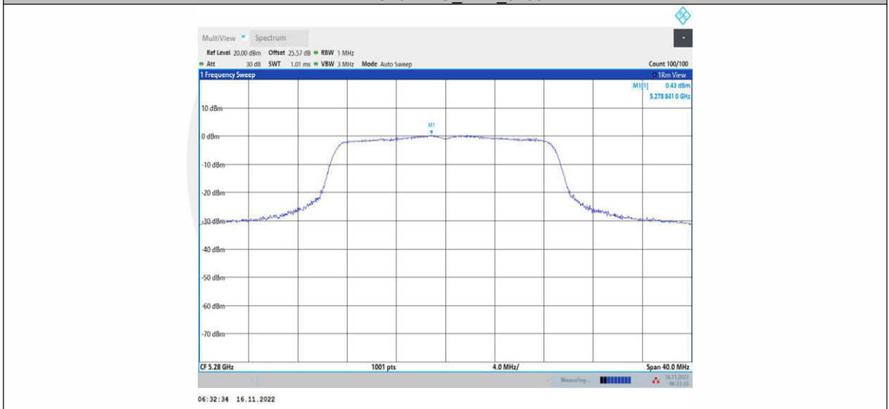
11AC20MIMO_Ant2_5280
