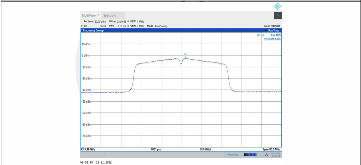
11N40MIMO_Ant2_5190
