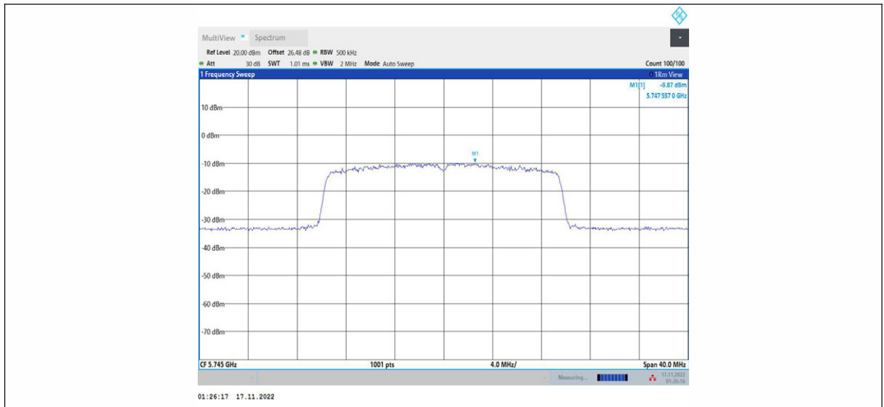
11AX20MIMO_Ant1_5745
