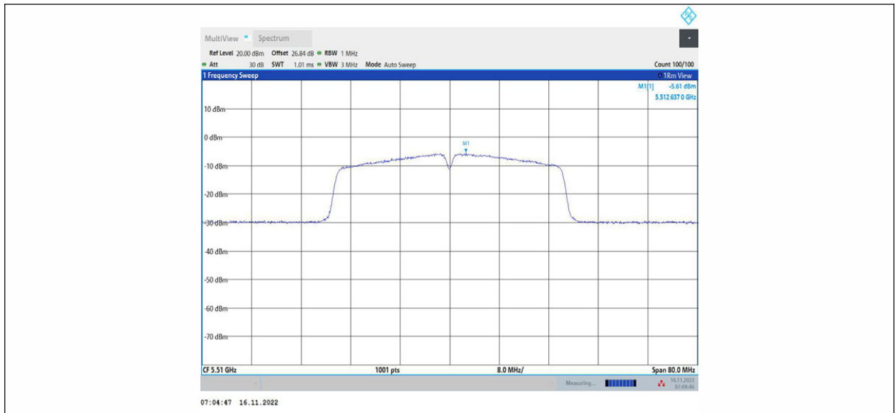
11AC40MIMO_Ant1_5510
