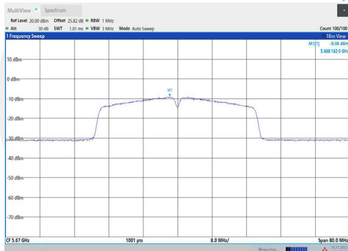
11N40MIMO_Ant2_5670
