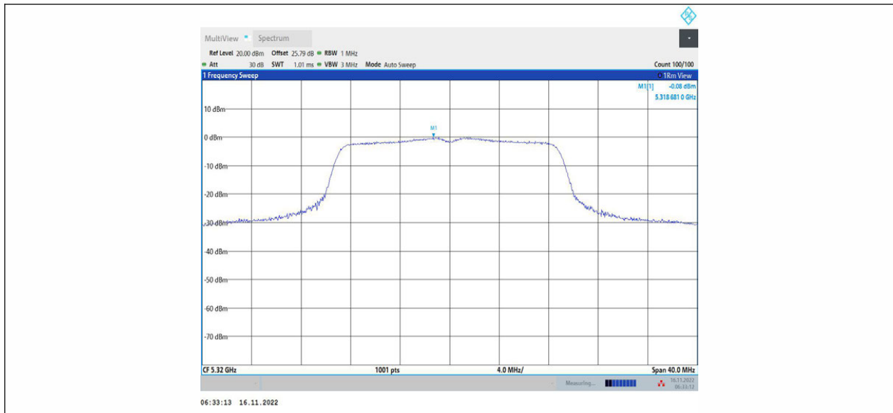
11AC20MIMO_Ant1_5320
