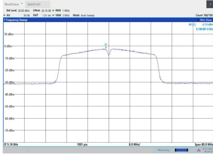
11AC40MIMO_Ant1_5190
