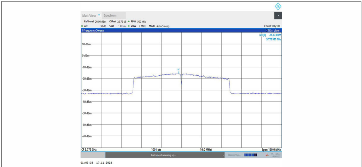
11AC80MIMO_Ant1_5775
