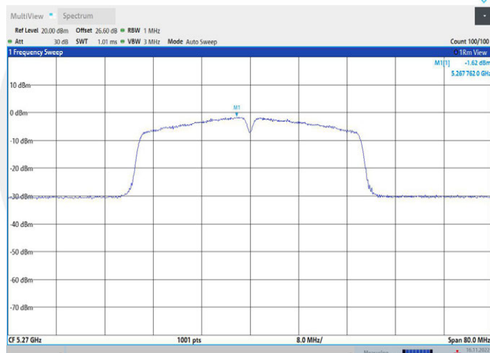
11AC40MIMO_Ant2_5270
