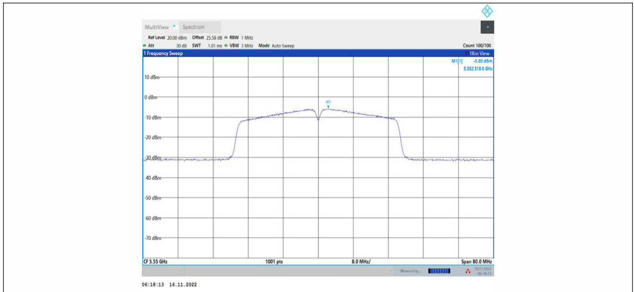
11N40MIMO_Ant1_5550
