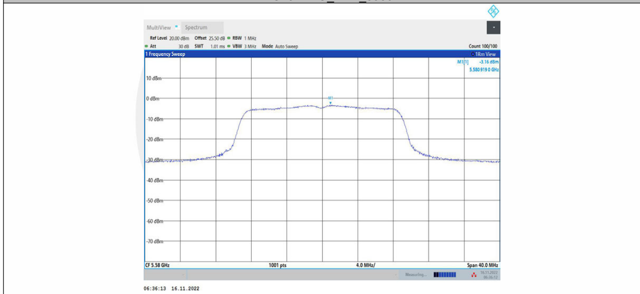
11AC20MIMO_Ant2_5580
