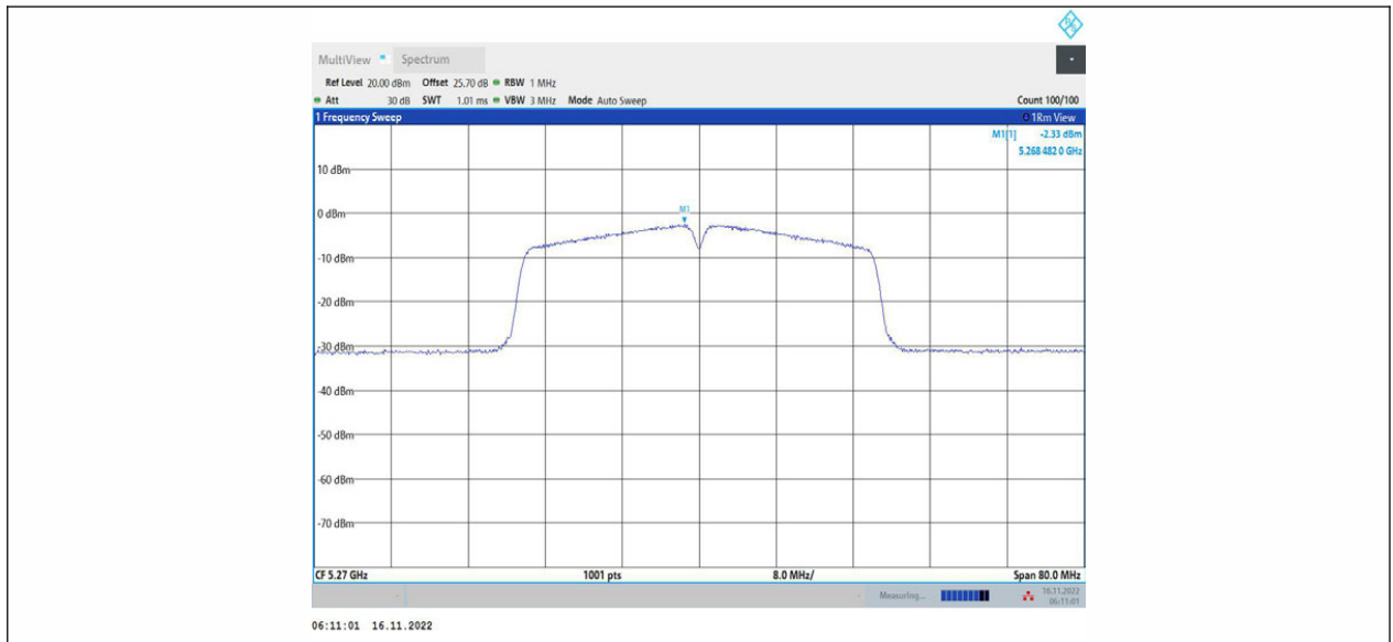
11N40MIMO_Ant1_5270
