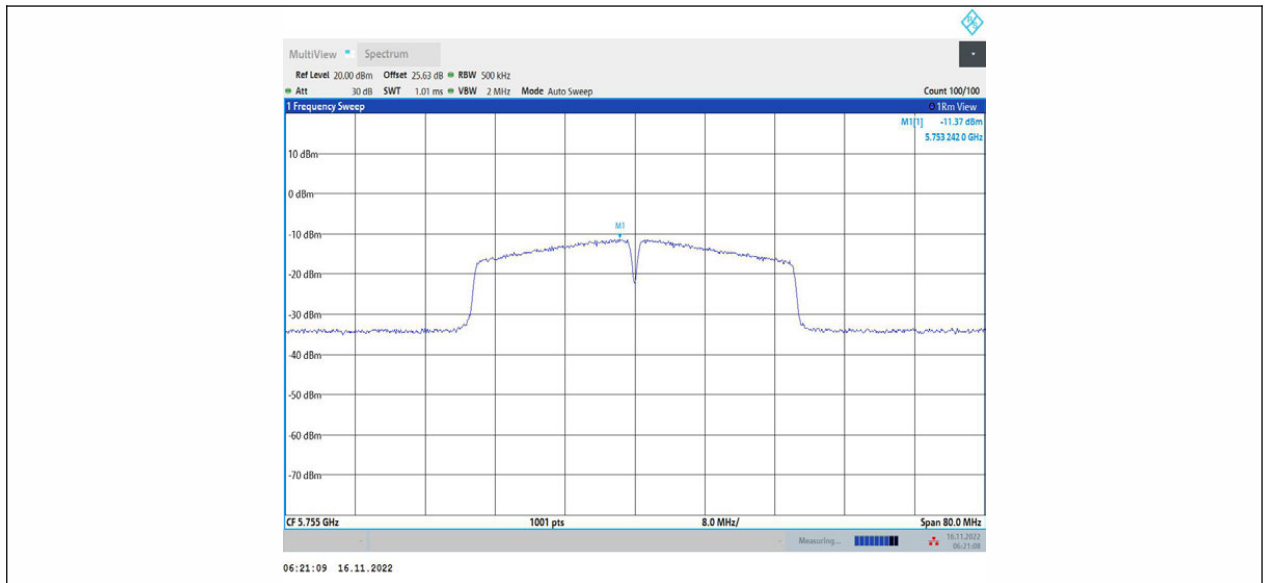
11N40MIMO_Ant1_5755
