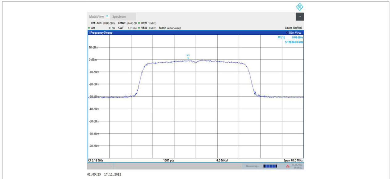
11AX20MIMO_Ant1_5180
