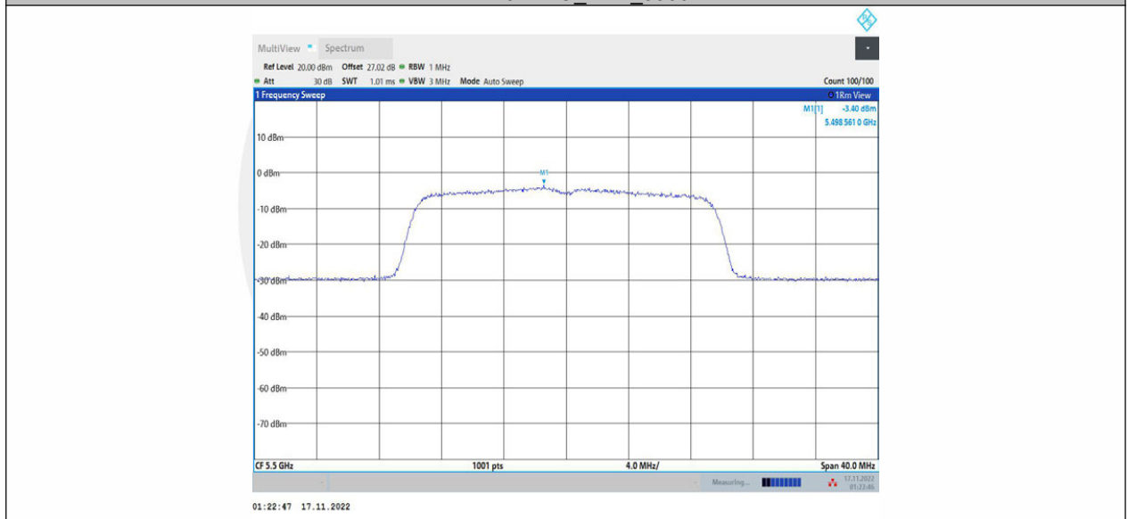
11AX20MIMO_Ant2_5500
