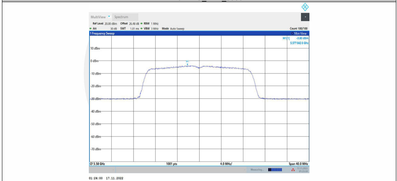
11AX20MIMO_Ant2_5580
