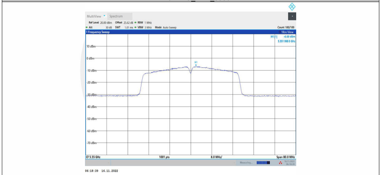
11N40MIMO_Ant2_5550
