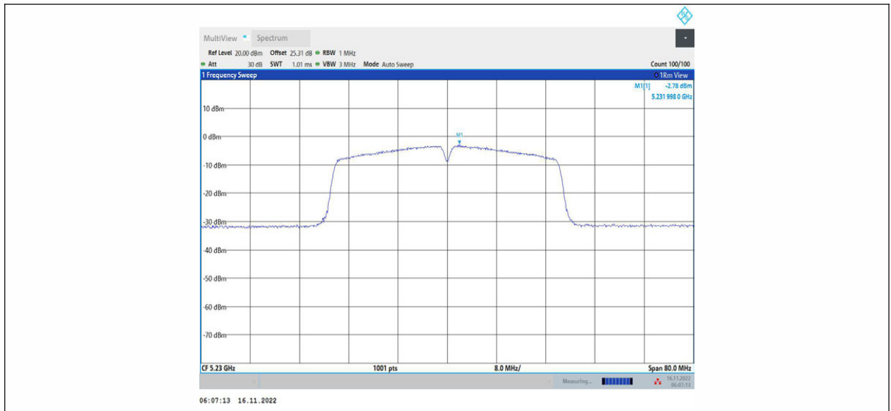
11N40MIMO_Ant1_5230
