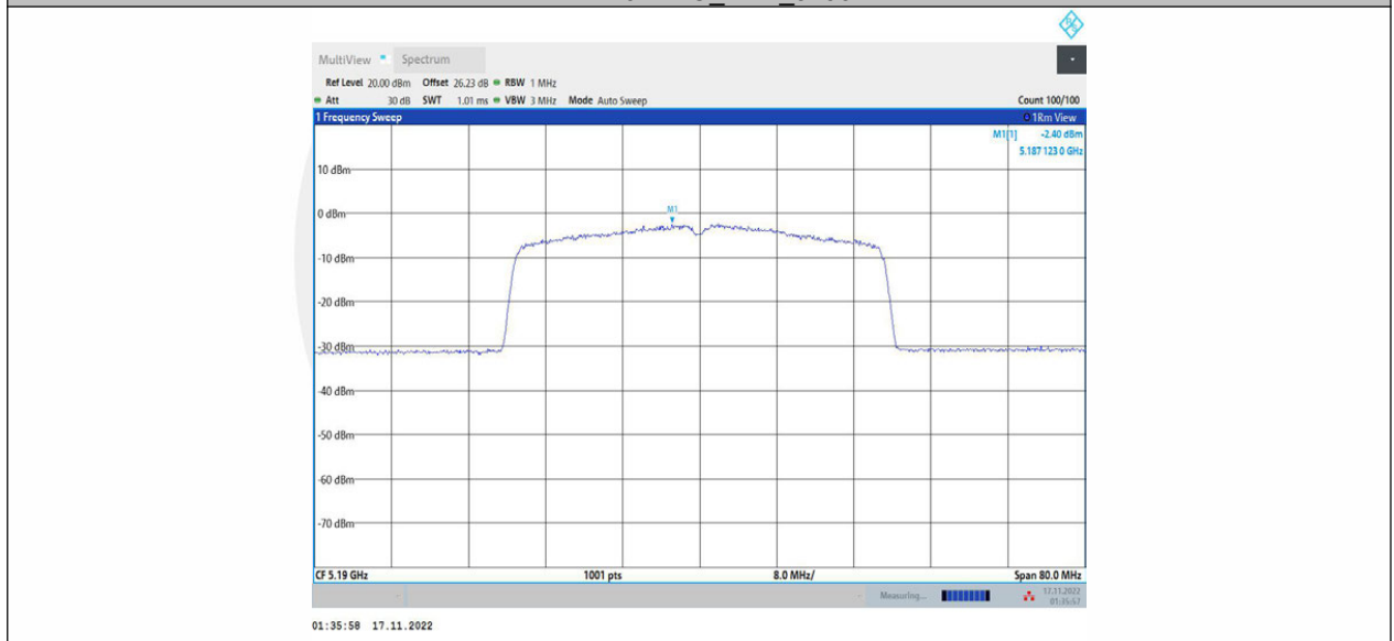
11AX40MIMO_Ant2_5190
