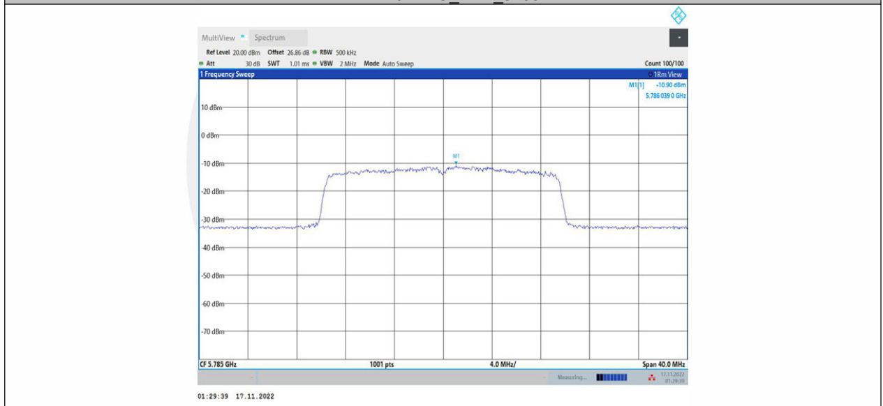
11AX20MIMO_Ant2_5785
