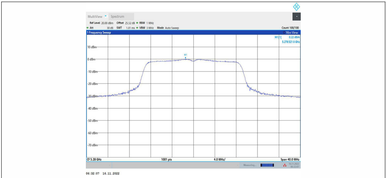
11AC20MIMO_Ant1_5280
