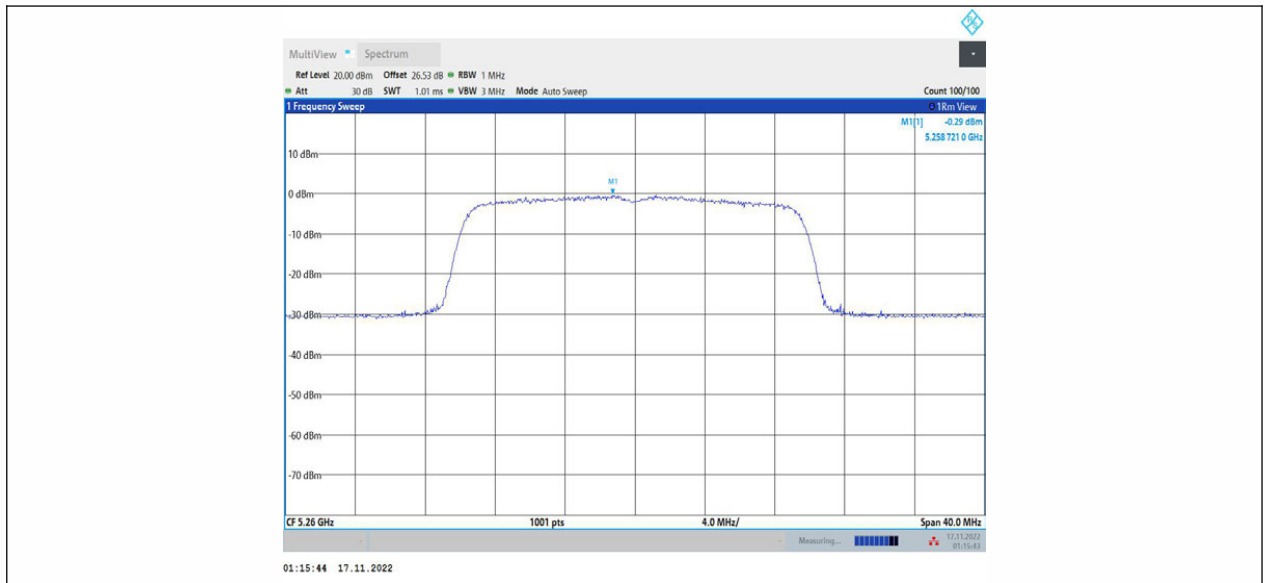
11AX20MIMO_Ant1_5260
