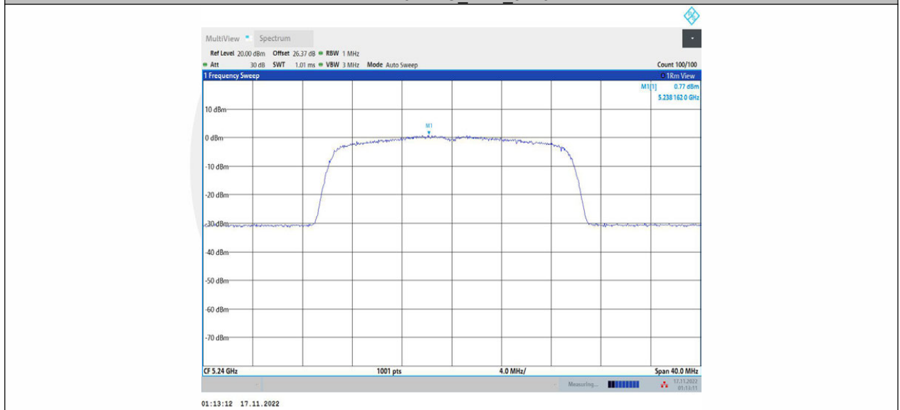
11AX20MIMO_Ant2_5240
