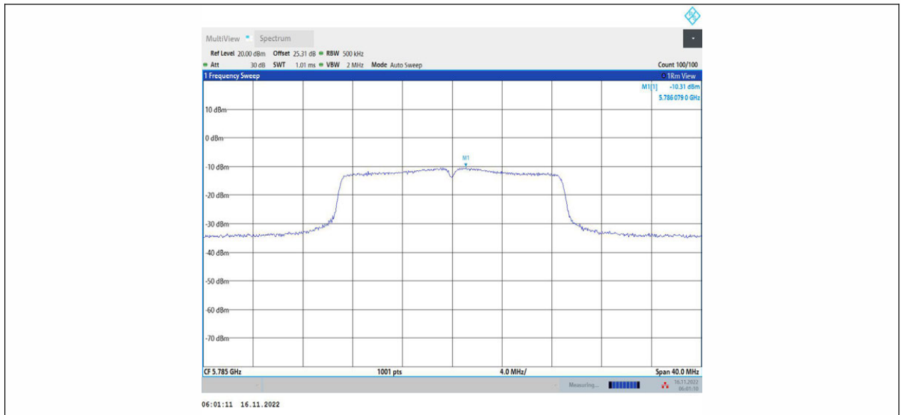
11N20MIMO_Ant1_5785
