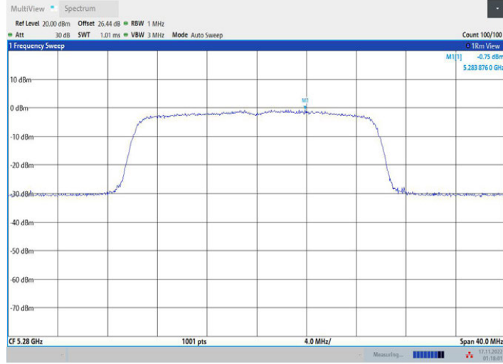
11AX20MIMO_Ant1_5280
