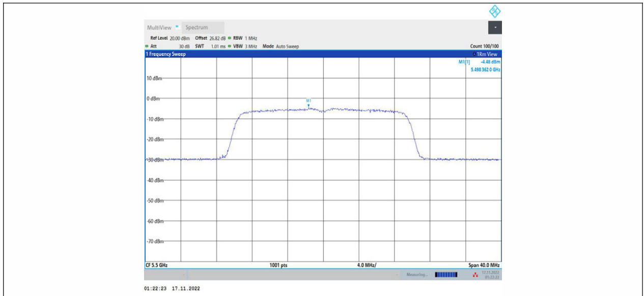
11AX20MIMO_Ant1_5500
