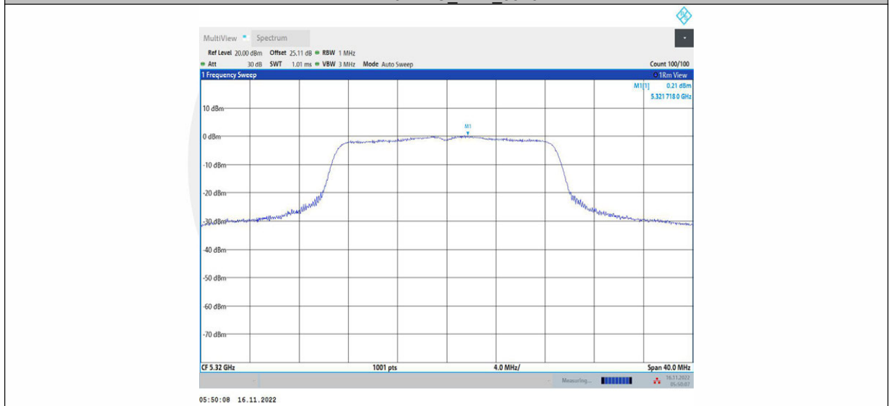
11N20MIMO_Ant2_5320
