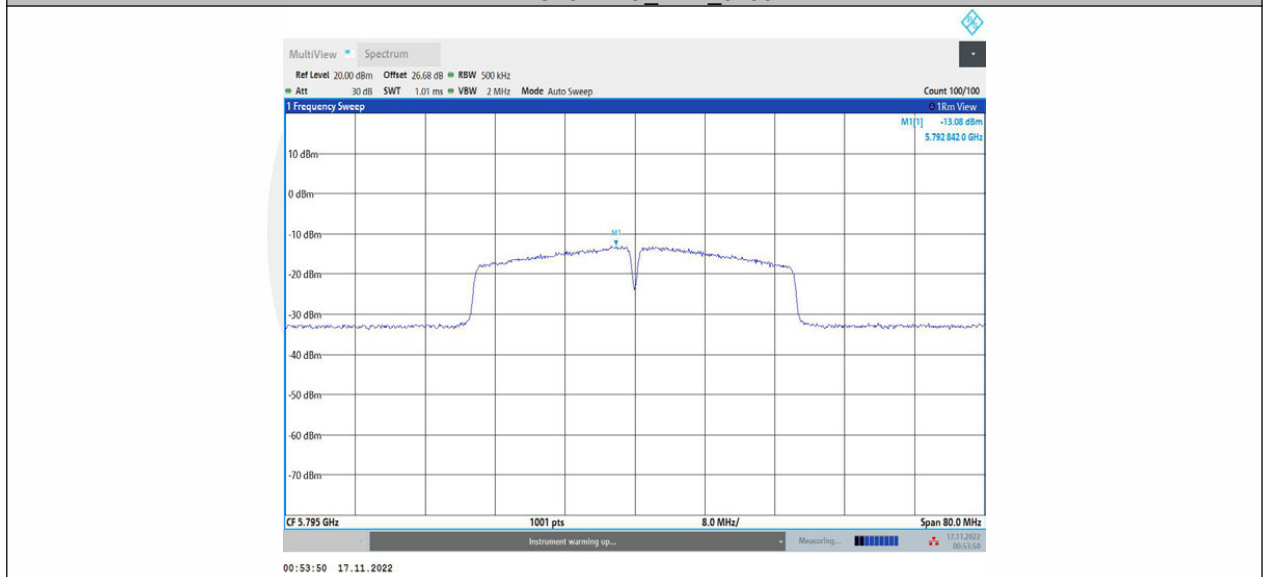
11AC40MIMO_Ant2_5795
