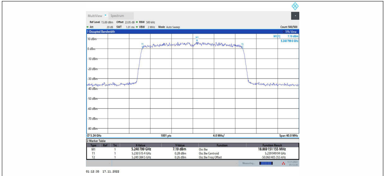
11AX20MIMO_Ant1_5240
