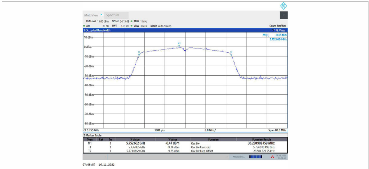
11AC40MIMO_Ant1_5755
