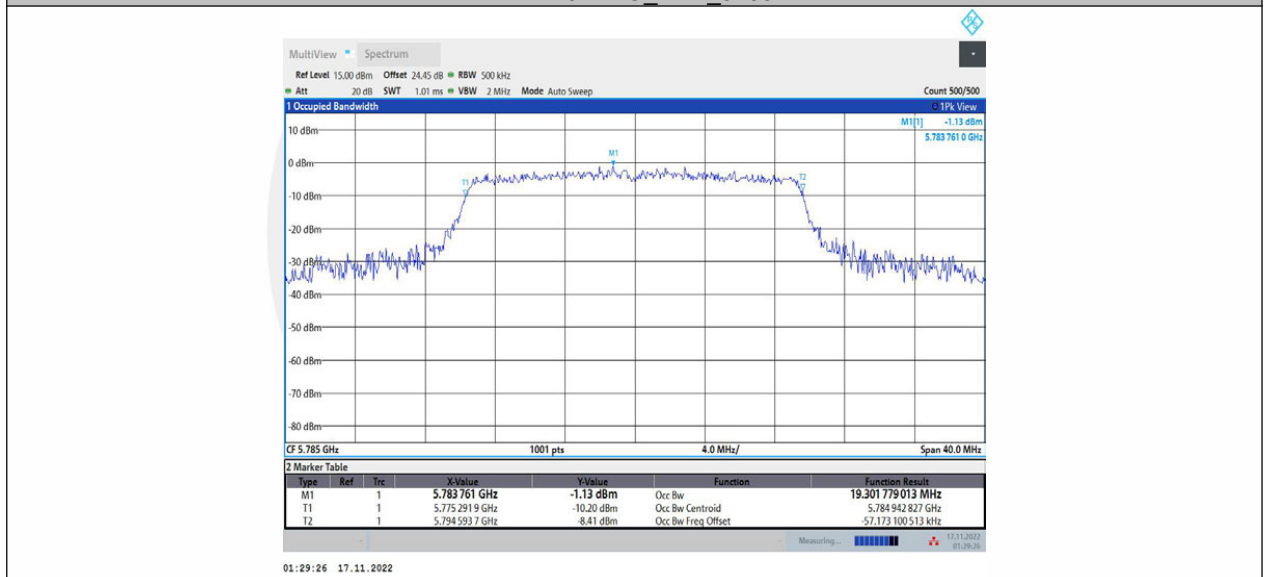
11AX20MIMO_Ant2_5785
