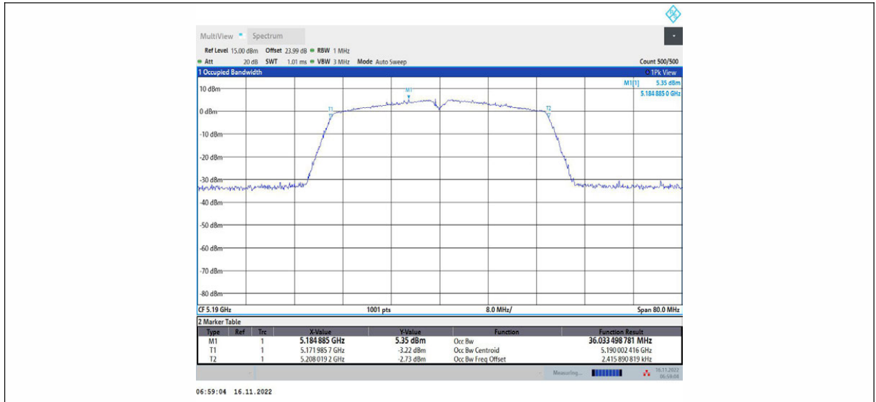
11AC40MIMO_Ant1_5190
