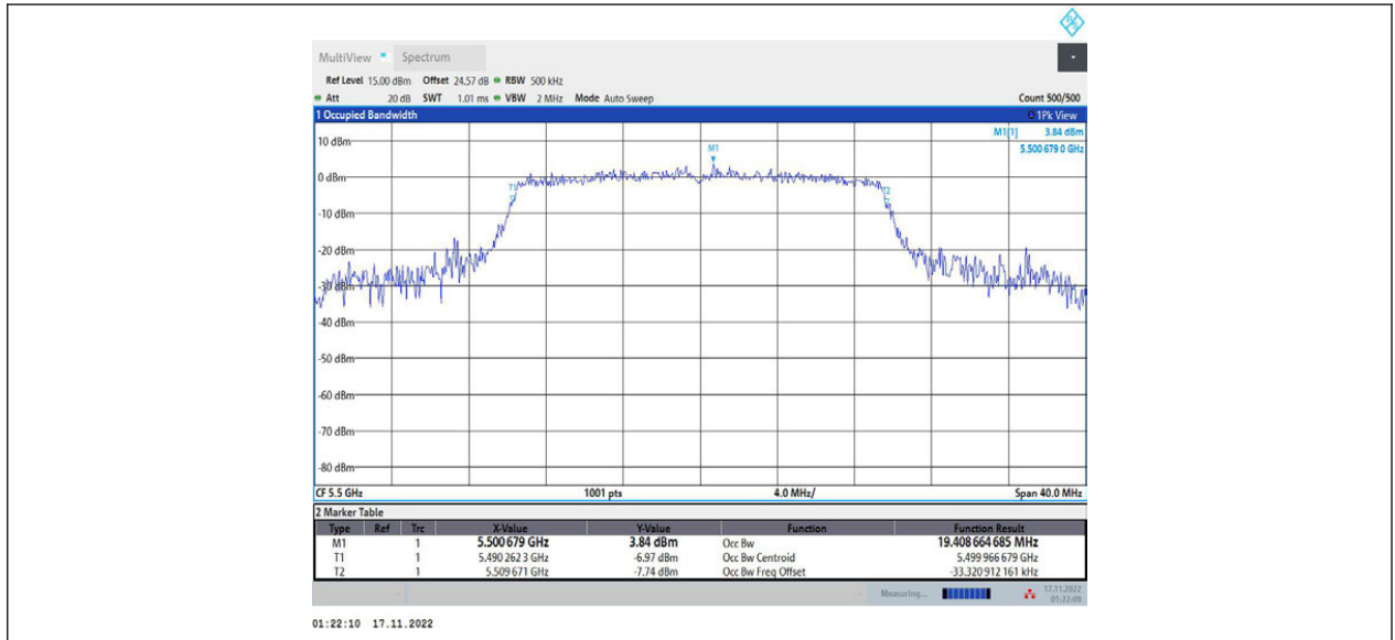
11AX20MIMO_Ant1_5500
