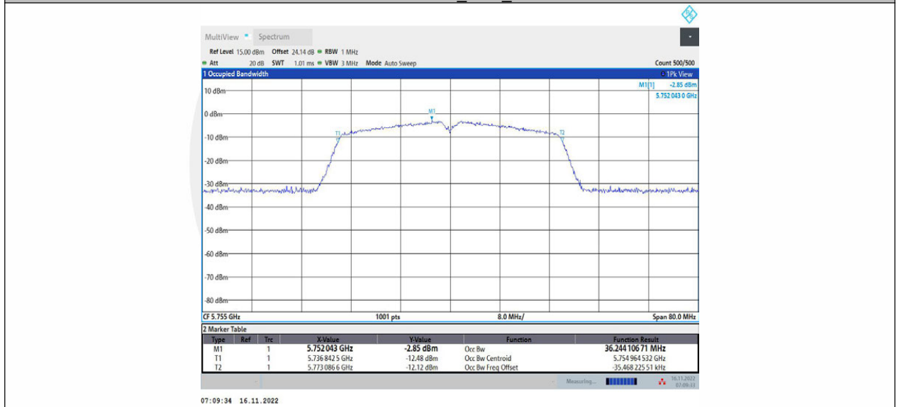
11AC40MIMO_Ant2_5755
