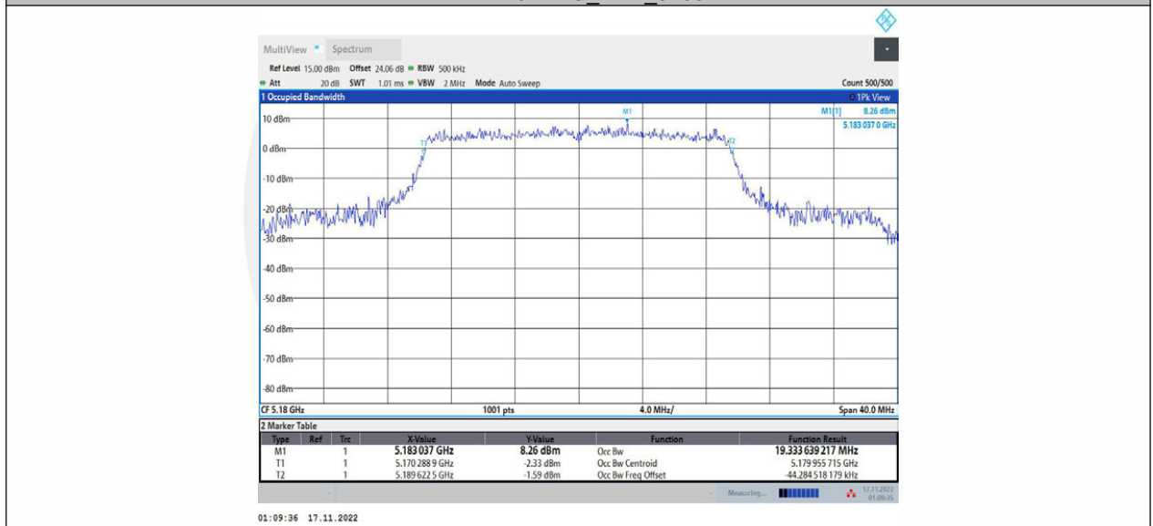
11AX20MIMO_Ant2_5180
