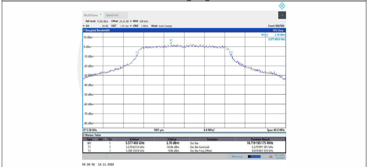
11AC20MIMO_Ant2_5580
