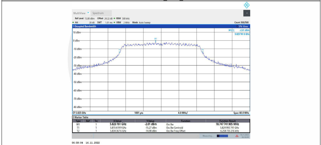
11AC20MIMO_Ant2_5825
