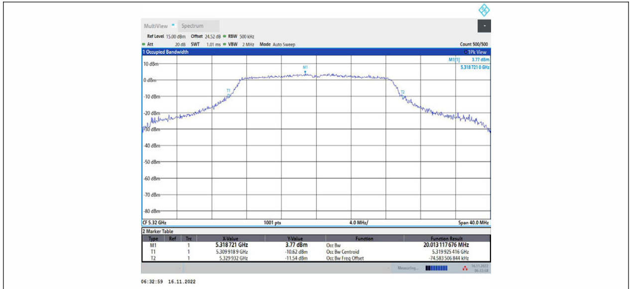
11AC20MIMO_Ant1_5320
