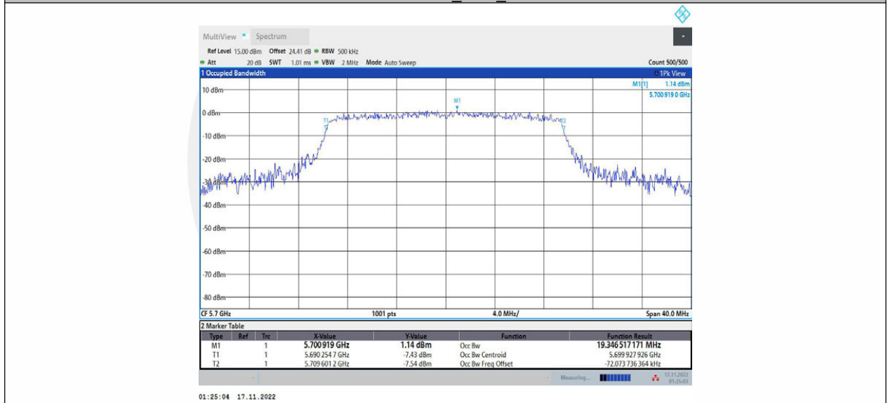
11AX20MIMO_Ant2_5700
