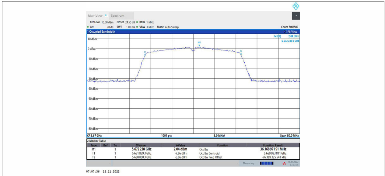
11AC40MIMO_Ant1_5670
