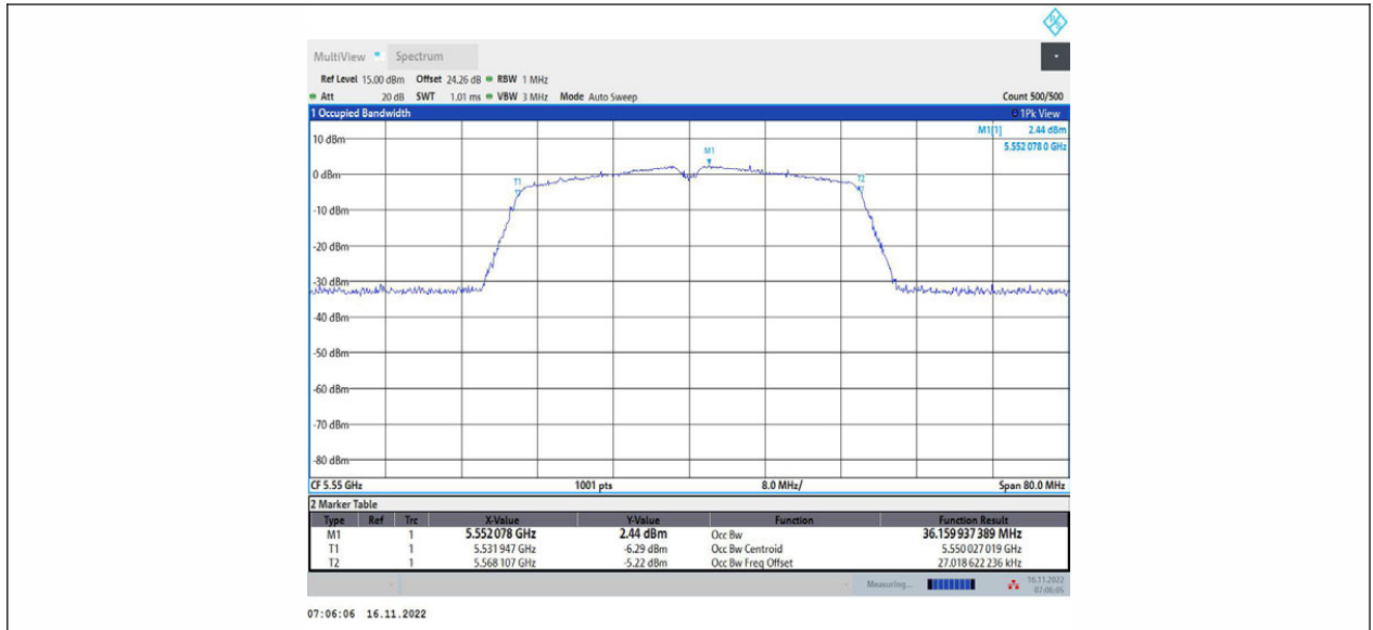
11AC40MIMO_Ant1_5550
