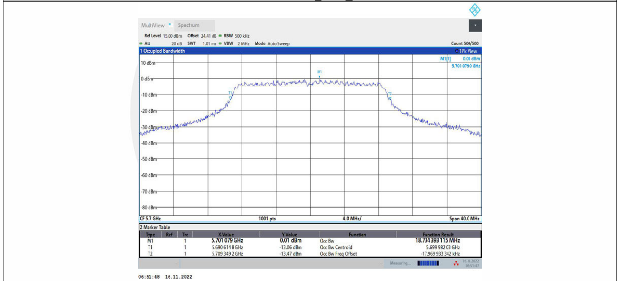
11AC20MIMO_Ant2_5700
