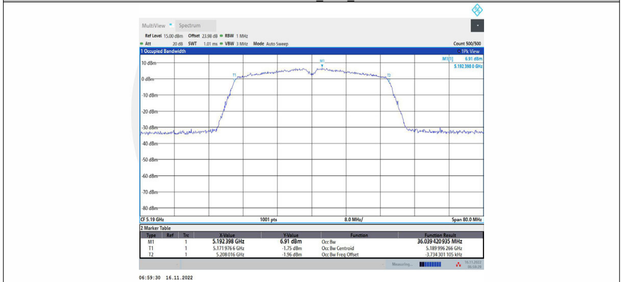
11AC40MIMO_Ant2_5190
