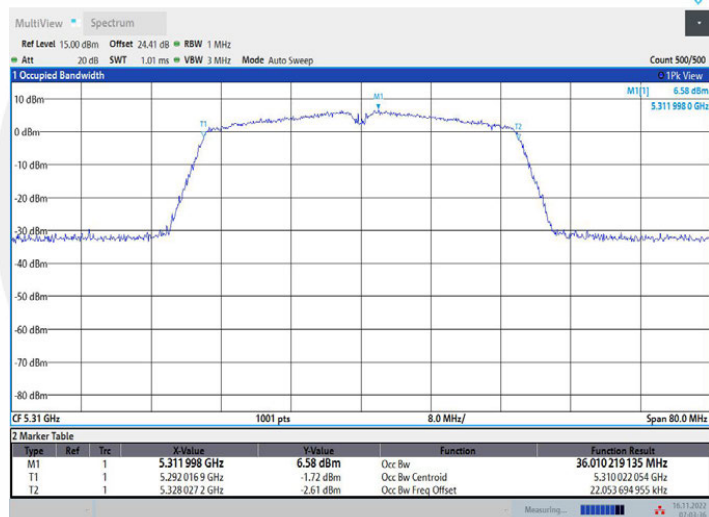
11AC40MIMO_Ant2_5310
