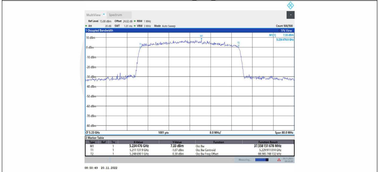
11AX40MIMO_Ant2_5230
