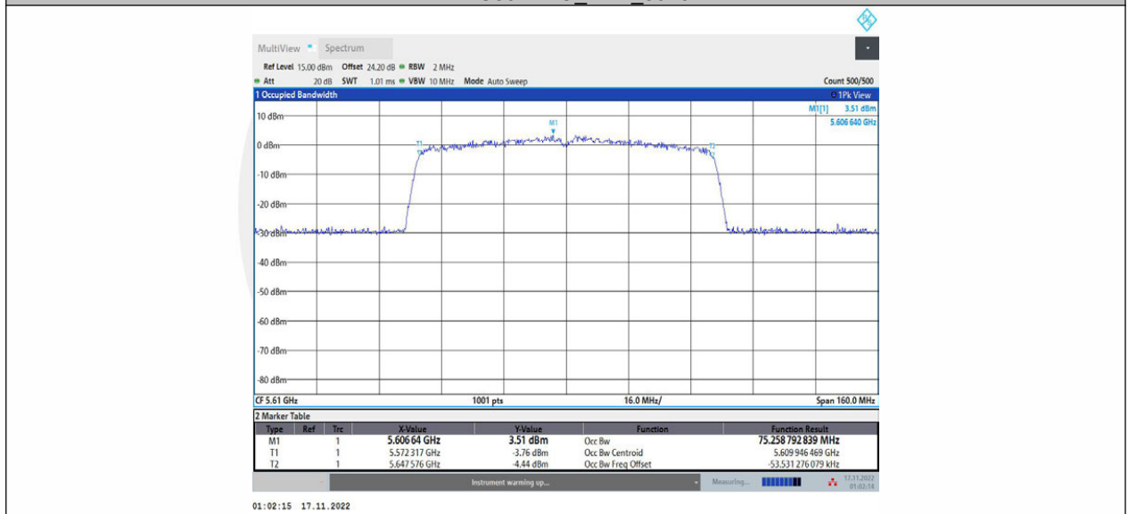
11AC80MIMO_Ant2_5610
