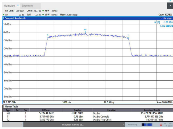
11AC80MIMO_Ant2_5775
