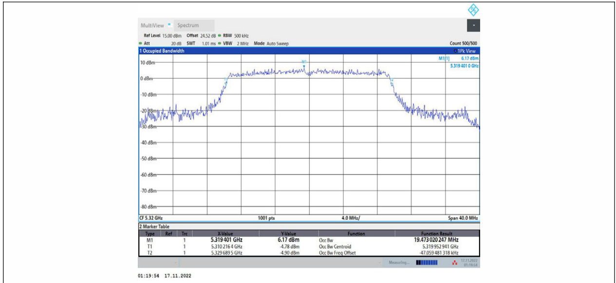
11AX20MIMO_Ant1_5320
