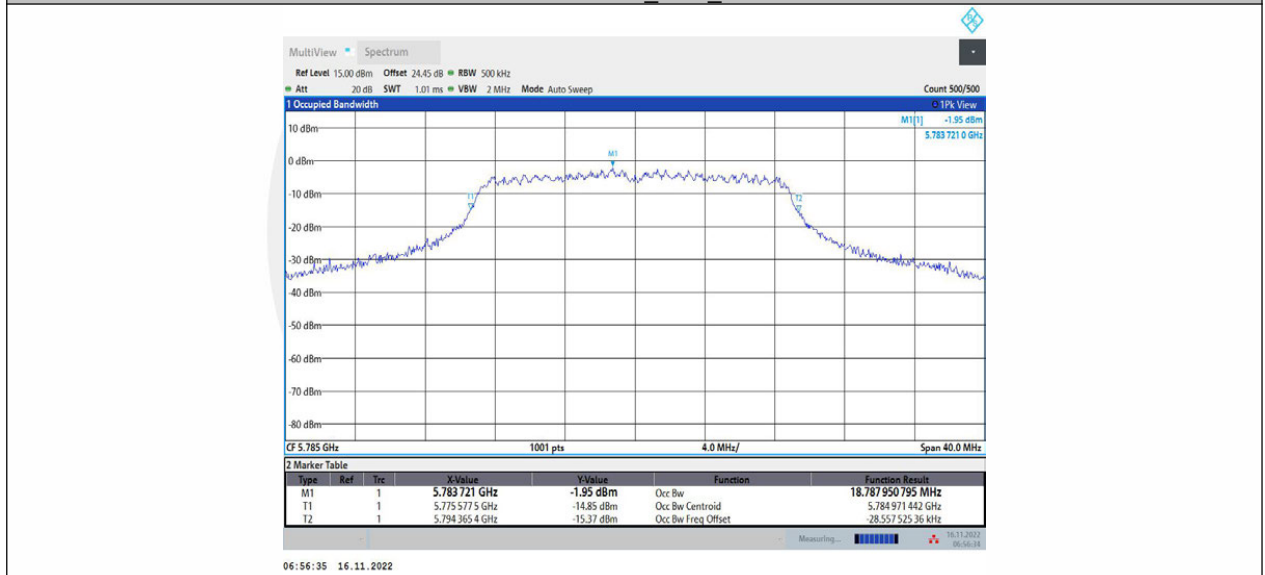
11AC20MIMO_Ant2_5785
