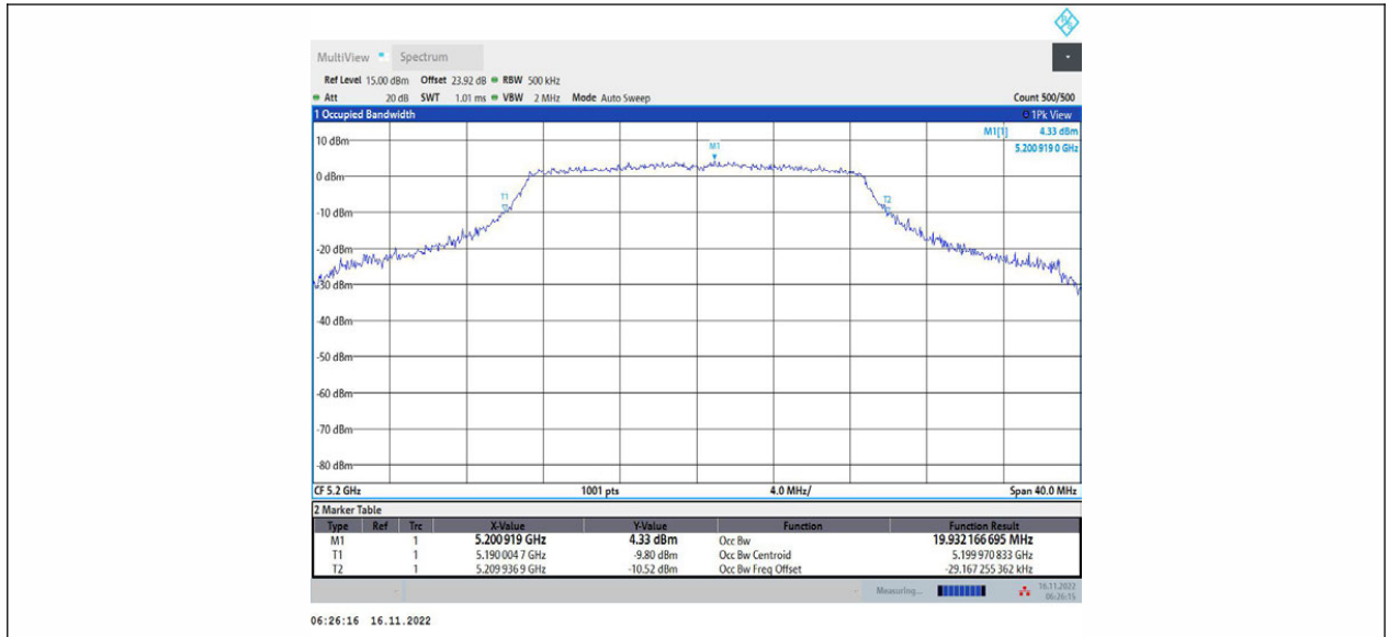
11AC20MIMO_Ant1_5200
