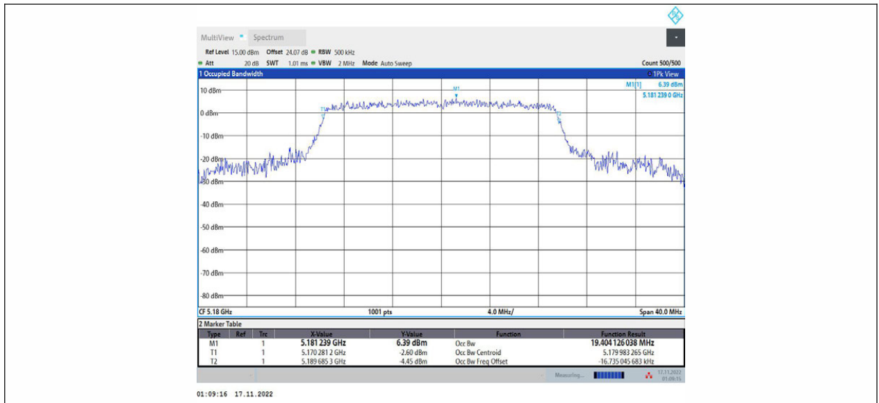
11AX20MIMO_Ant1_5180
