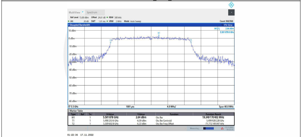
11AX20MIMO_Ant2_5500
