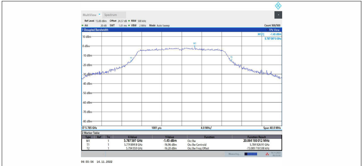
11AC20MIMO_Ant1_5785
