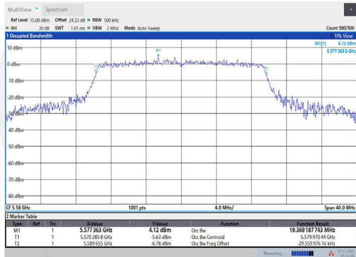
11AX20MIMO_Ant2_5580
