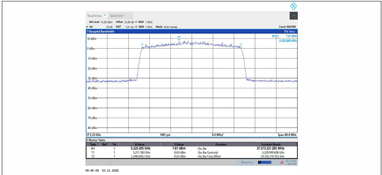
11AX40MIMO_Ant1_5230
