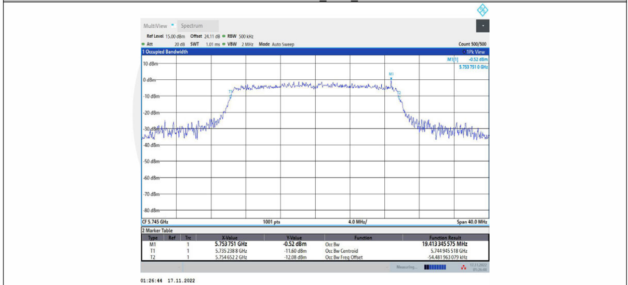
11AX20MIMO_Ant2_5745
