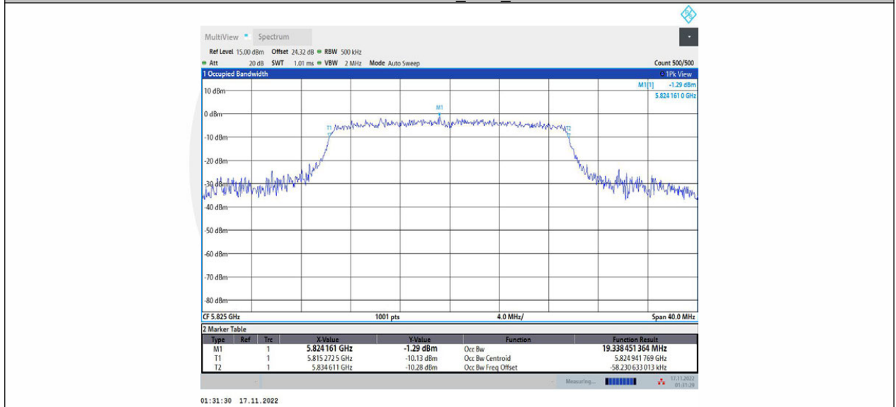
11AX20MIMO_Ant2_5825
