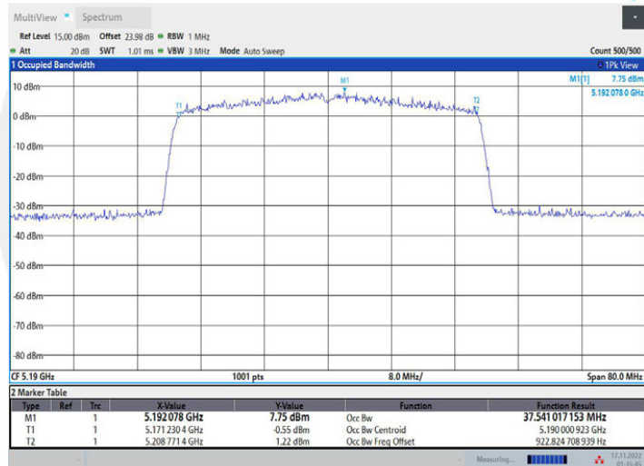
11AX40MIMO_Ant2_5190
