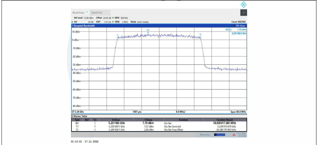
11AX20MIMO_Ant2_5240
