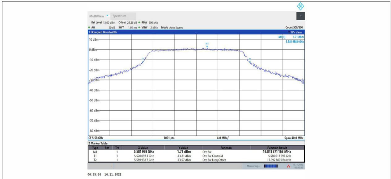
11AC20MIMO_Ant1_5580
