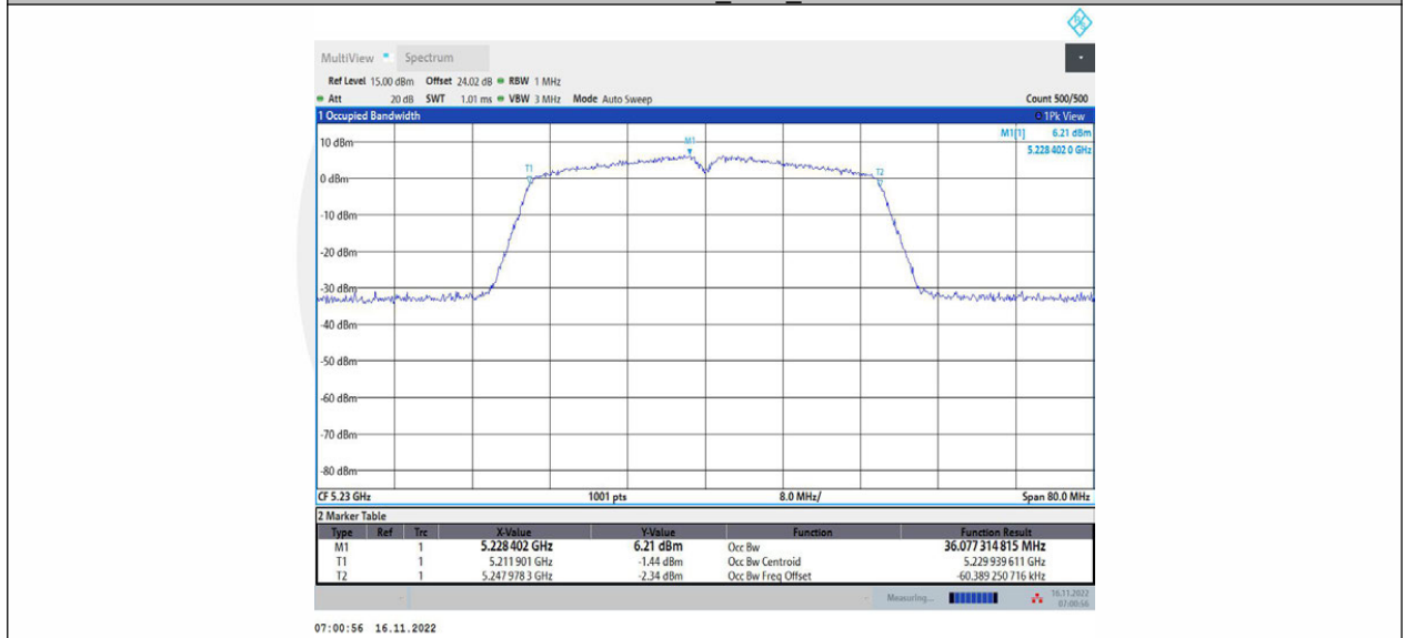
11AC40MIMO_Ant2_5230
