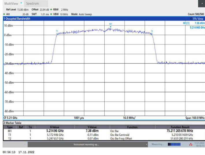
11AC80MIMO_Ant1_5210
