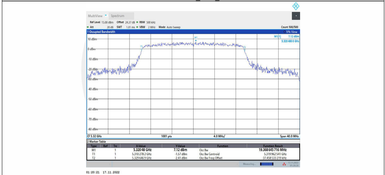
11AX20MIMO_Ant2_5320
