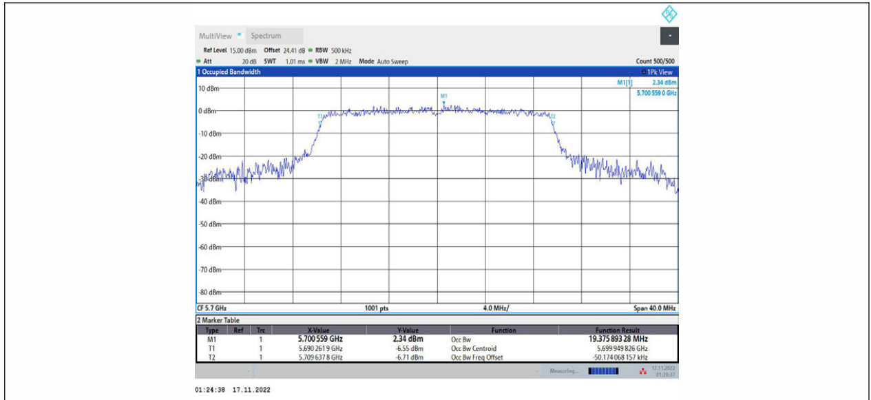
11AX20MIMO_Ant1_5700
