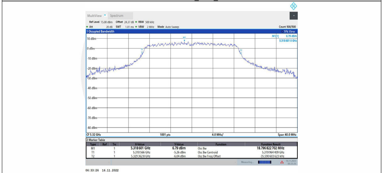
11AC20MIMO_Ant2_5320
