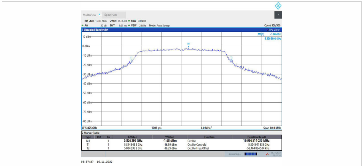
11AC20MIMO_Ant1_5825
