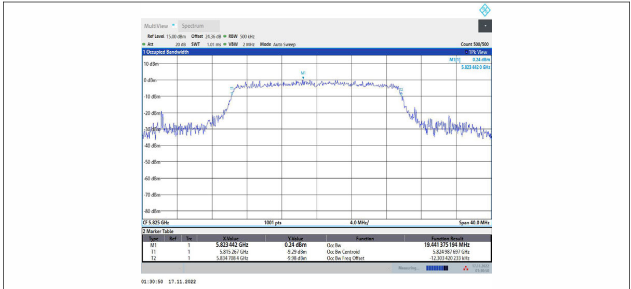
11AX20MIMO_Ant1_5825
