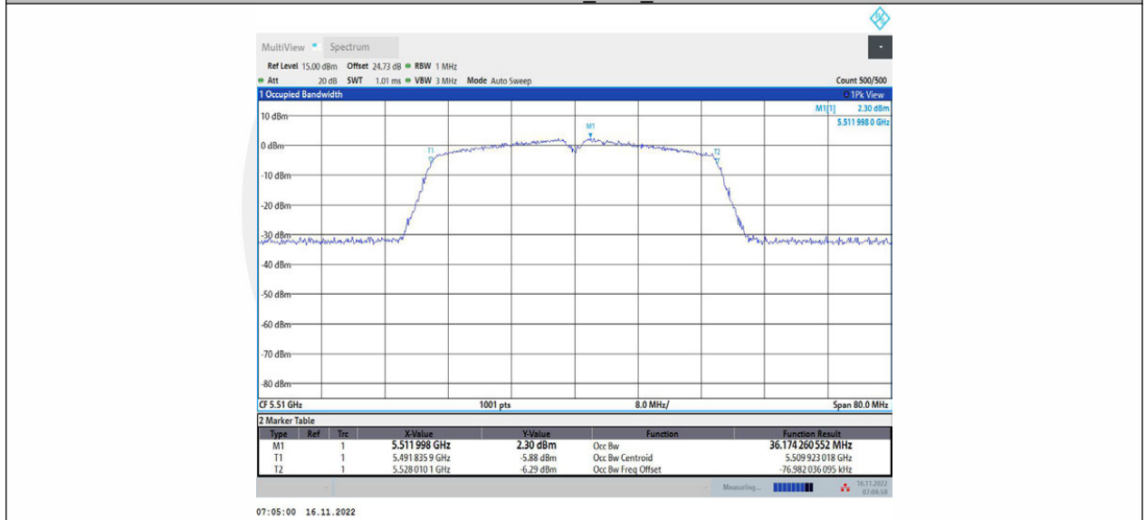
11AC40MIMO_Ant2_5510
