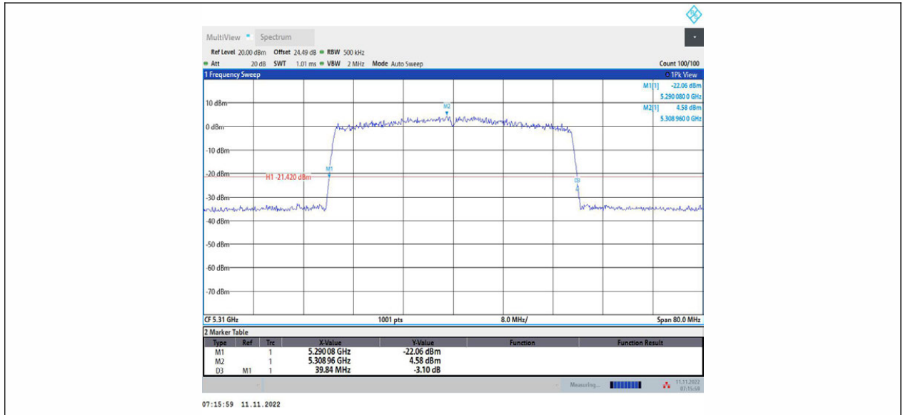
11AX40MIMO_Ant1_5310
