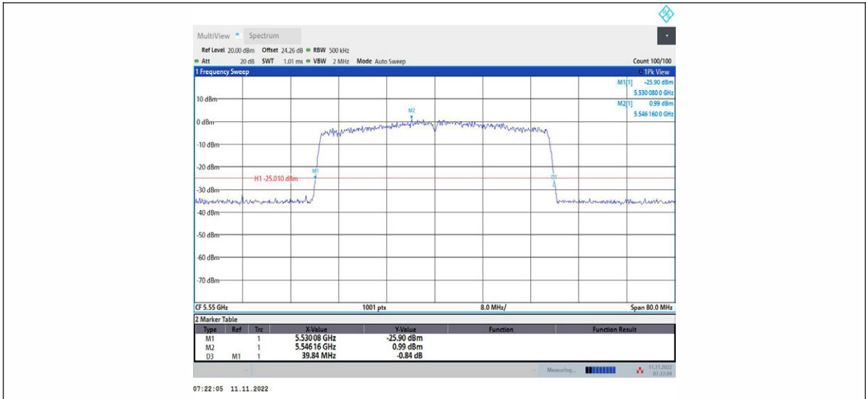
11AX40MIMO_Ant1_5550
