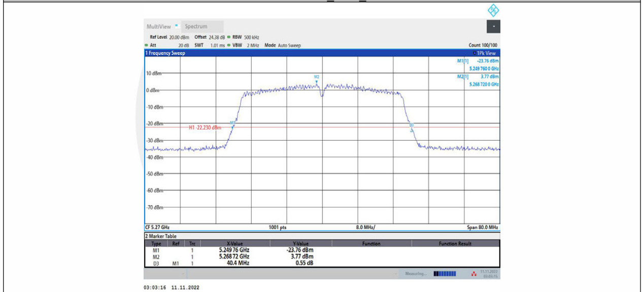
11AC40MIMO_Ant2_5270
