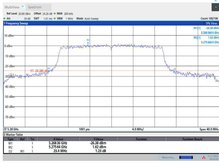
11AX20MIMO_Ant2_5280
