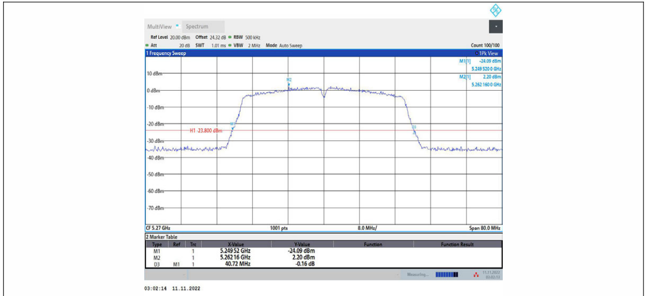
11AC40MIMO_Ant1_5270
