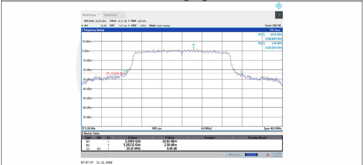
11AX20MIMO_Ant2_5260
