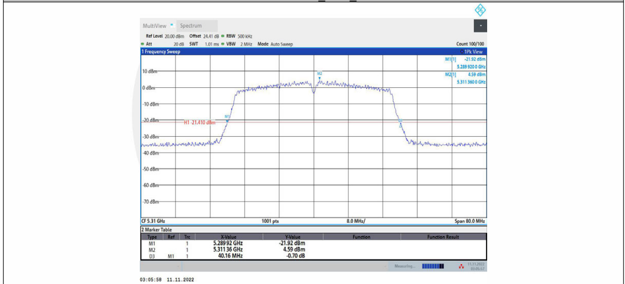
11AC40MIMO_Ant2_5310
