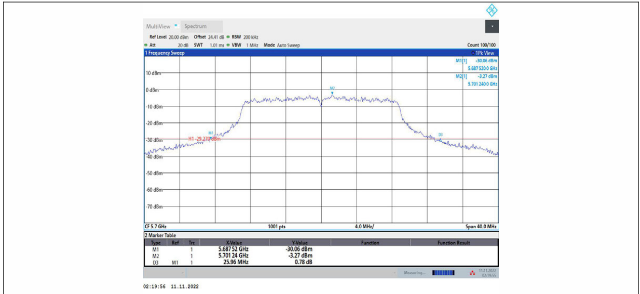
11AC20MIMO_Ant1_5700
