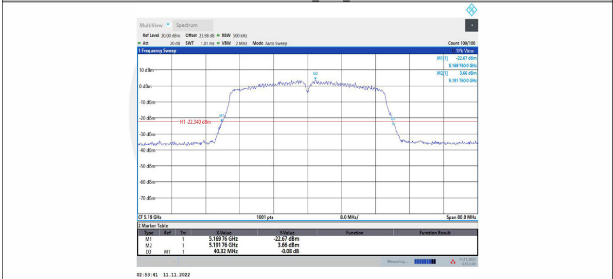
11AC40MIMO_Ant2_5190
