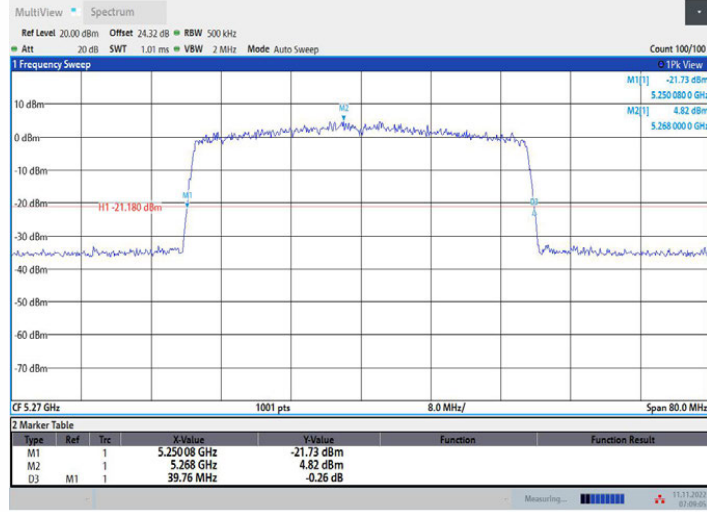
11AX40MIMO_Ant1_5270
