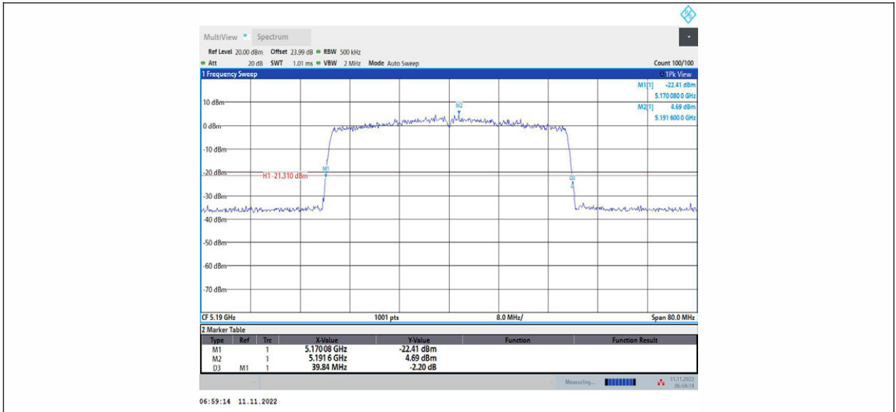
11AX40MIMO_Ant1_5190
