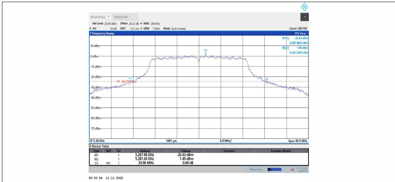
11AC20MIMO_Ant1_5280
