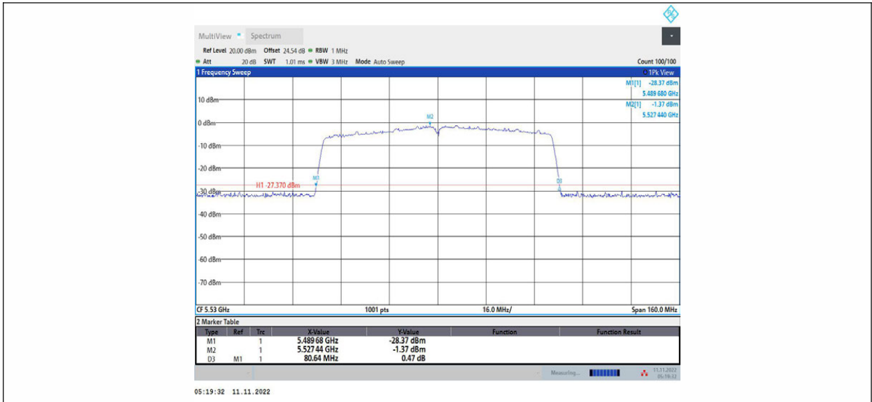
11AC80MIMO_Ant1_5530
