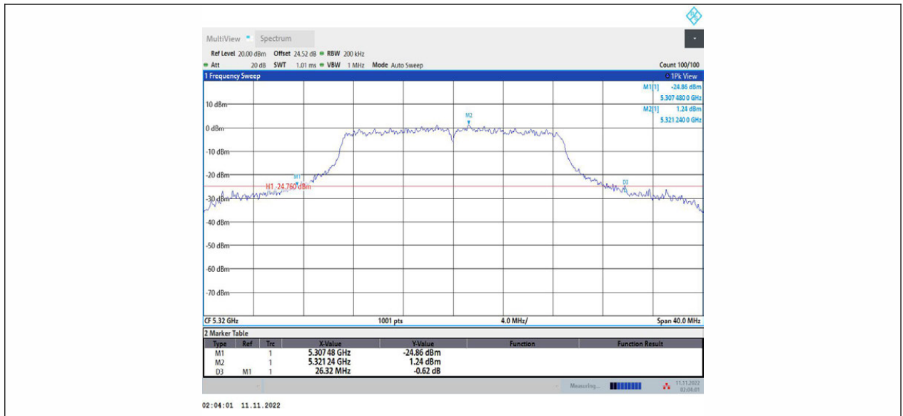
11AC20MIMO_Ant1_5320
