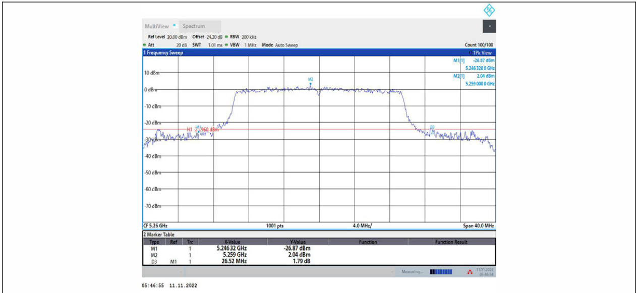
11AX20MIMO_Ant1_5260
