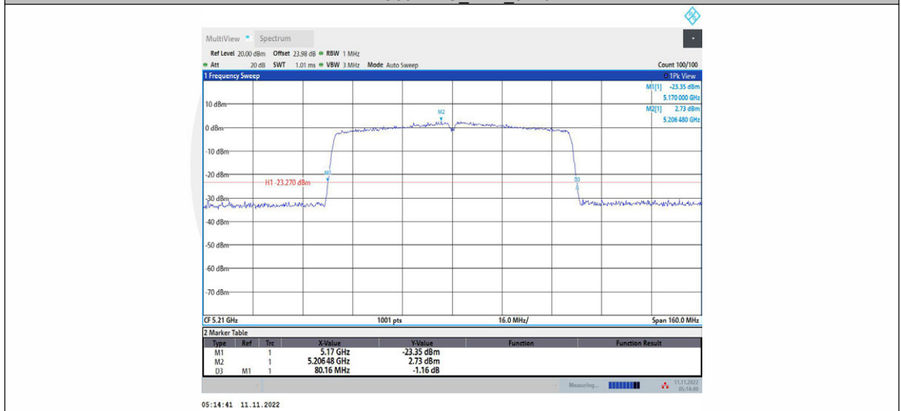
11AC80MIMO_Ant2_5210
