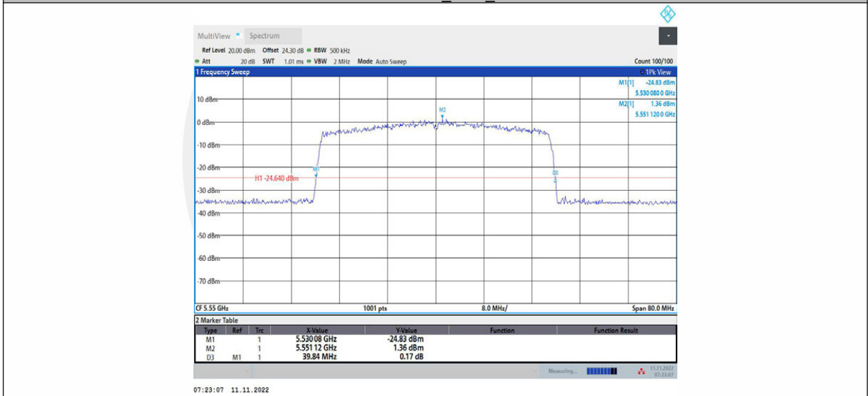
11AX40MIMO_Ant2_5550
