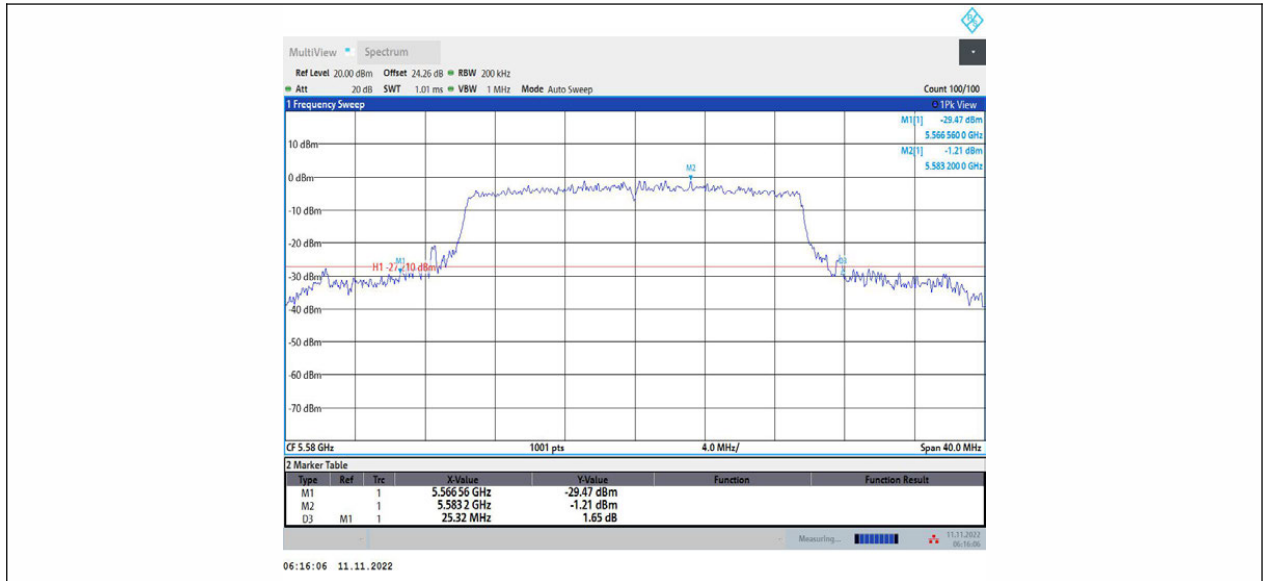
11AX20MIMO_Ant1_5580
