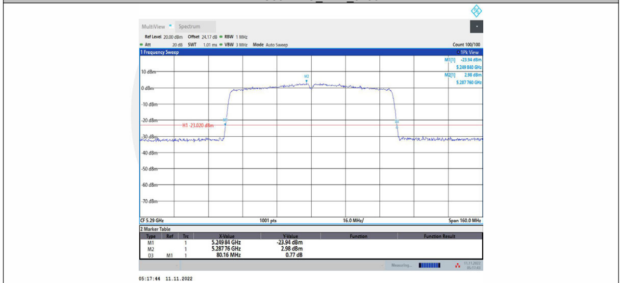
11AC80MIMO_Ant2_5290
