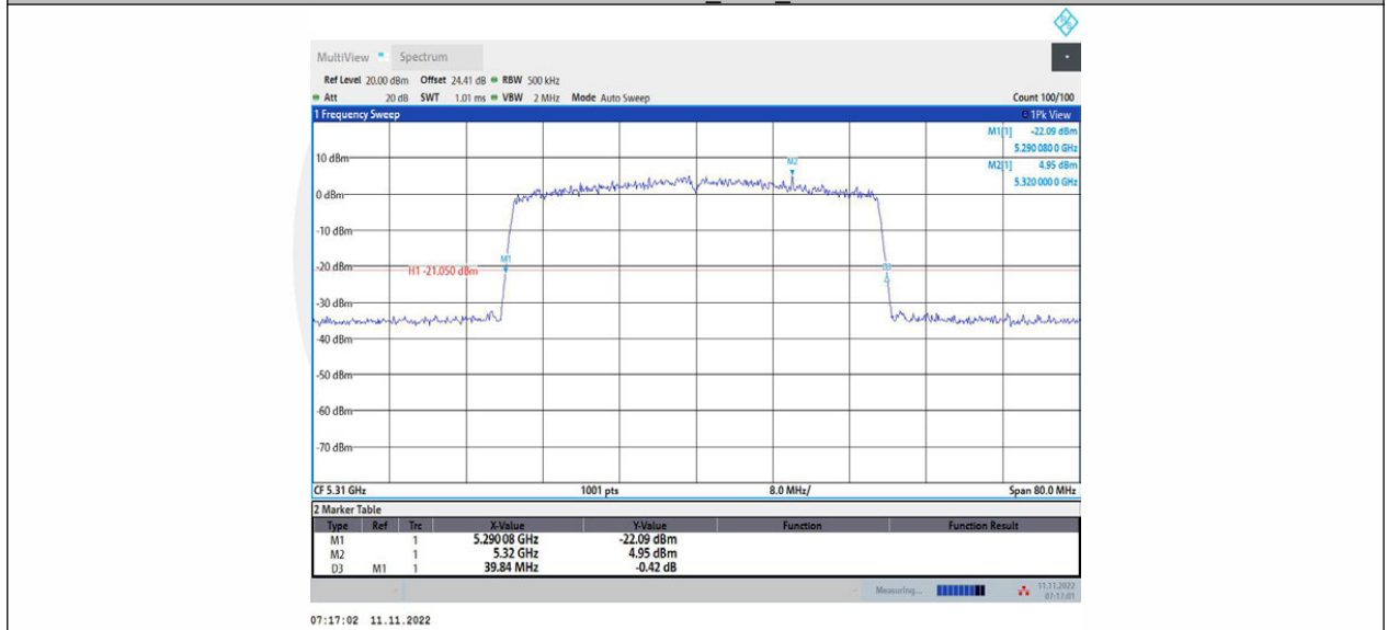
11AX40MIMO_Ant2_5310
