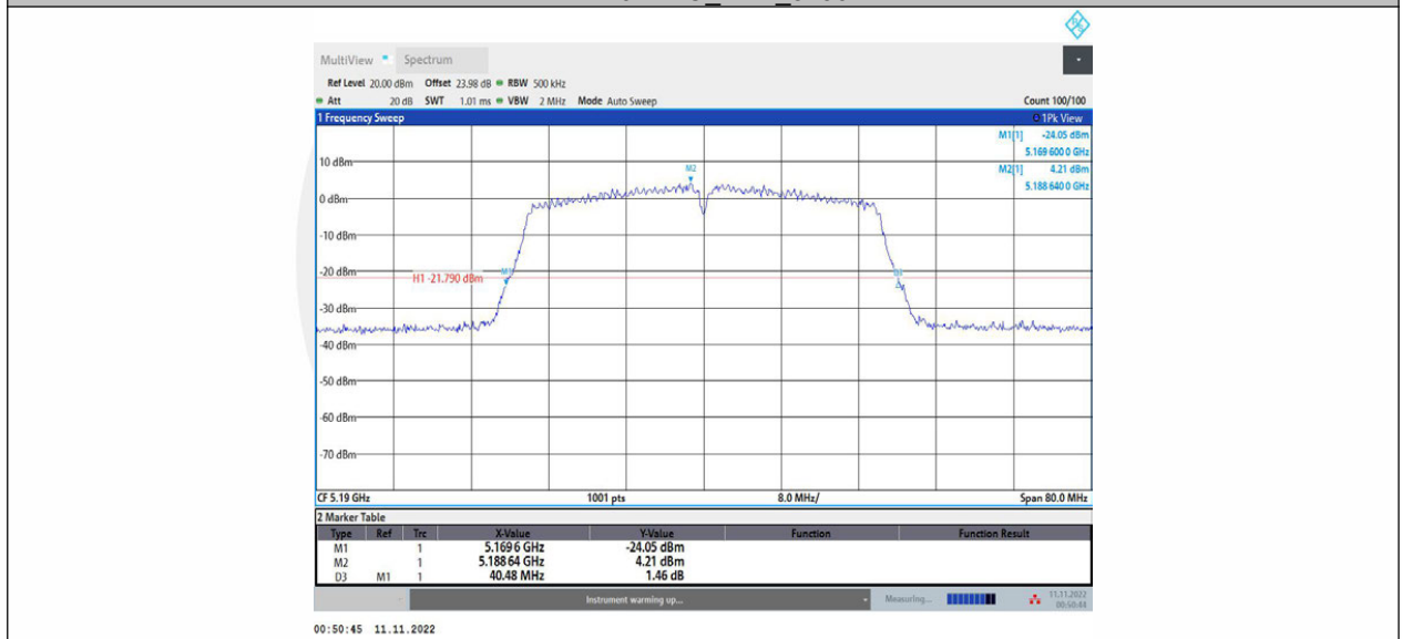
11N40MIMO_Ant2_5190
