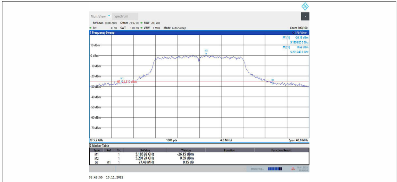
11A_Ant1_5200
