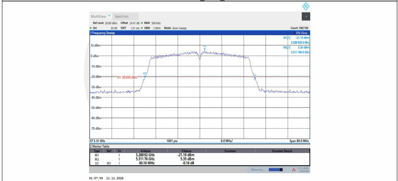
11N40MIMO_Ant2_5310
