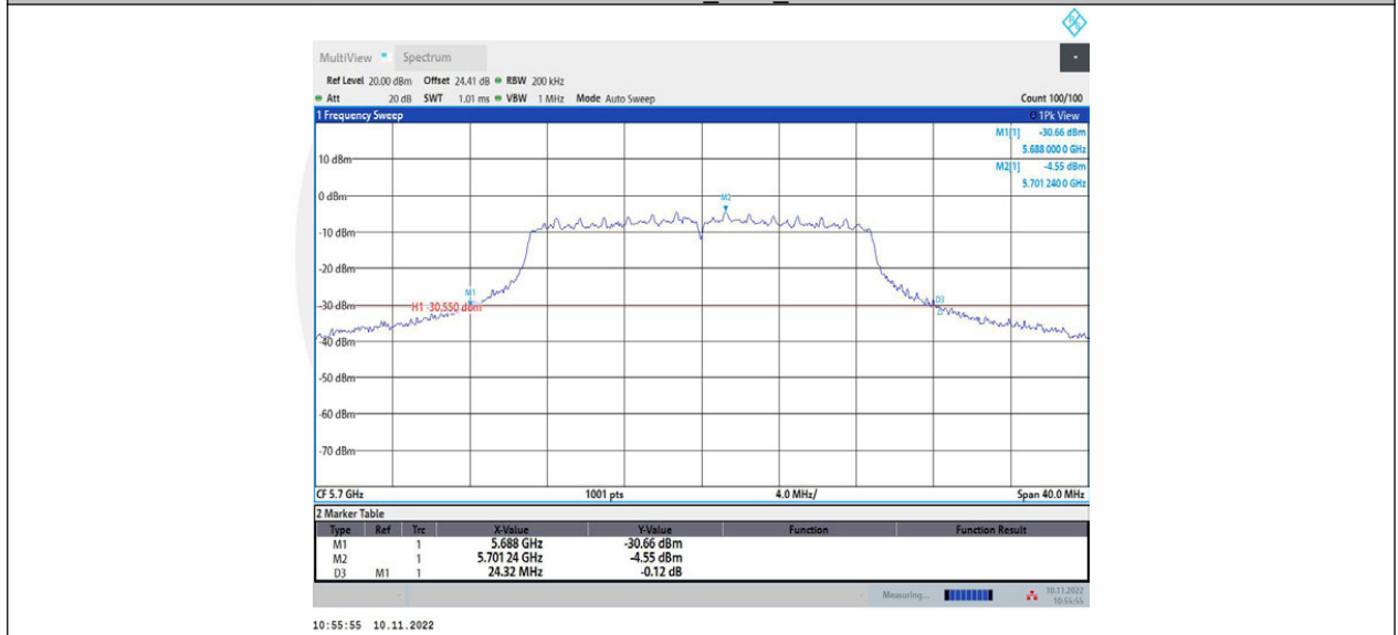
11N20MIMO_Ant2_5700
