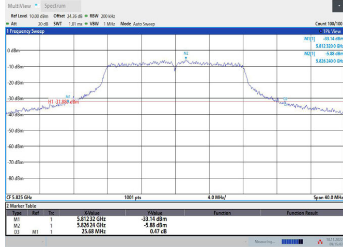
11A_Ant1_5825
