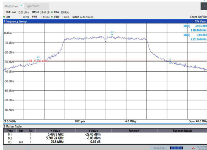
11A_Ant2_5500
