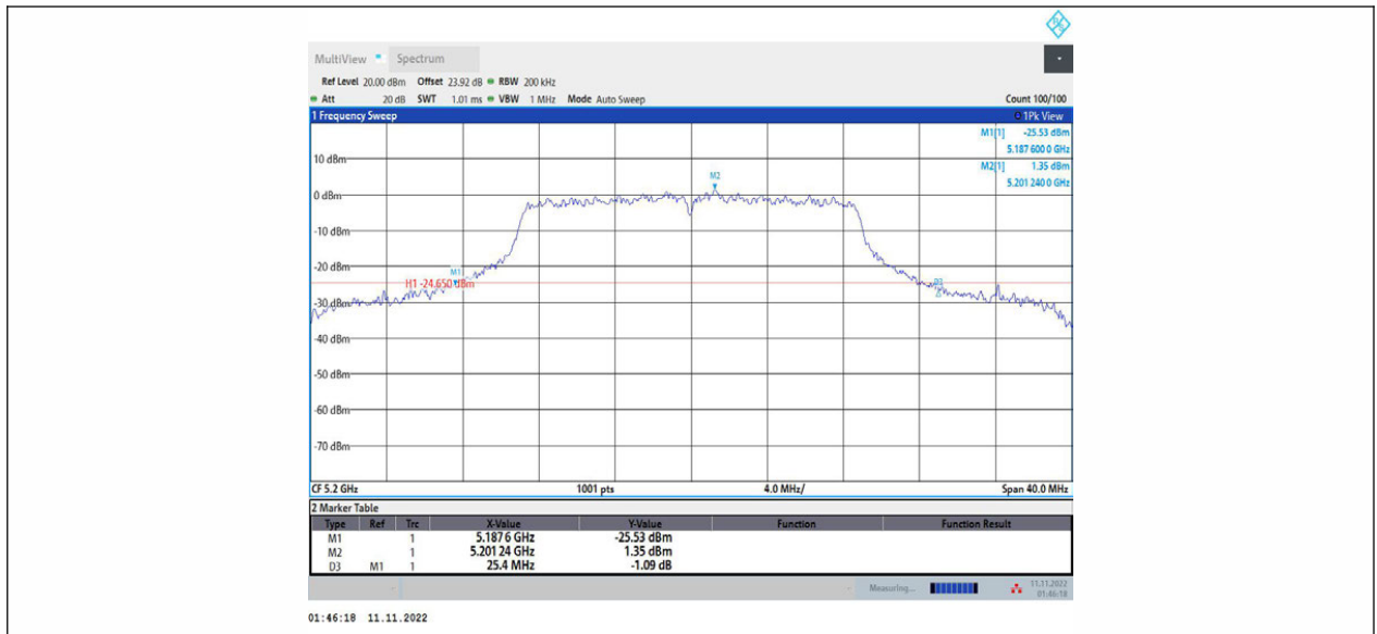
11AC20MIMO_Ant1_5200
