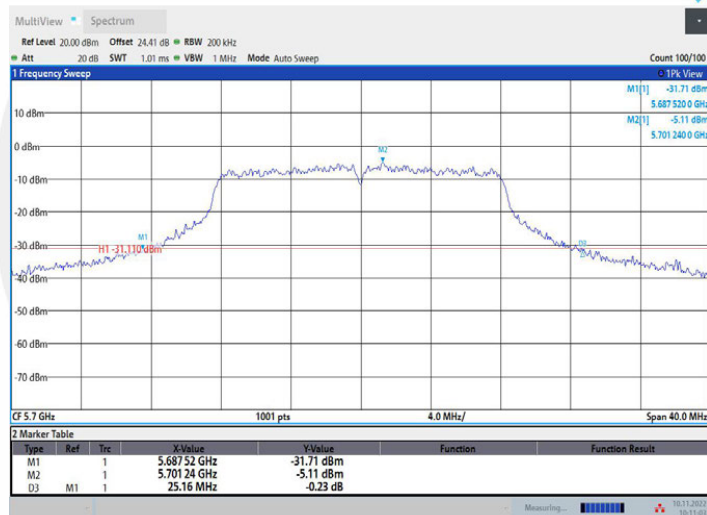
11A_Ant2_5700
