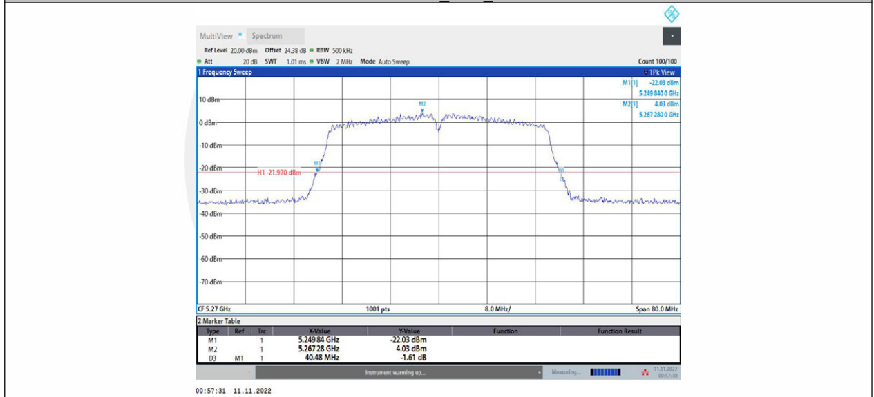
11N40MIMO_Ant2_5270
