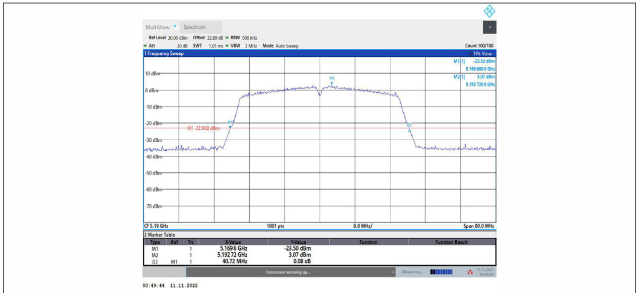
11N40MIMO_Ant1_5190
