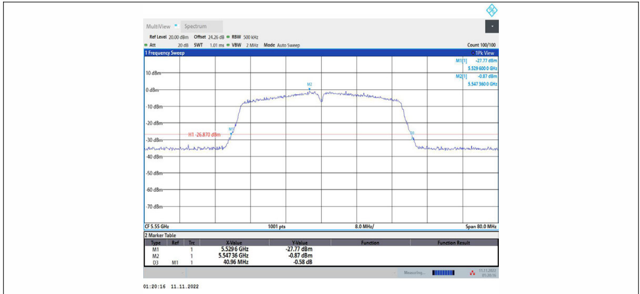
11N40MIMO_Ant1_5550
