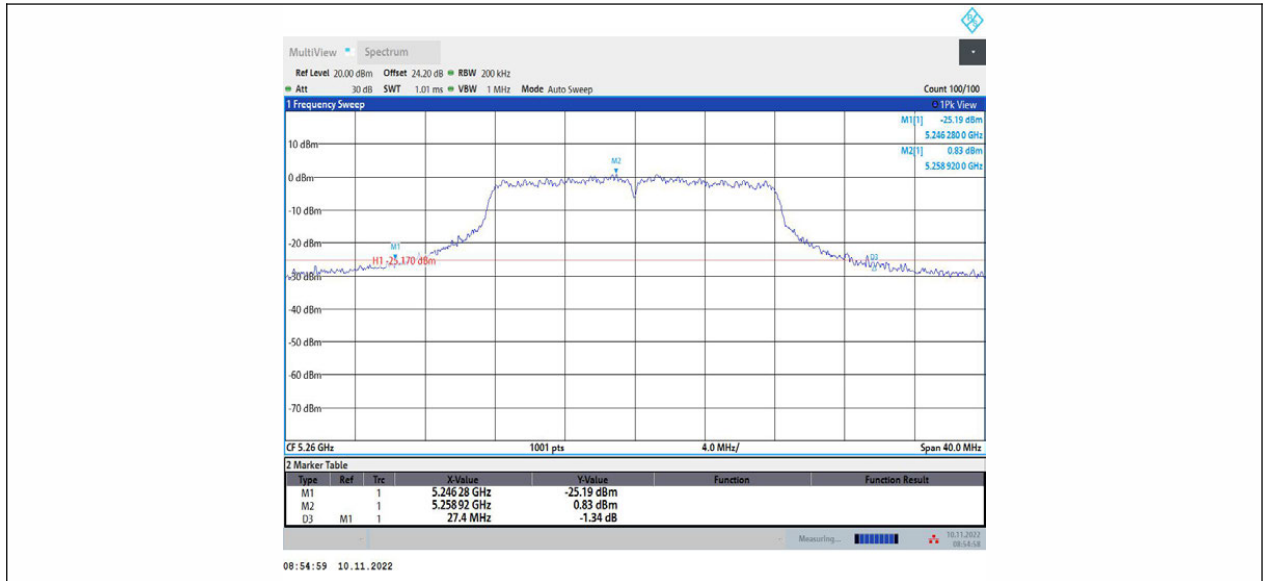
11A_Ant1_5260
