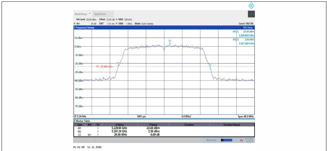
11AC20MIMO_Ant1_5240
