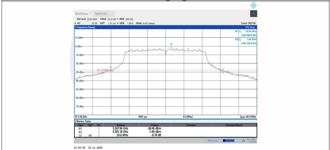
11N20MIMO_Ant2_5580
