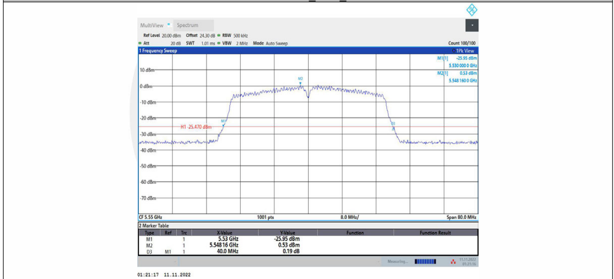
11N40MIMO_Ant2_5550
