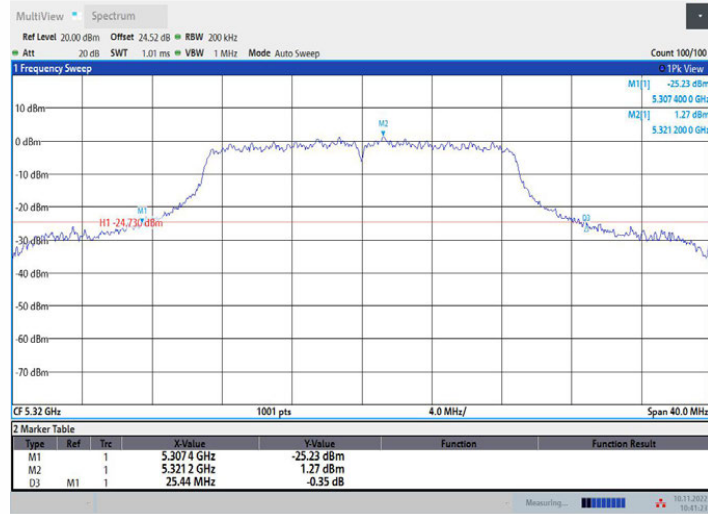
11N20MIMO_Ant1_5320
