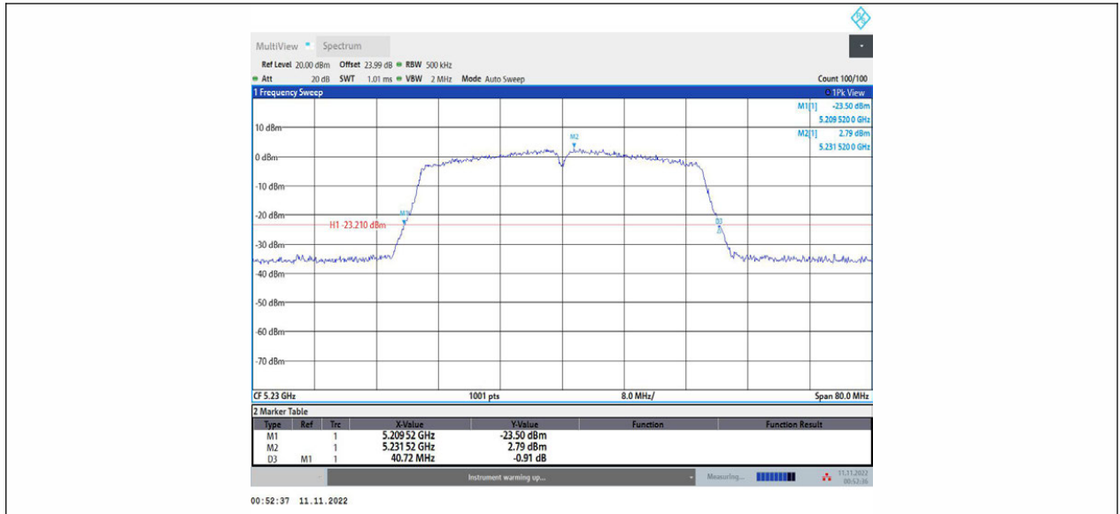
11N40MIMO_Ant1_5230
