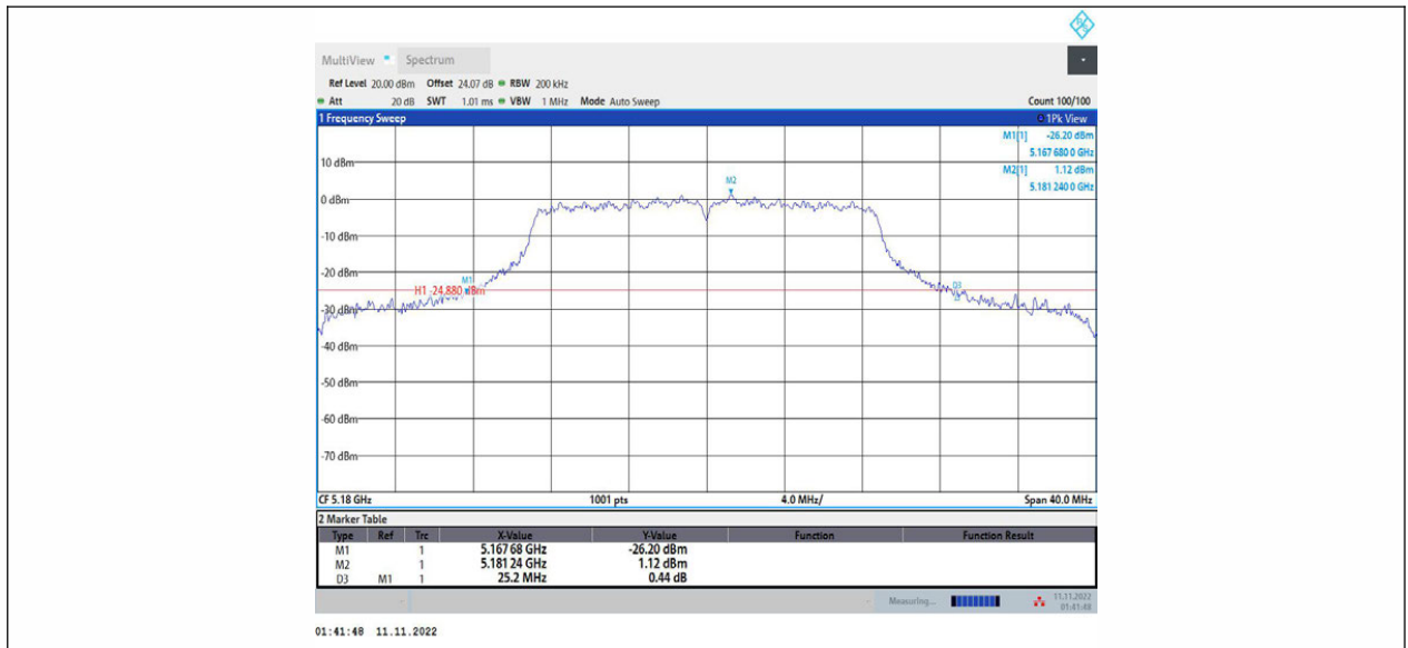
11AC20MIMO_Ant1_5180
