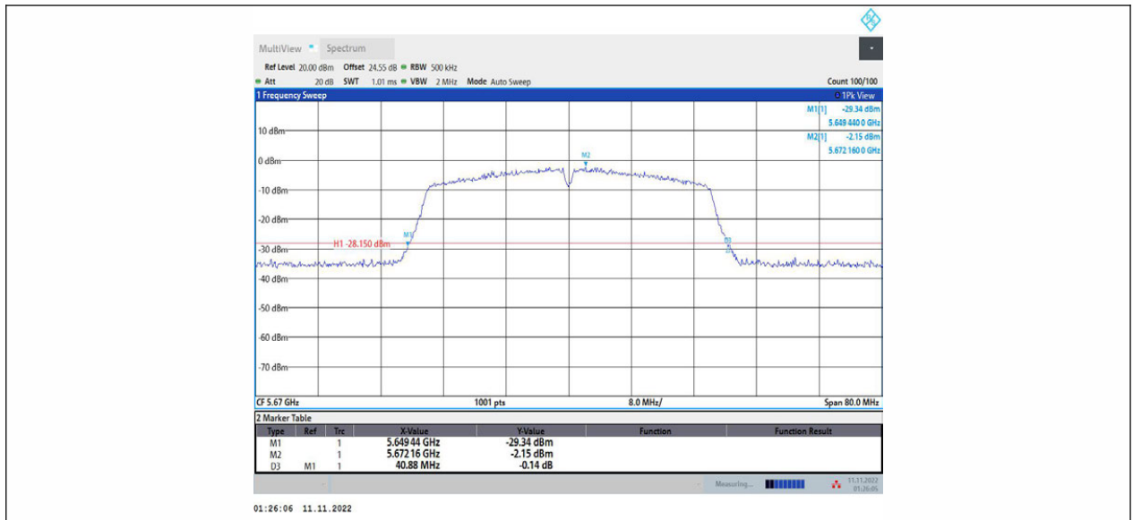
11N40MIMO_Ant1_5670
