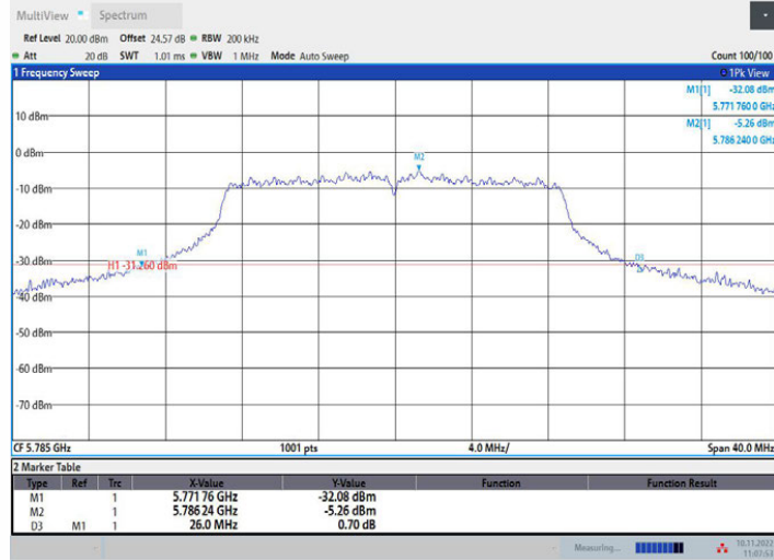
11N20MIMO_Ant1_5785
