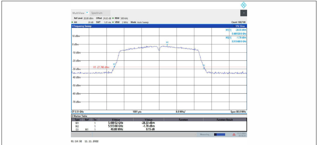
11N40MIMO_Ant1_5510
