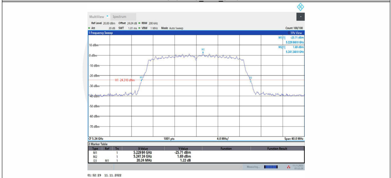
11AC20MIMO_Ant2_5240
