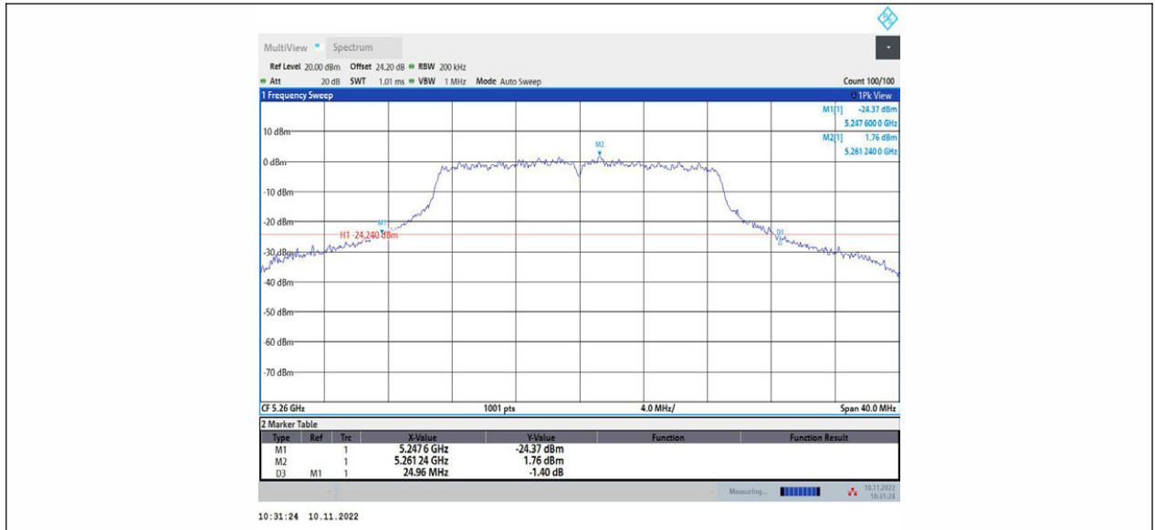
11N20MIMO_Ant1_5260
