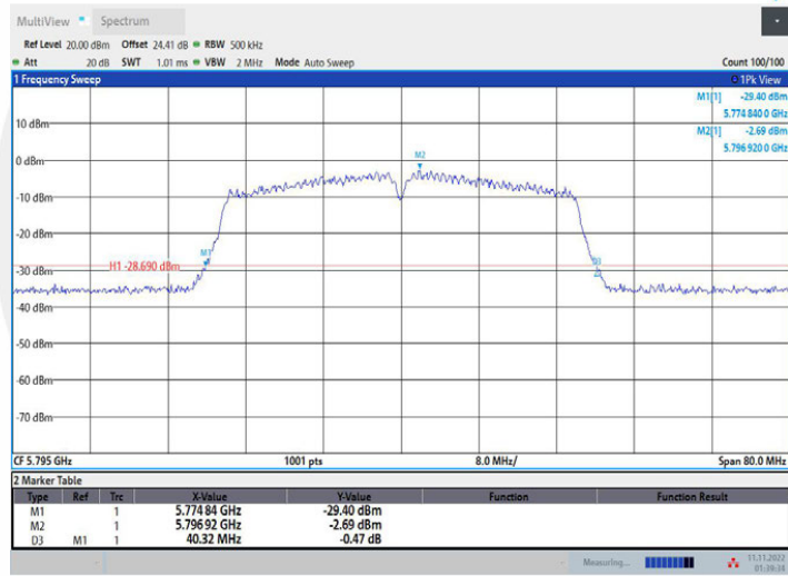
11N40MIMO_Ant2_5795
