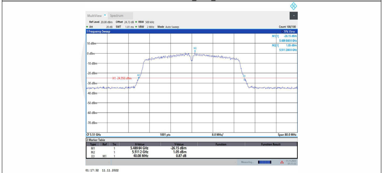
11N40MIMO_Ant2_5510
