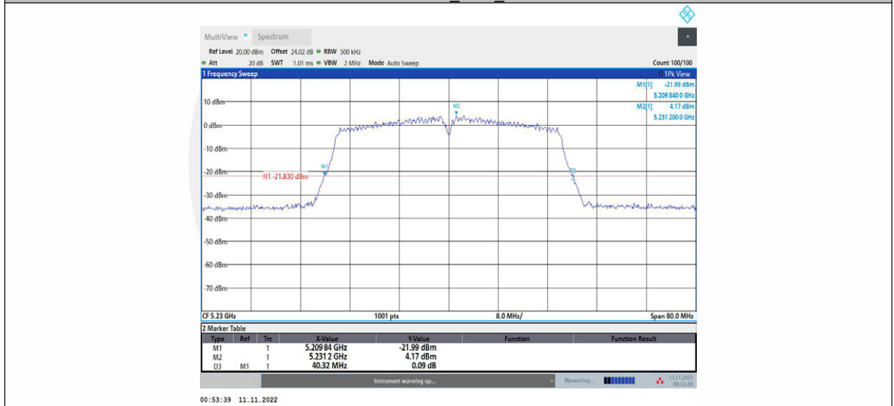
11N40MIMO_Ant2_5230
