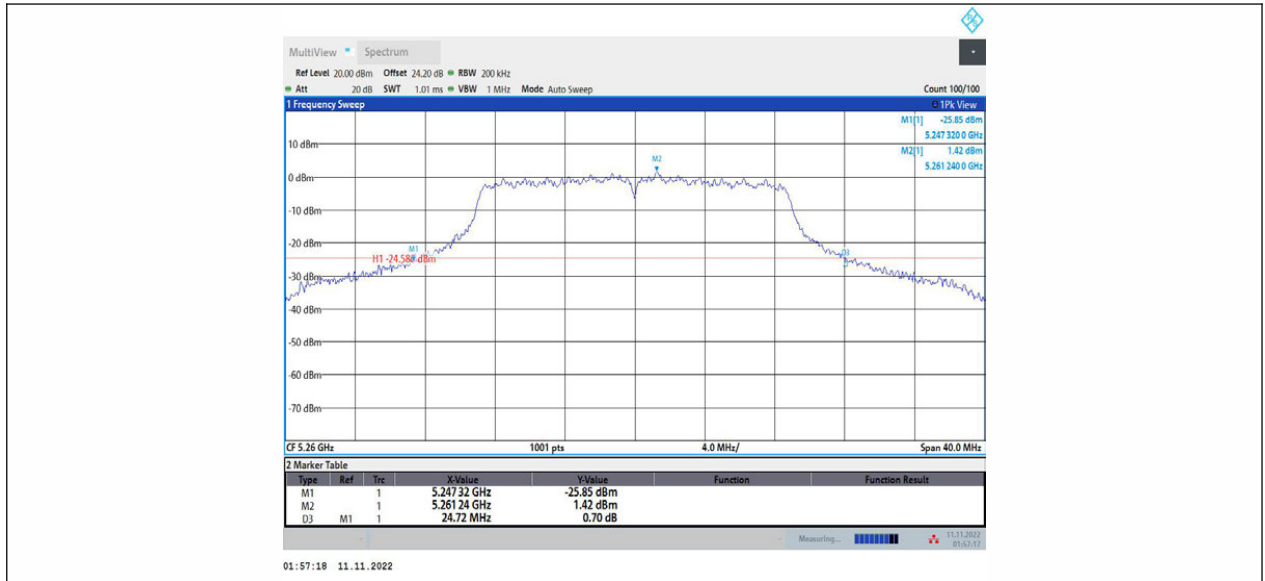
11AC20MIMO_Ant1_5260
