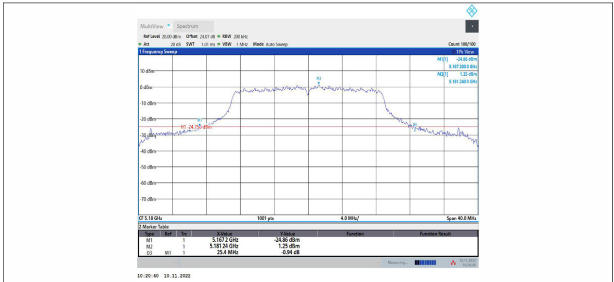
11N20MIMO_Ant1_5180
