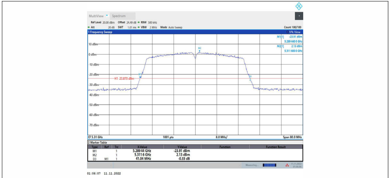
11N40MIMO_Ant1_5310
