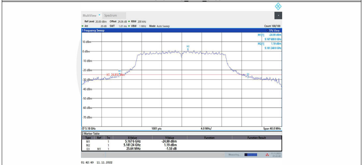
11AC20MIMO_Ant2_5180
