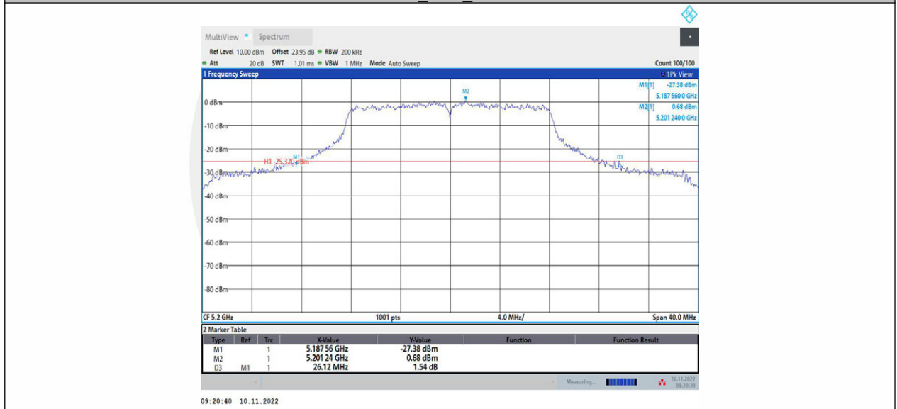
11A_Ant2_5200
