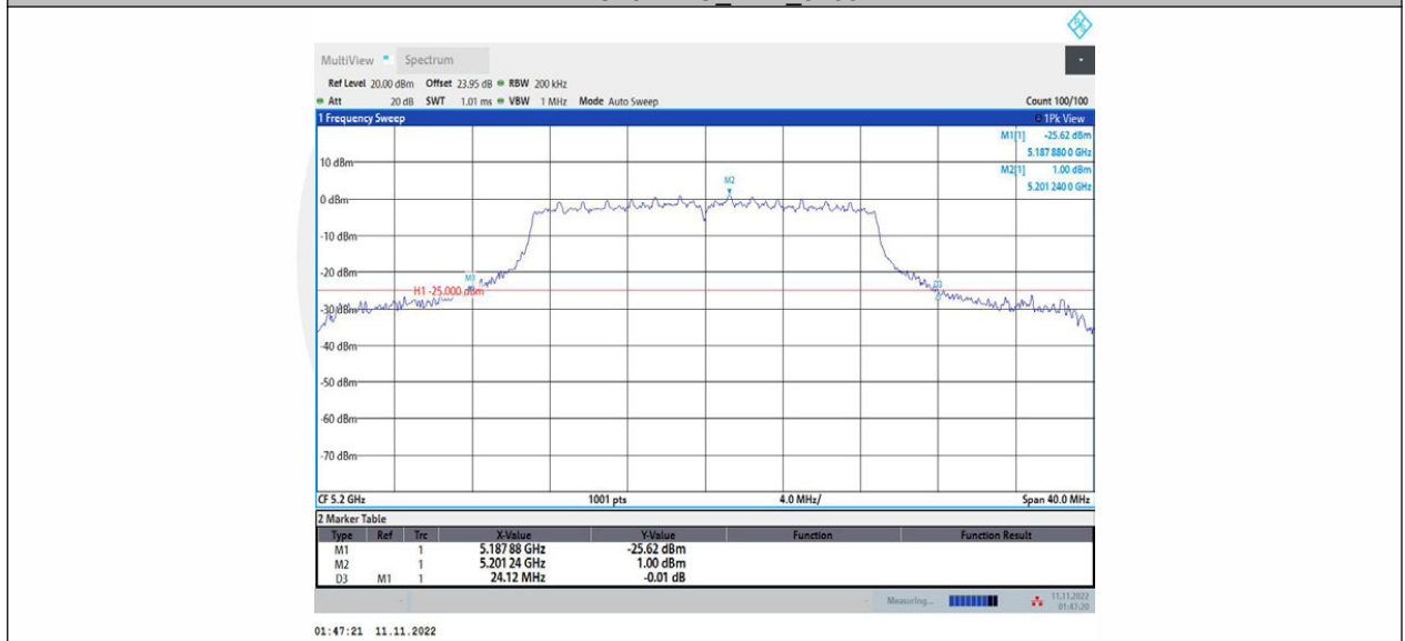
11AC20MIMO_Ant2_5200
