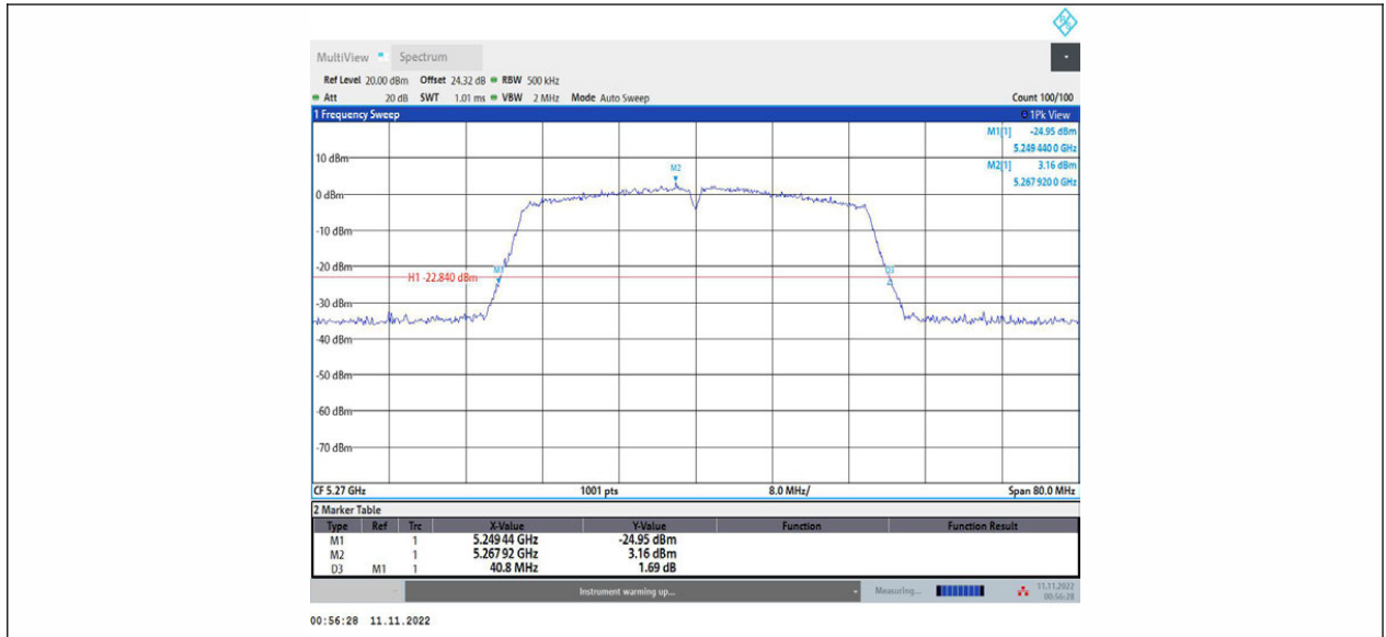
11N40MIMO_Ant1_5270
