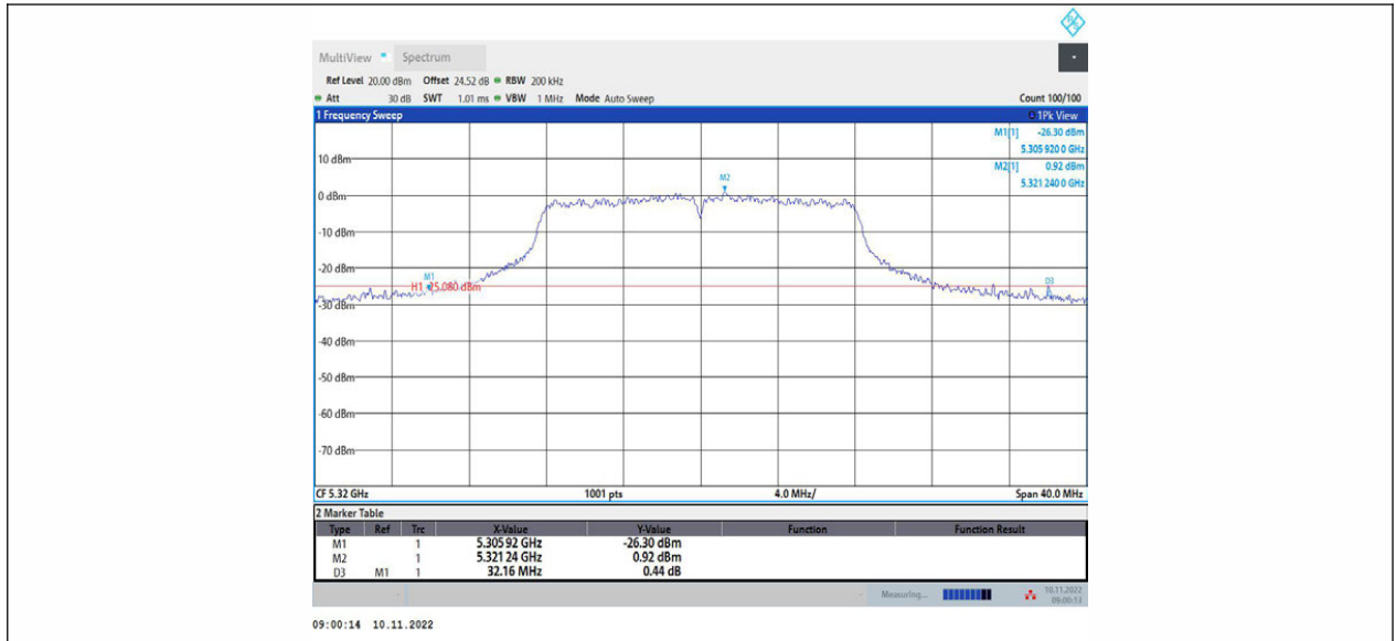
11A_Ant1_5320
