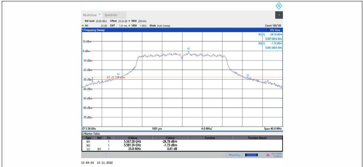
11N20MIMO_Ant1_5580
