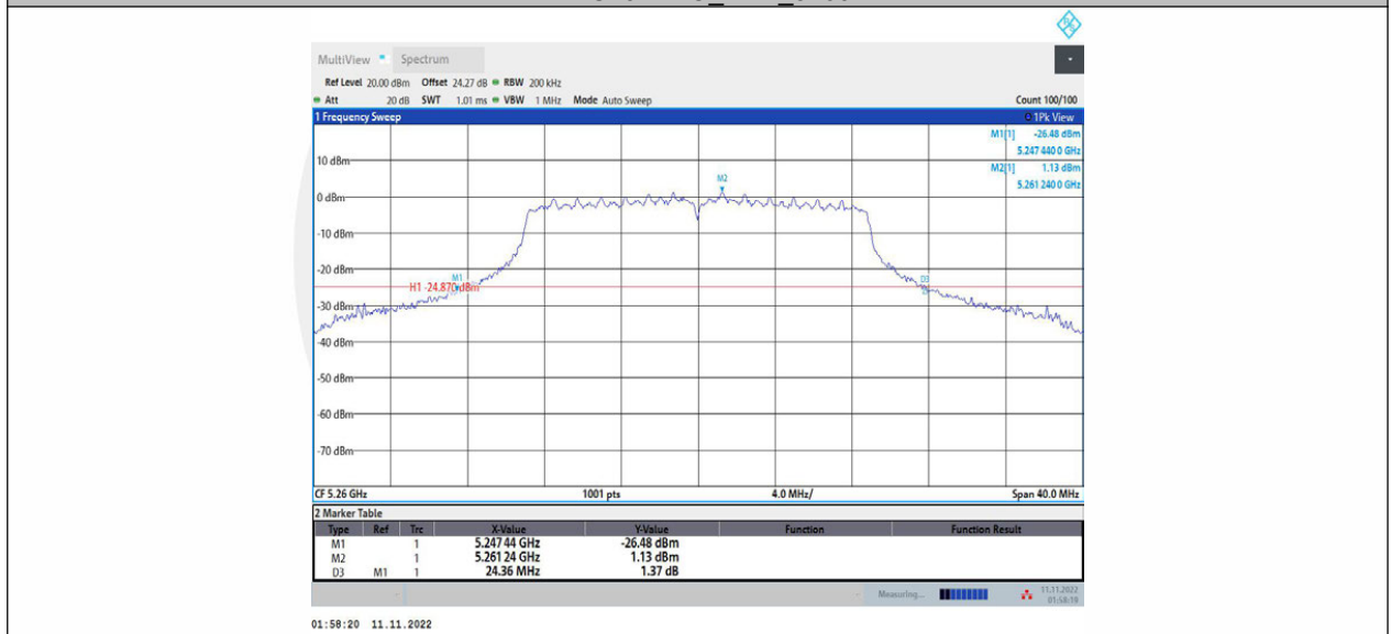
11AC20MIMO_Ant2_5260
