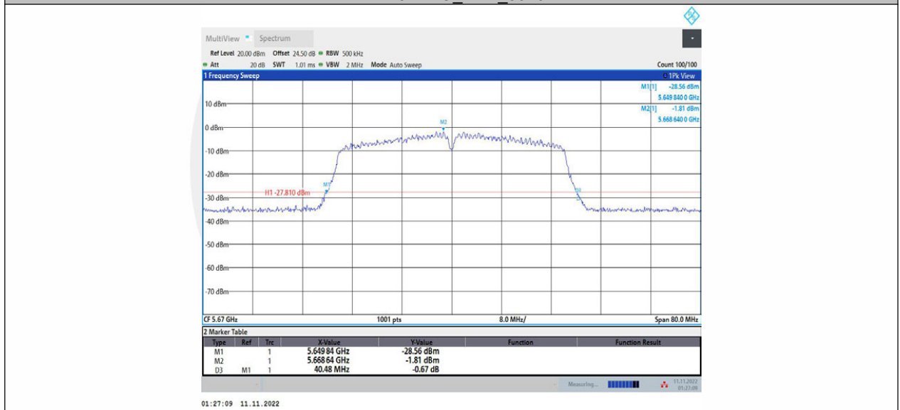
11N40MIMO_Ant2_5670
