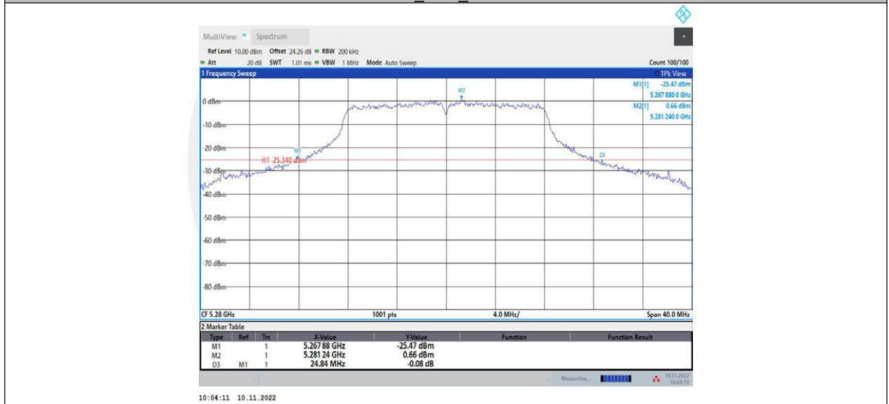
11A_Ant2_5280
