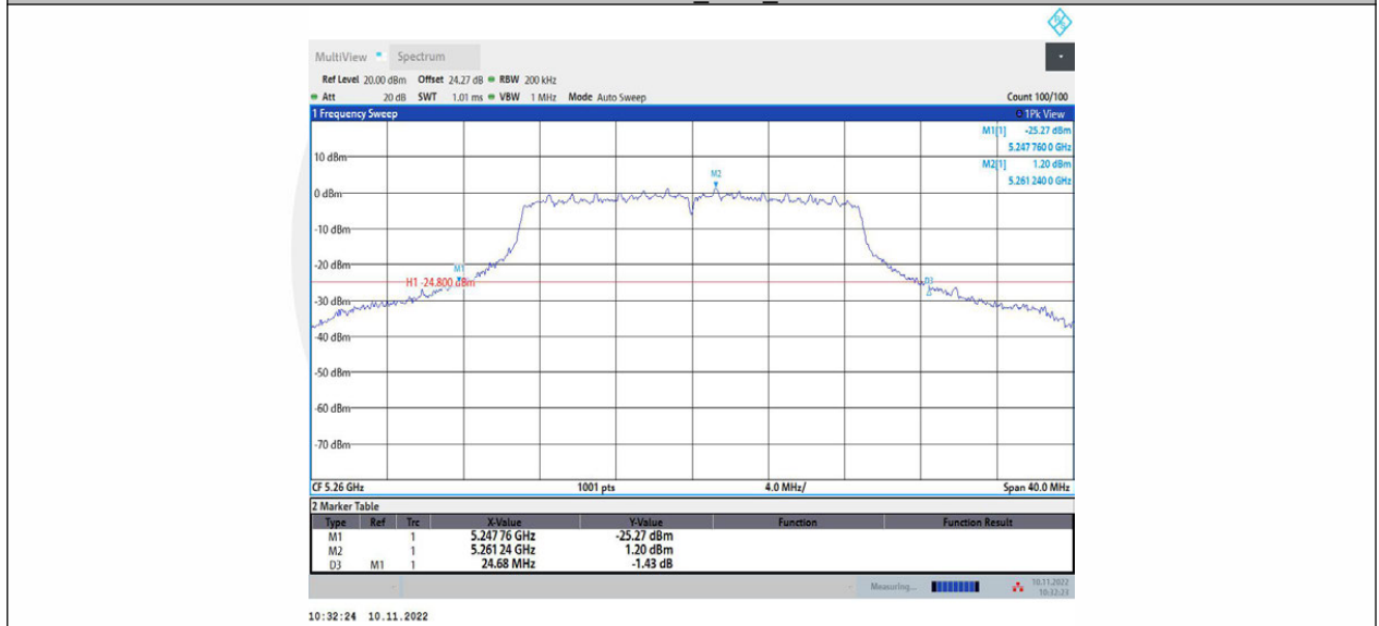
11N20MIMO_Ant2_5260
