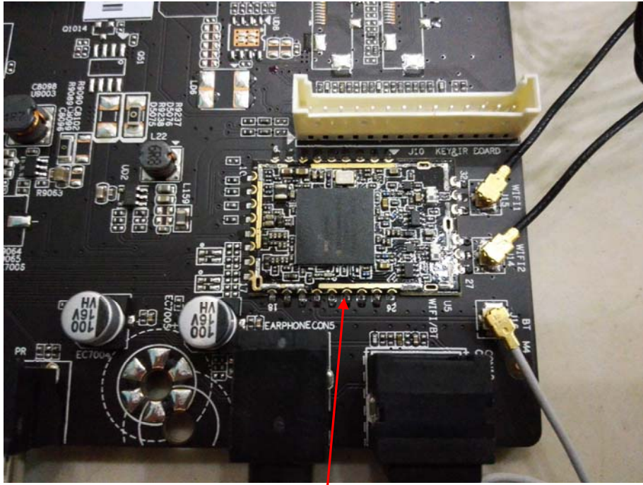
BT+WIFI Module
