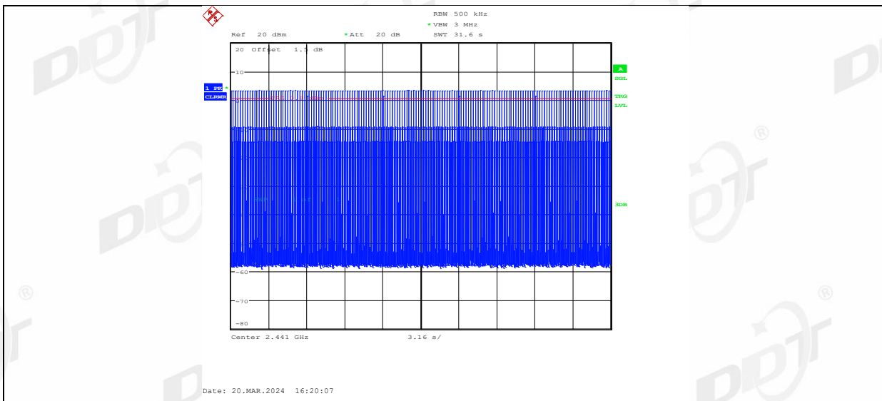
2DH5_Ant1_Hop
