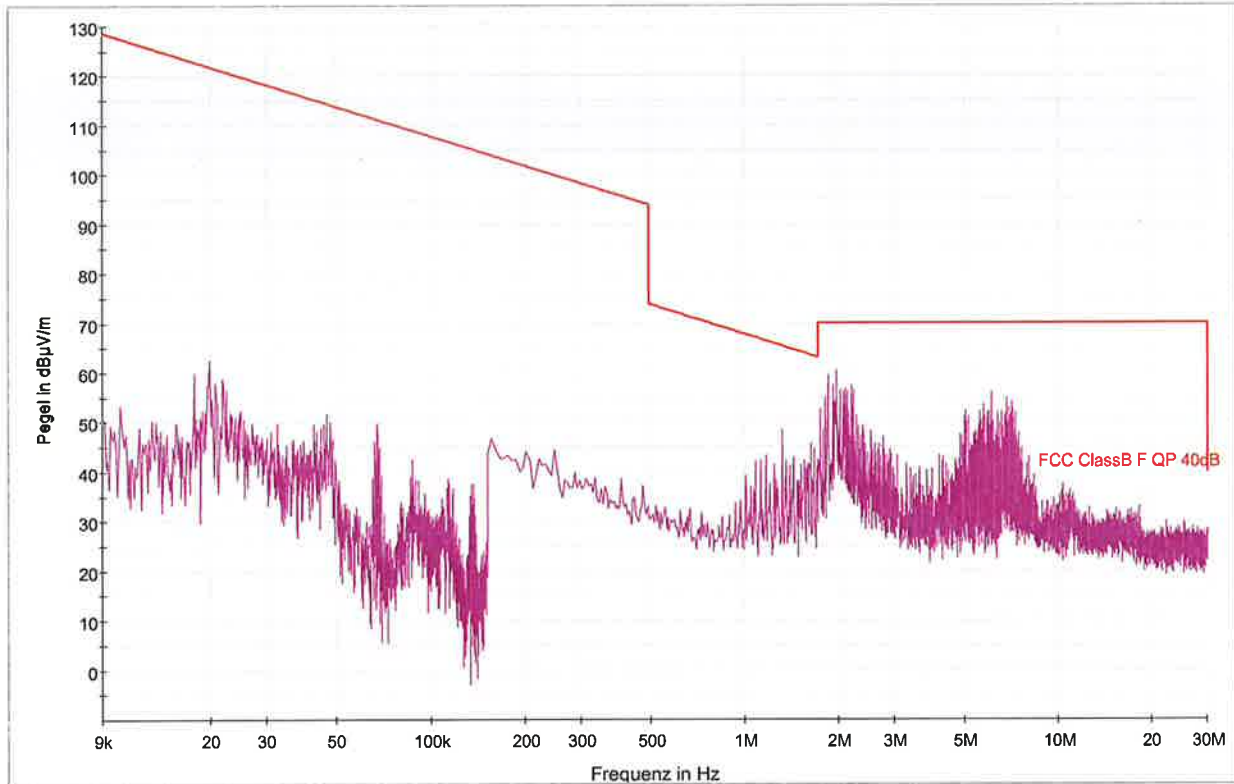
— FCC ClassB F QP 40dB — PK+_CLRWR@Naim F0
