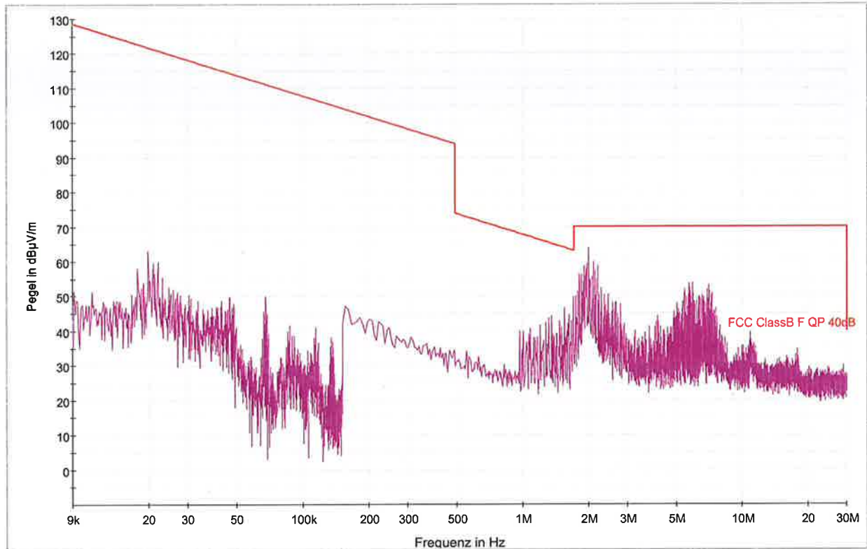
PK+_CLRWR@Naim F0 FCC ClassB F QP 40dB
