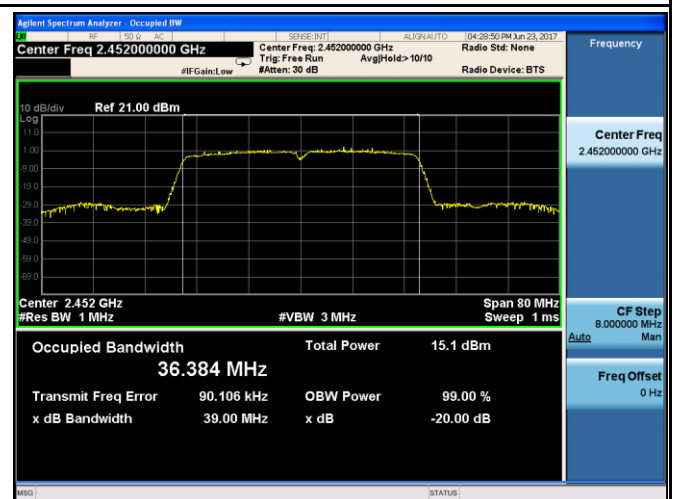
802.11n40 20dB Bandwidth - CH 9
