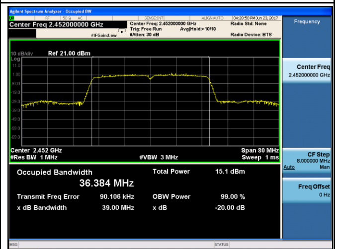
802.11n40 20dB Bandwidth - CH 11
