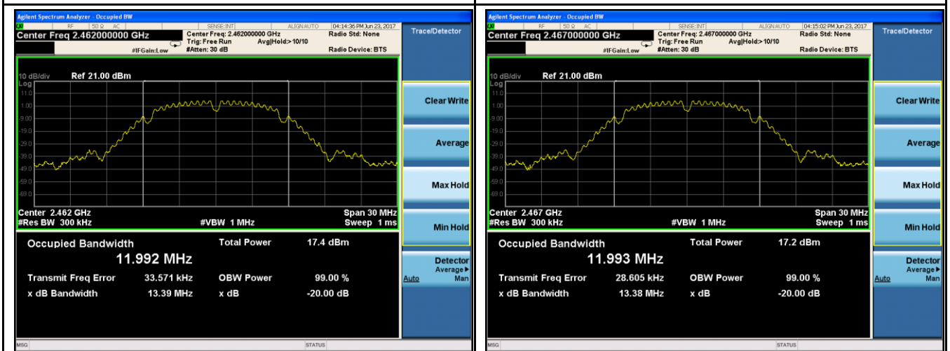
802.11b 20dB Bandwidth - CH 11
