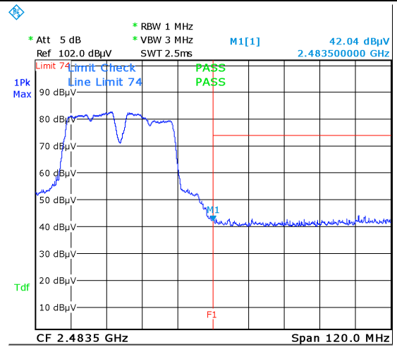
CH11 - 802.11n40 - PK
