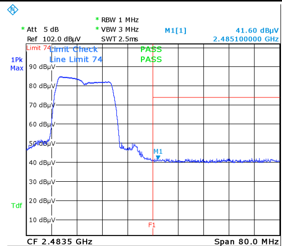
CH11 - 802.11g - PK
