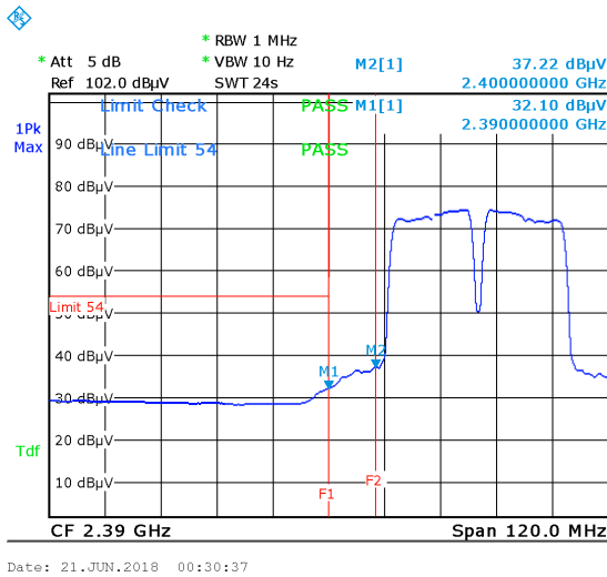
CH1 - 802.11n40 - AV
