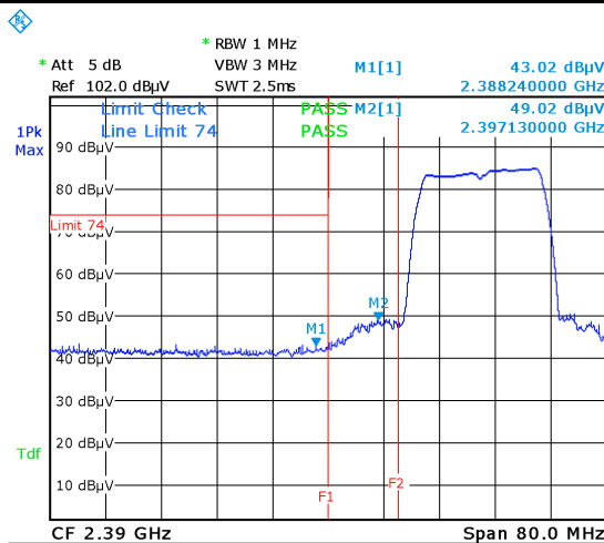
CH1 - 802.11g - PK
