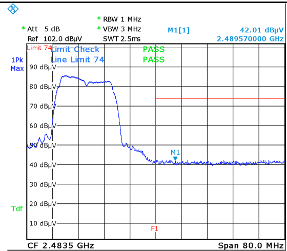
CH11 - 802.11b - PK
