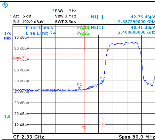
CH1 - 802.11b - PK
