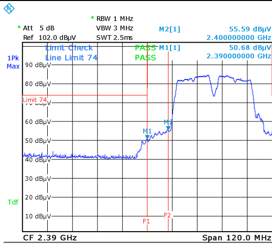
CH1 - 802.11n40 - PK
