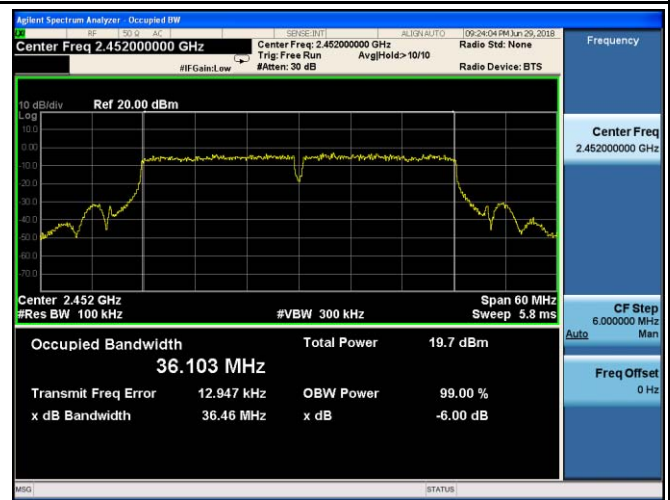
802.11n40 6dB Bandwidth - CH 9
