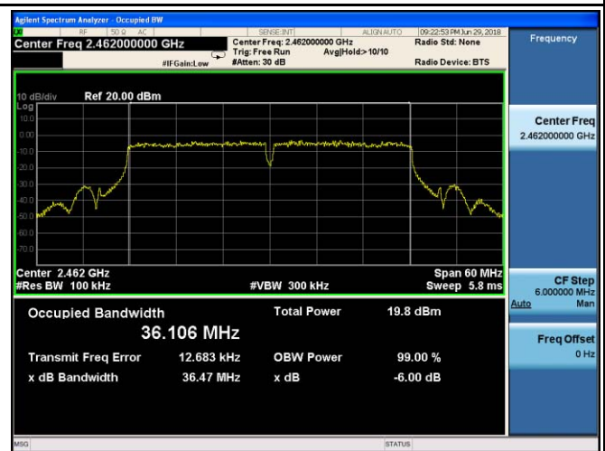
802.11n40 6dB Bandwidth - CH 11
