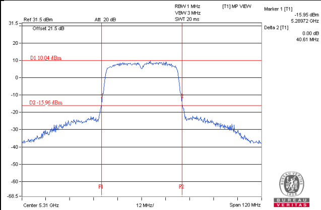
802.11ac (VHT80+80) / Chain 2 - CH58
