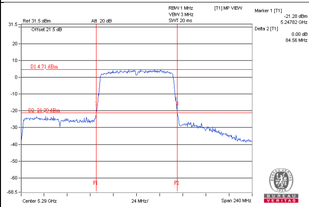
802.11ac (VHT80+80) / Chain 2 - CH58
