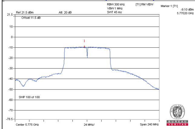
802.11ac (VHT80+80) / Chain 3– CH155(UNII-3 Band)
