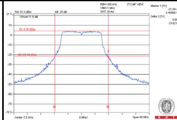
802.11ac (20MHz)
