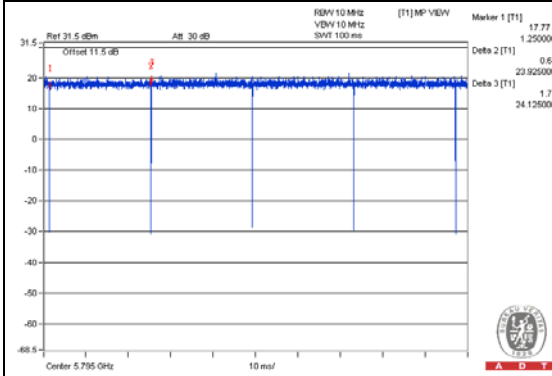
802.11ac (VHT40)_2TX
