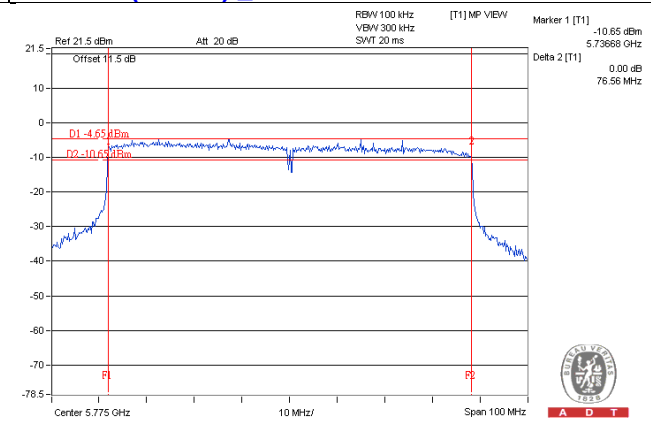
802.11ac (VHT80)_2TX
