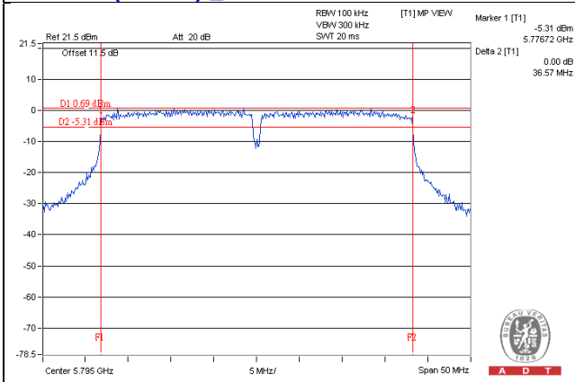
802.11ac (VHT40)_2TX
