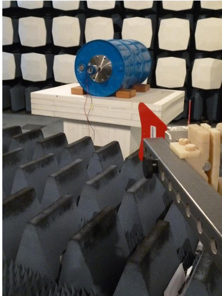
1-18GHz
