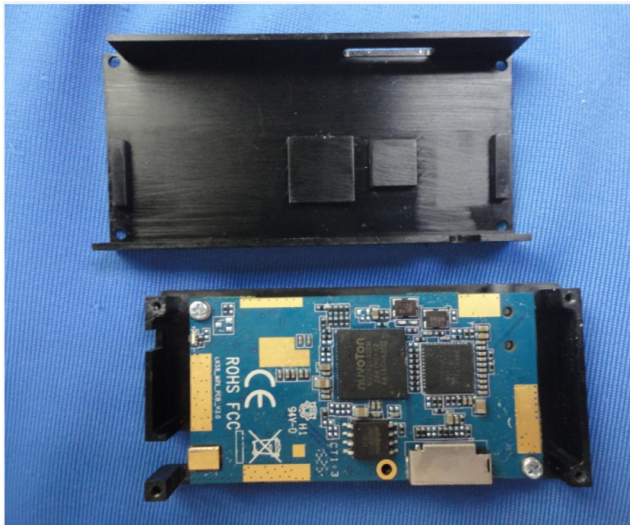
(3) EUT Photo
