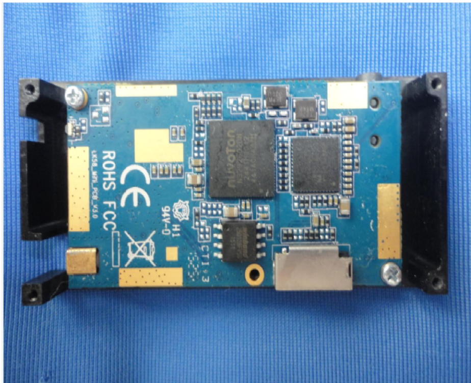
(4) EUT Photo
