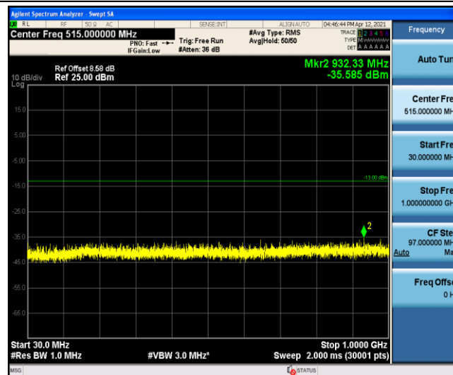
Band5-3MHz-QPSK-20415-1-0-Low-30-1000--35.59-PASS
