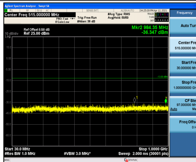
Band5-1.4MHz-QPSK-20525-1-0-Low-30-1000--36.35-PASS
