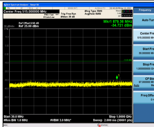
Band4-10MHz-QPSK-20000-1-0-Low-30-1000
