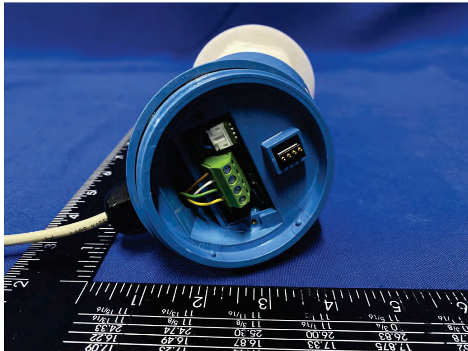
(2) EUT Photo
