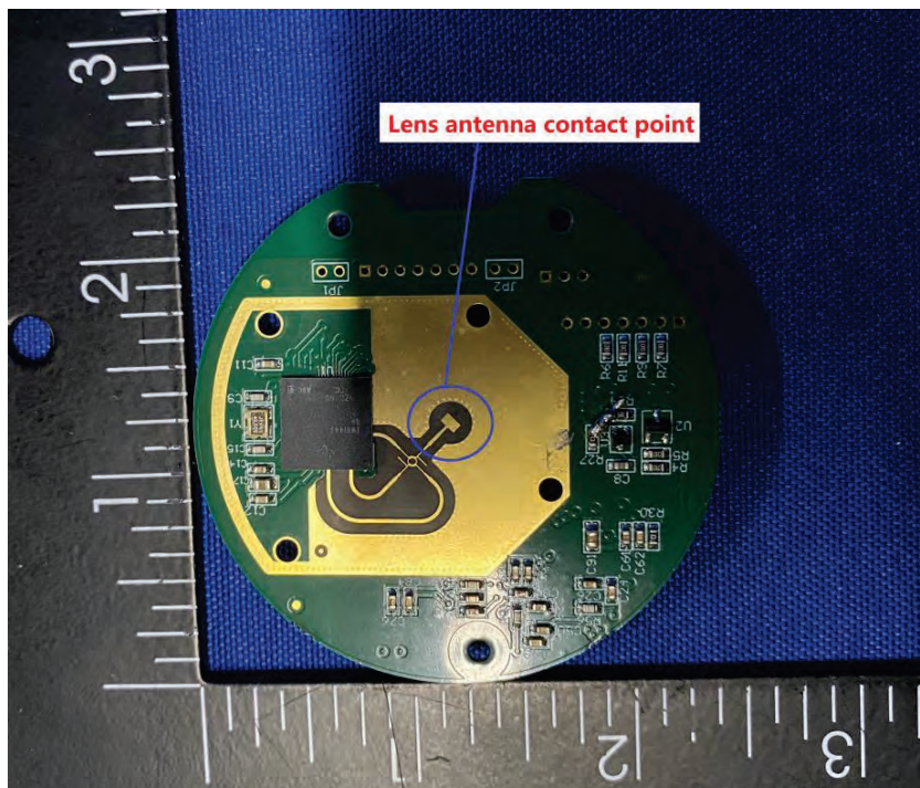
(14) EUT Photo
