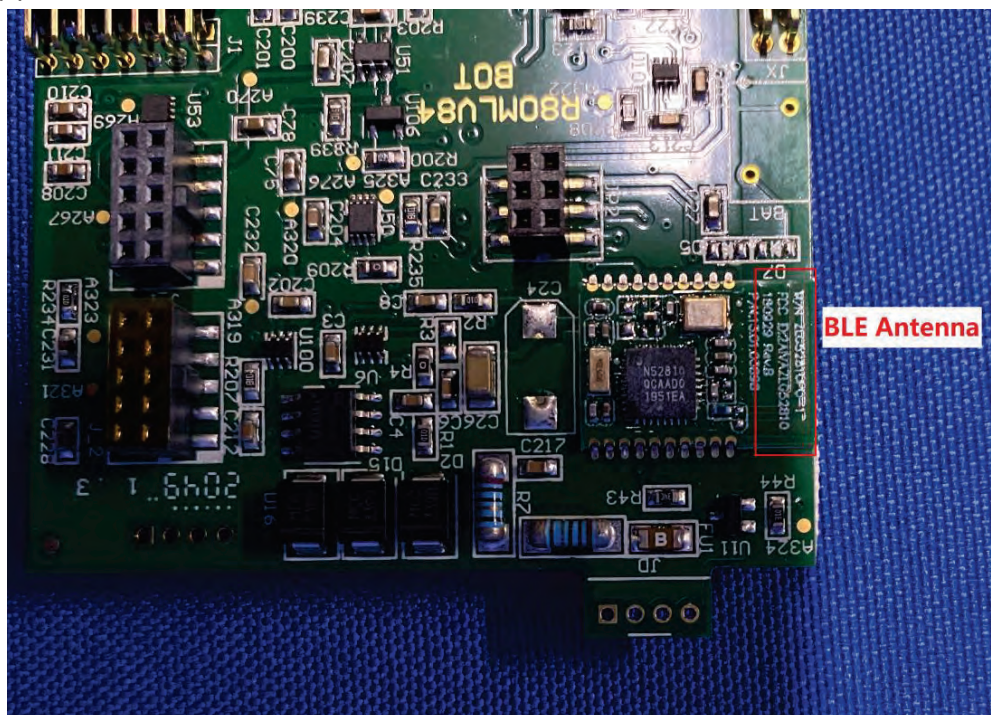
(6) EUT Photo
