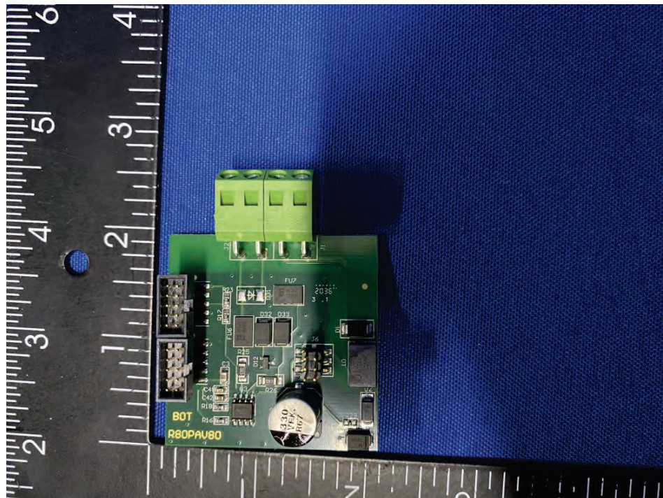
(8) EUT Photo
