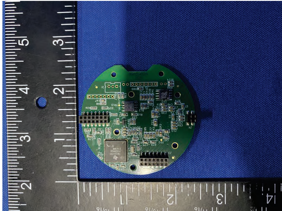
(14) EUT Photo
